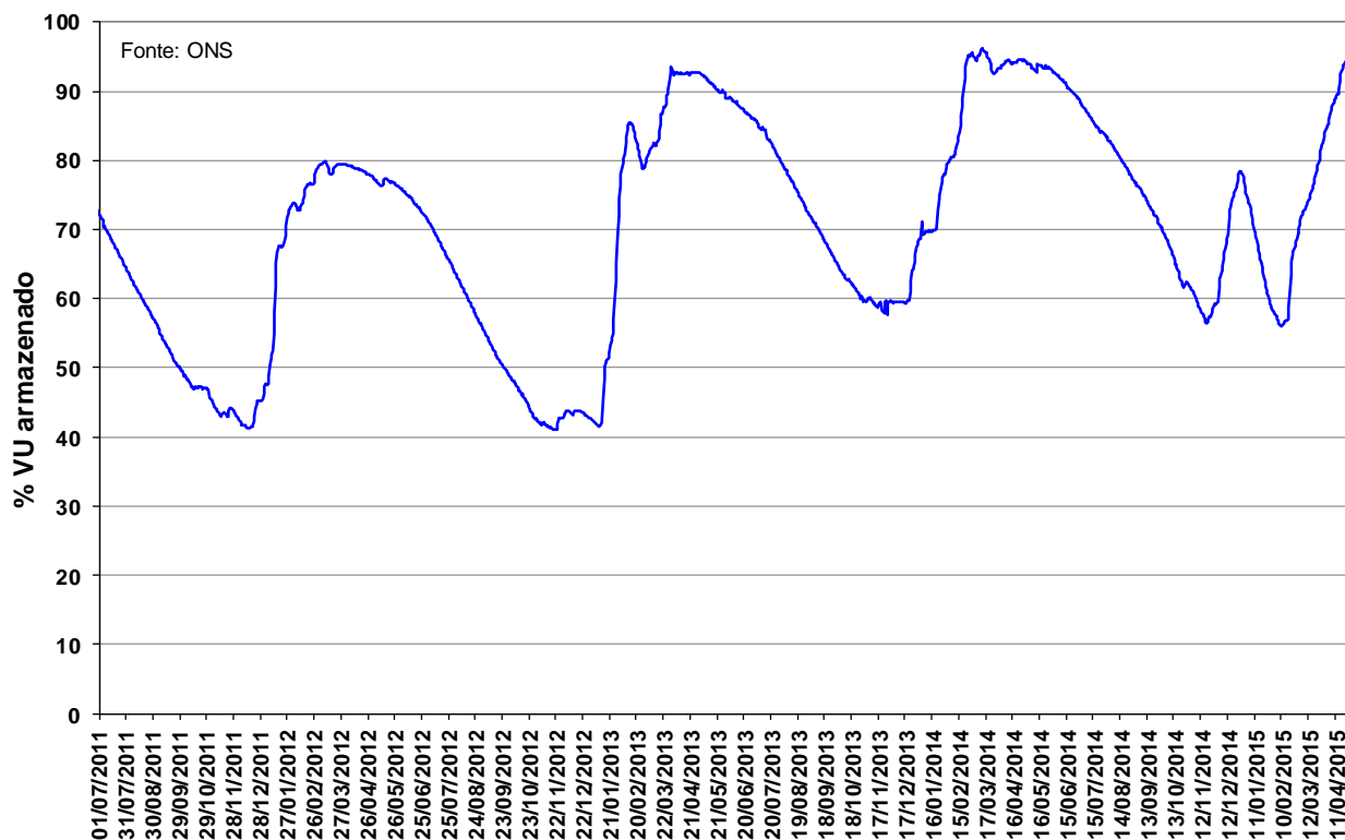
Figura 13 – Volume Útil armazenado na UHE Manso de julho de 2011 a abril de 2015.
