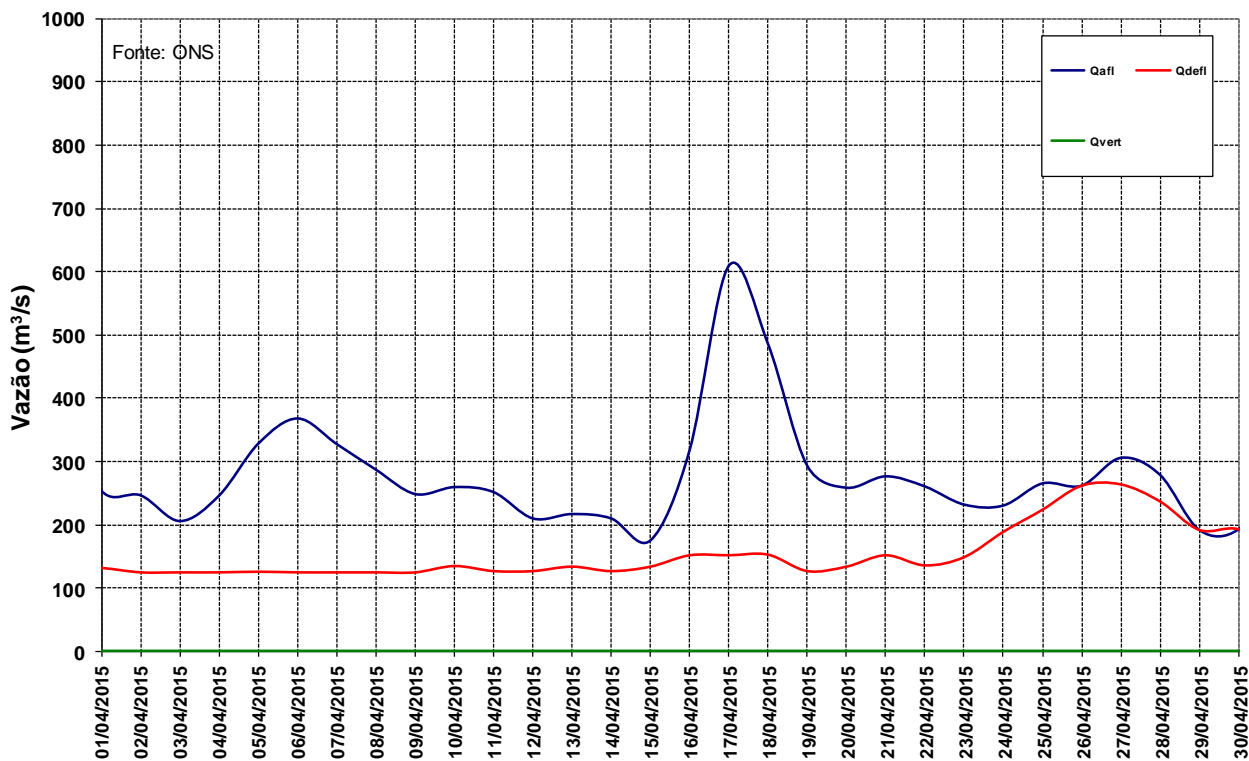
Figura 12 – Vazões na UHE Manso para o mês de abril de 2015.
