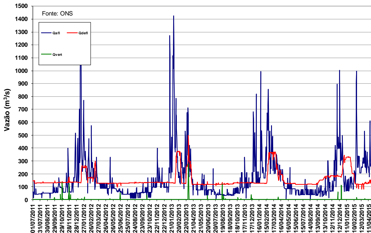
Figura 11 – Vazões na UHE Manso de julho de 2011 a abril de 2015.
