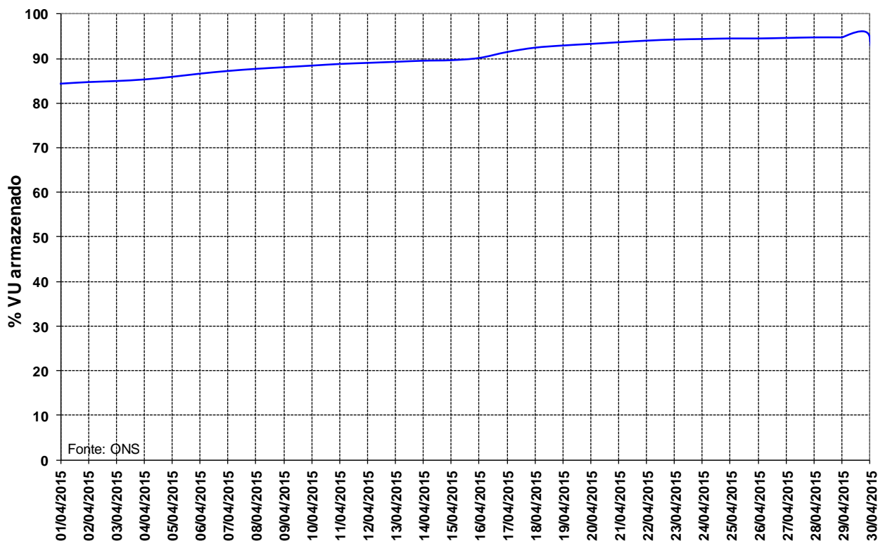
Figura 14 – Volume Útil armazenado na UHE Manso para o mês de abril de 2015.
