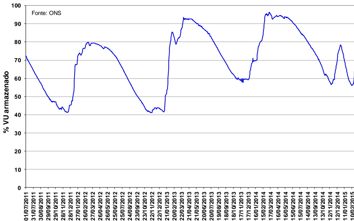
Figura 13 – Volume Útil armazenado na UHE Manso de julho de 2011 a fevereiro de 2015.
