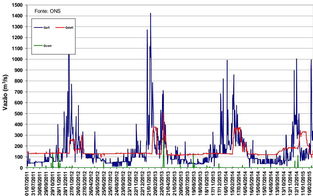
Fonte: ONS Figura 11 – Vazões na UHE Manso de julho de 2011 a fevereiro de 2015.
