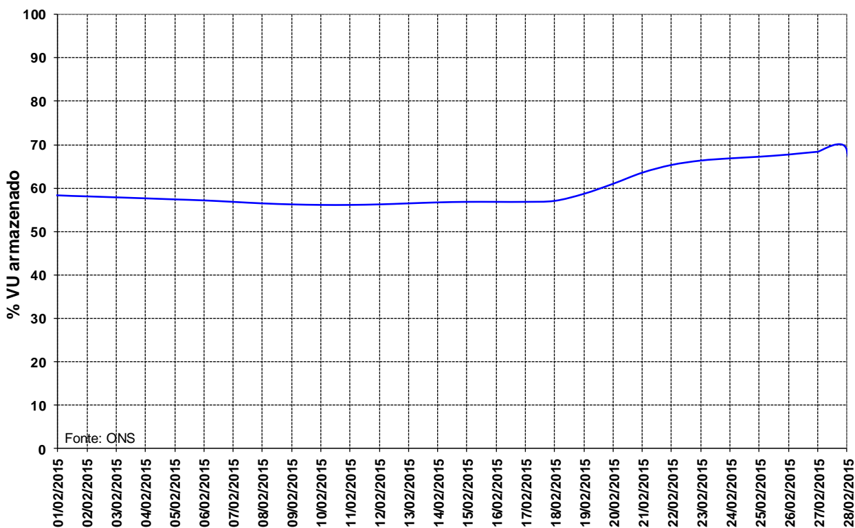
Figura 14 – Volume Útil armazenado na UHE Manso para o mês de fevereiro de 2015.
