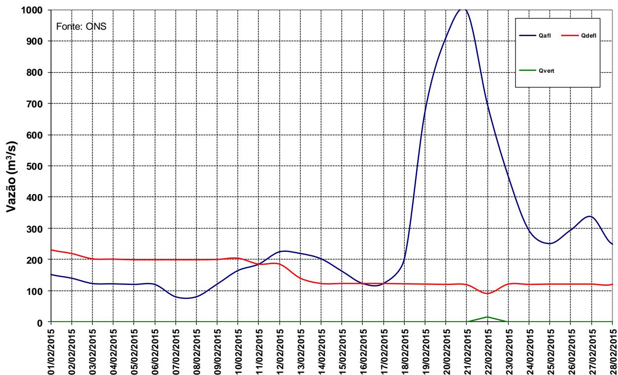
Fonte: ONS Figura 12 – Vazões na UHE Manso para o mês de fevereiro de 2015.
