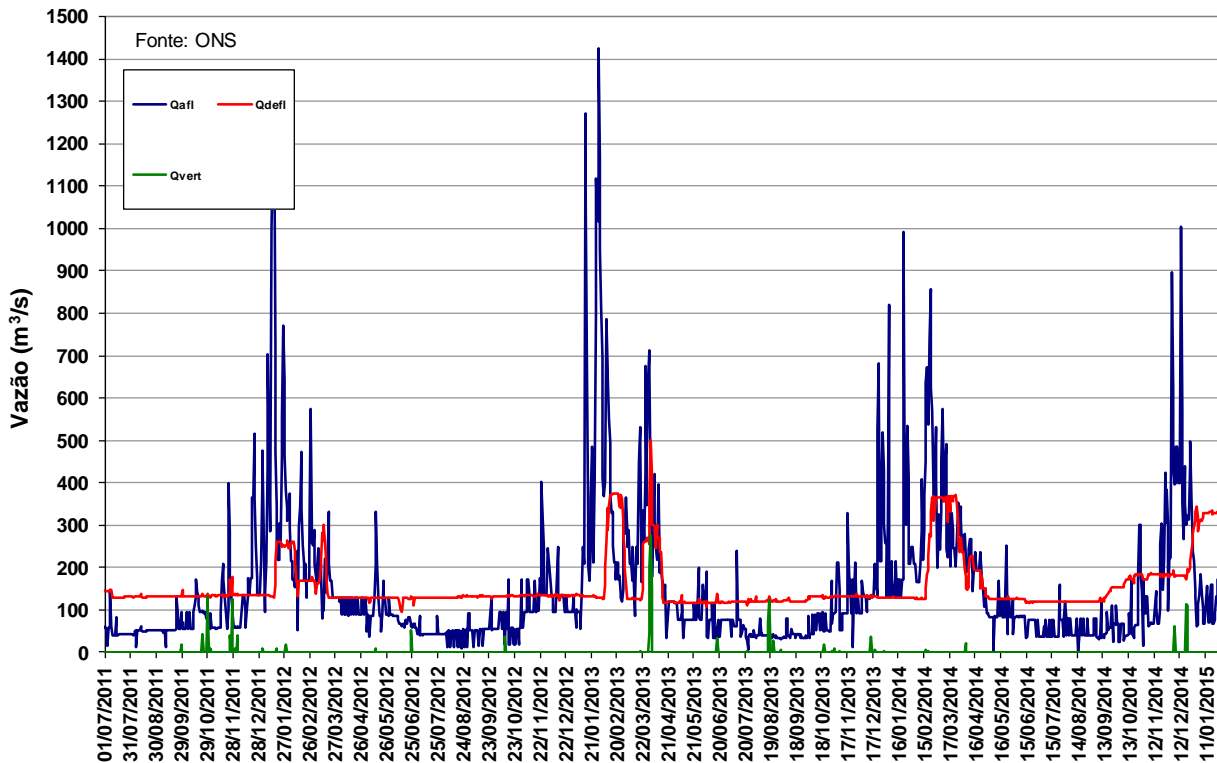
Figura 11 – Vazões na UHE Manso de julho de 2011 a janeiro de 2015.
