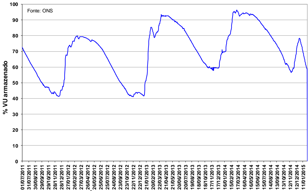
Figura 13 – Volume Útil armazenado na UHE Manso de julho de 2011 a janeiro de 2015.
