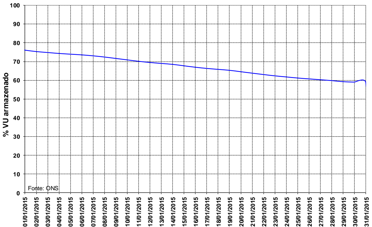
Figura 14 – Volume Útil armazenado na UHE Manso para o mês de janeiro de 2015.
