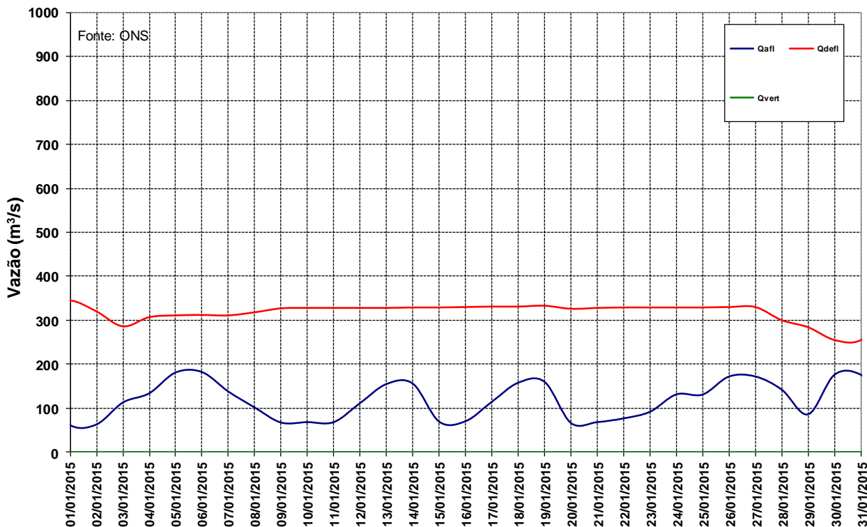
Figura 12 – Vazões na UHE Manso para o mês de janeiro de 2015.
