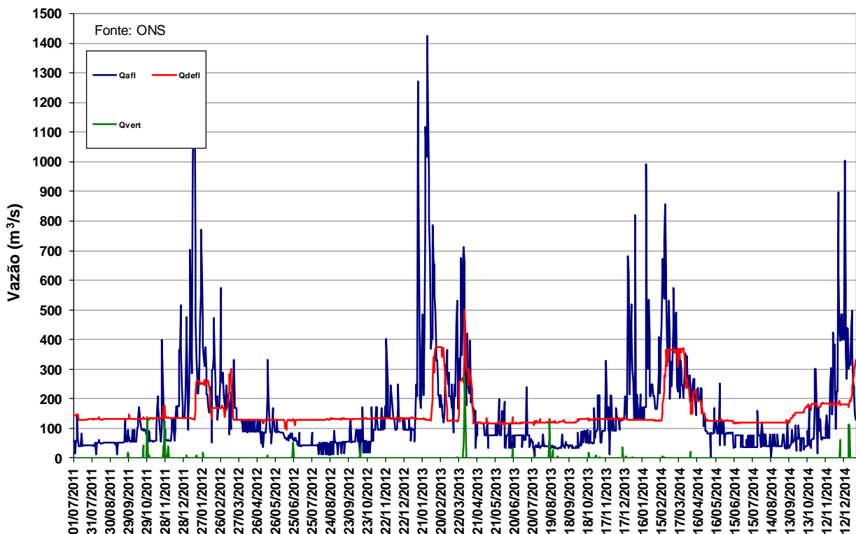
Figura 11 – Vazões na UHE Manso de julho de 2011 a dezembro de 2014.
