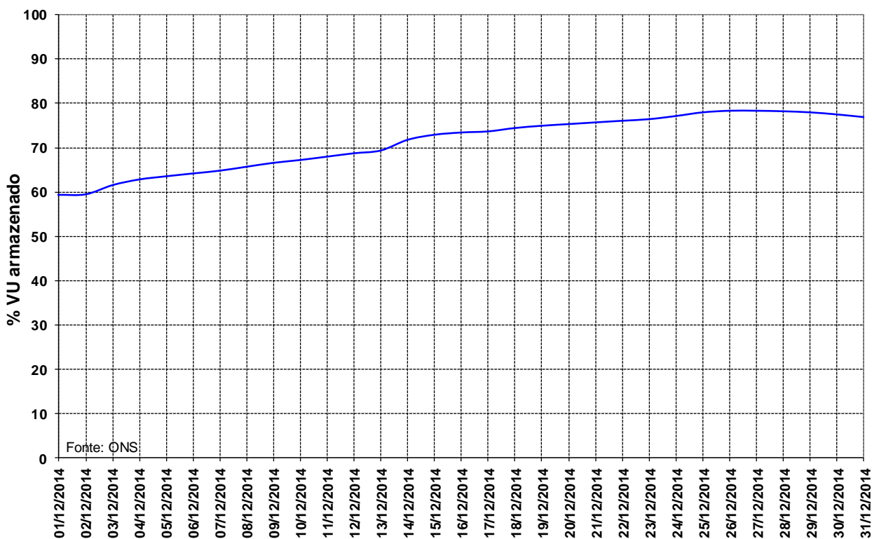
Figura 14 – Volume Útil armazenado na UHE Manso para o mês de dezembro de 2014.
