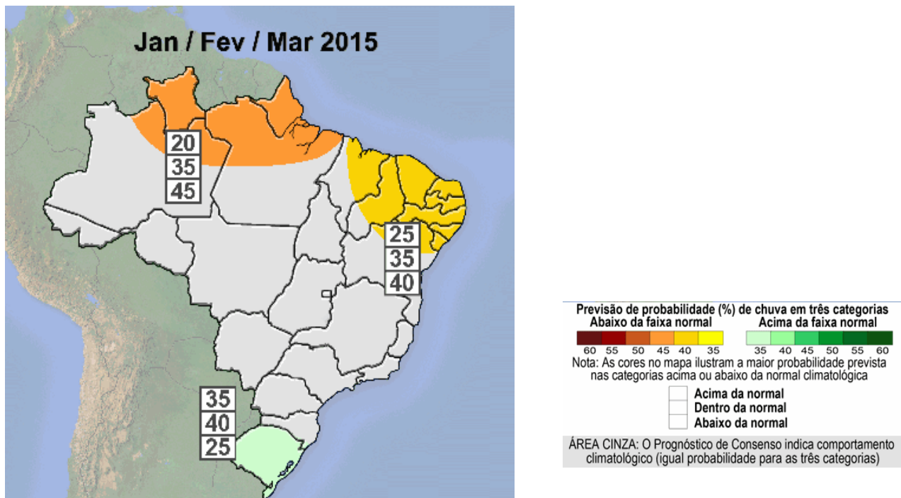
Figura 19 – Previsão climática para o trimestre jan/ fev /mar de 2015.
