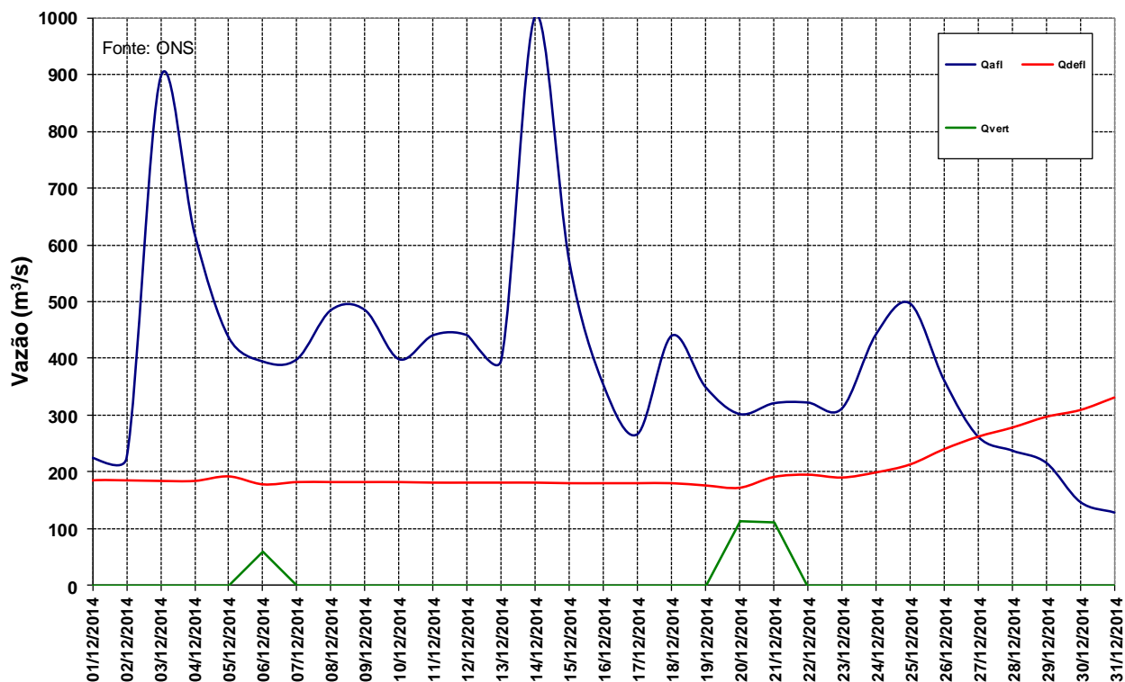
Figura 12 – Vazões na UHE Manso para o mês de dezembro de 2014.
