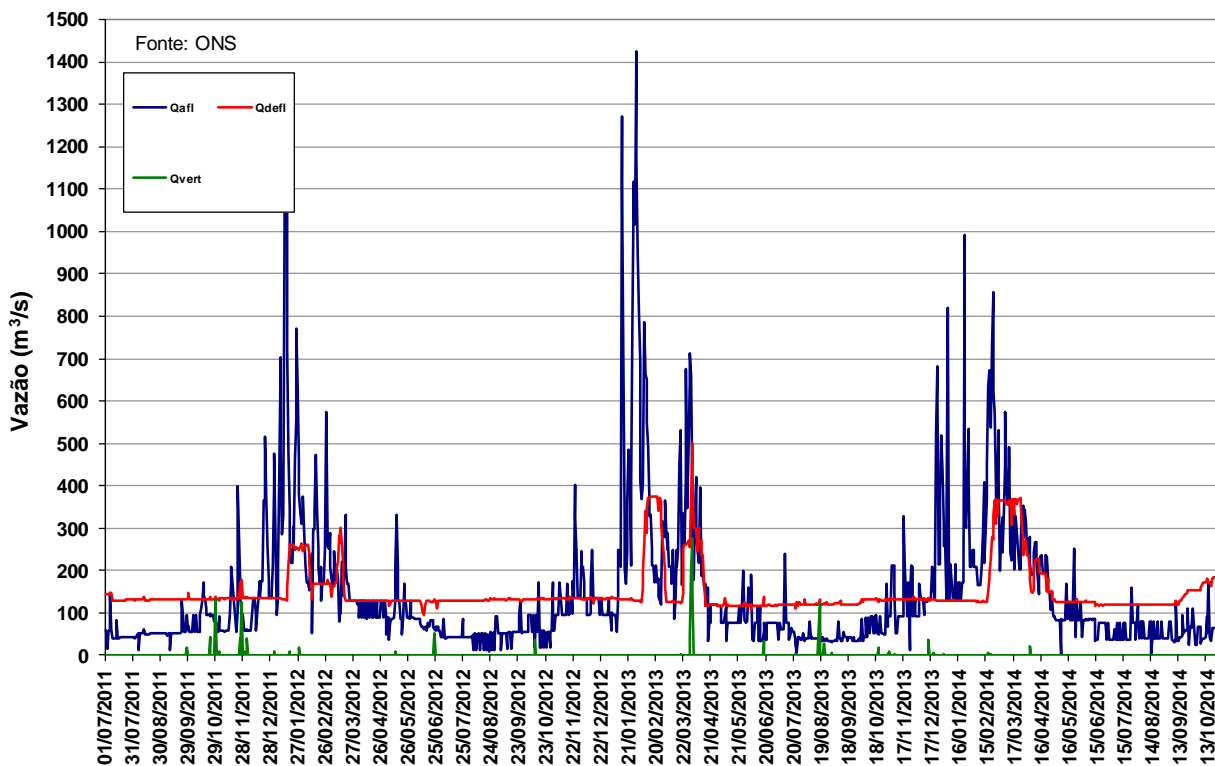
Fonte: ONS Figura 11 – Vazões na UHE Manso de julho de 2011 a outubro de 2014.
