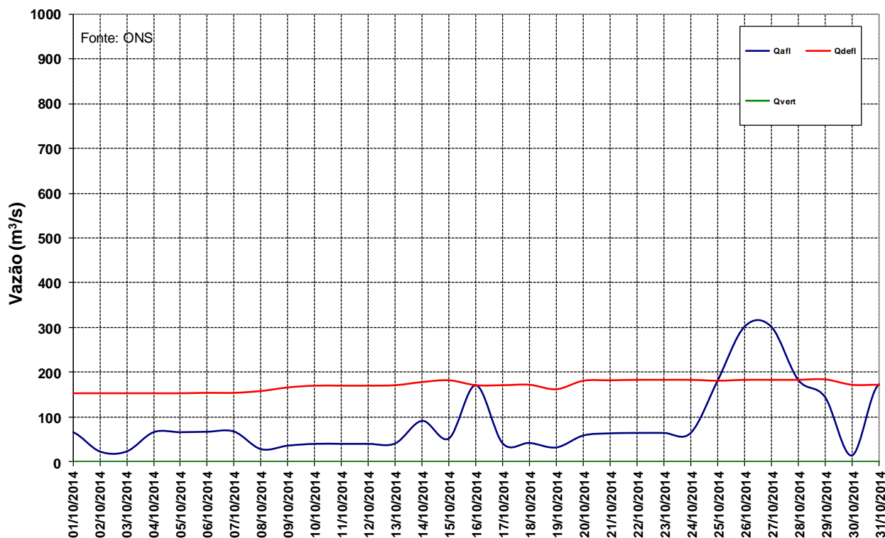
Fonte: ONS Figura 12 – Vazões na UHE Manso para o mês de outubro de 2014.
