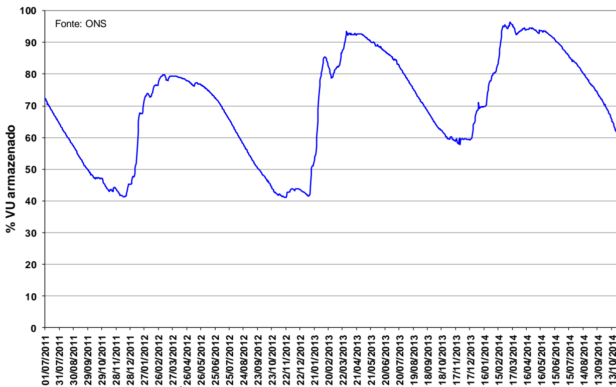
Figura 13 – Volume Útil armazenado na UHE Manso de julho de 2011 a outubro de 2014.
