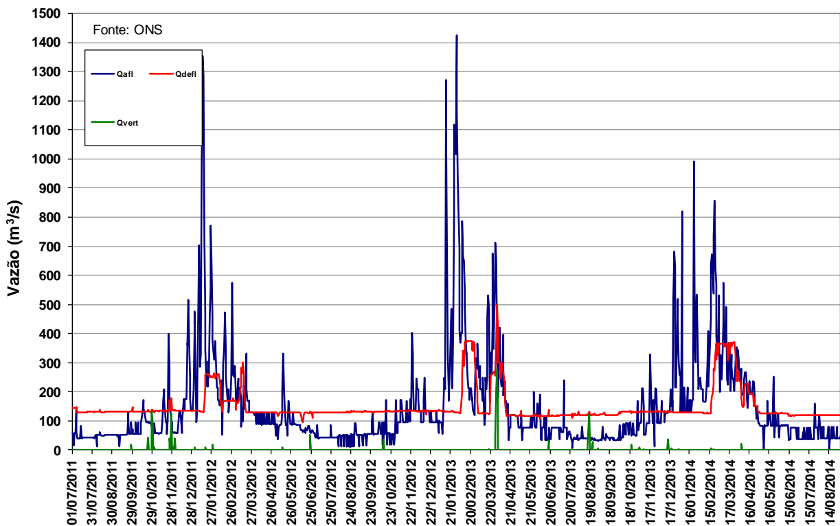
Figura 11 – Vazões na UHE Manso de julho de 2011 a agosto de 2014.
