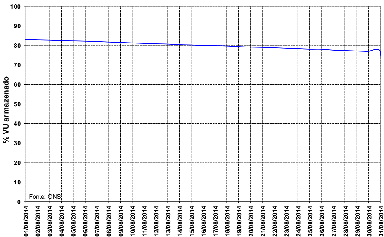
Figura 14 – Volume Útil armazenado na UHE Manso para o mês de agosto de 2014.
