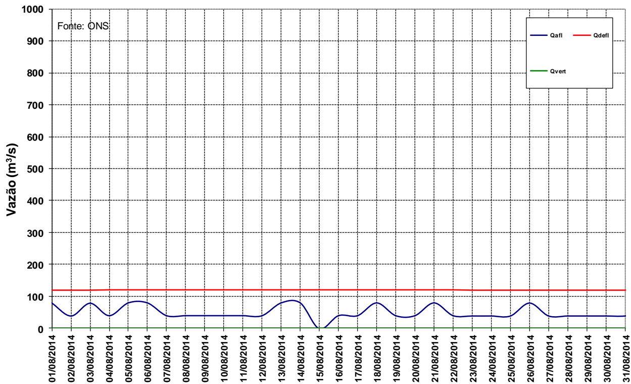
Figura 12 – Vazões na UHE Manso para o mês de agosto de 2014.
