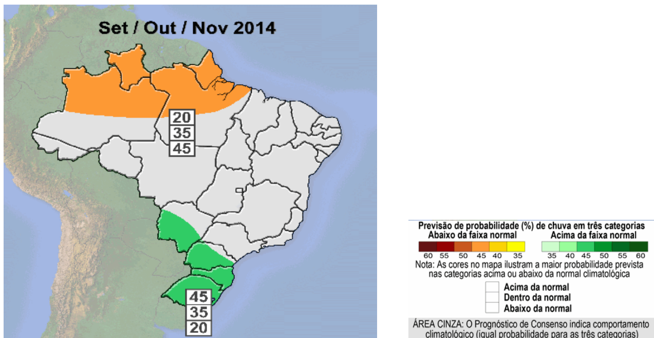
Figura 20 – Previsão climática para o trimestre set/ out /nov de 2014.
