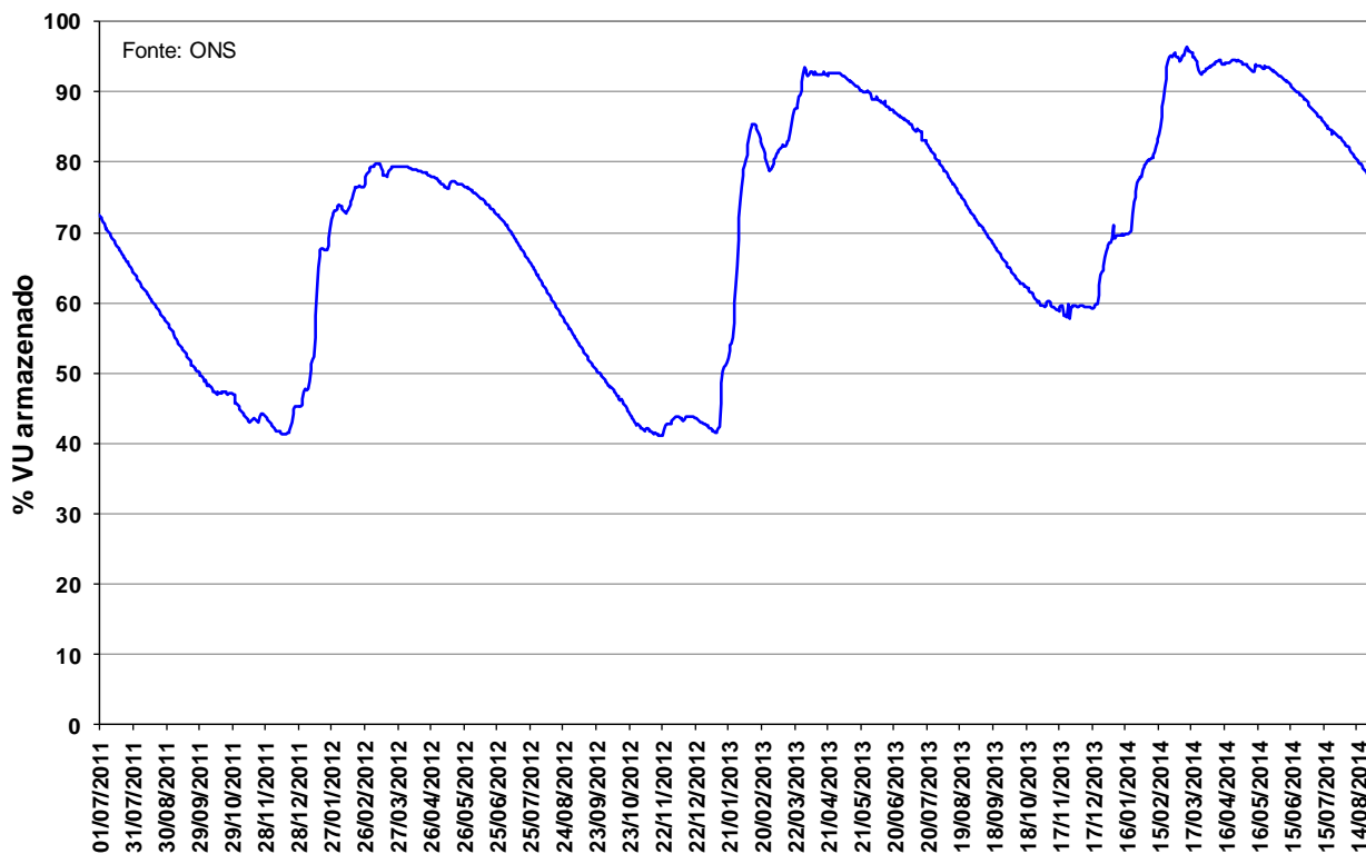
Figura 13 – Volume Útil armazenado na UHE Manso de julho de 2011 a agosto de 2014.
