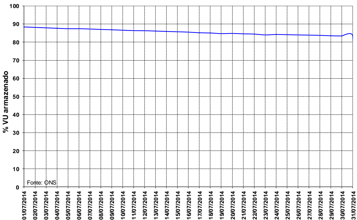
Figura 14 – Volume Útil armazenado na UHE Manso para o mês de julho de 2014.
