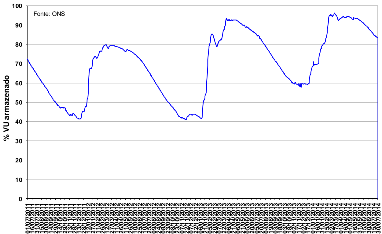
Figura 13 – Volume Útil armazenado na UHE Manso de julho de 2011 a julho de 2014.
