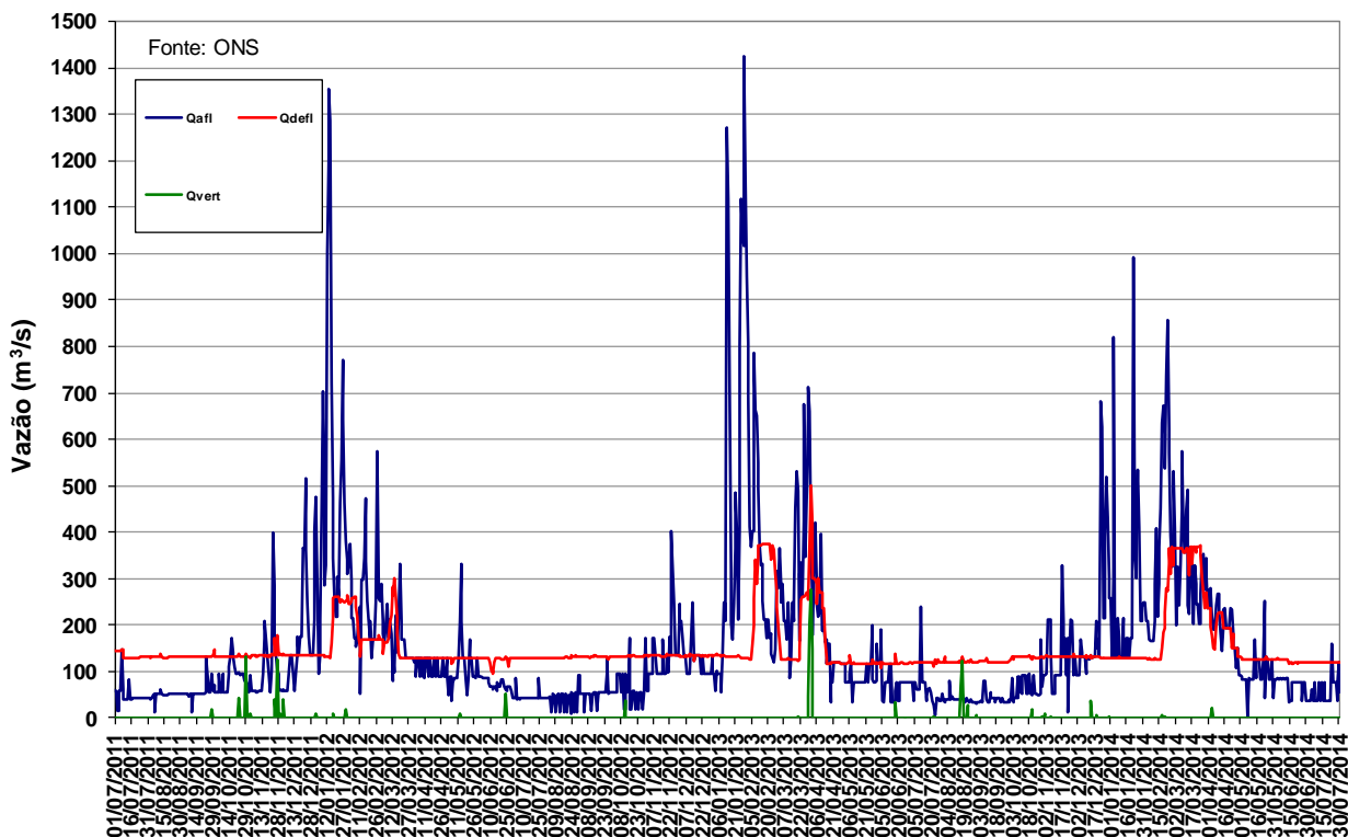
Figura 11 – Vazões na UHE Manso de julho de 2011 a julho de 2014.
