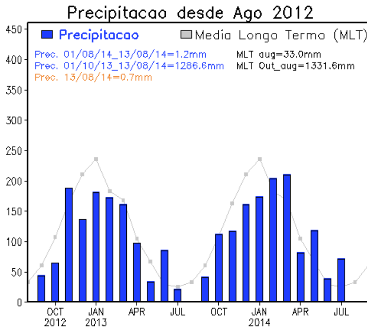
Figura 17 – Evolução da Precipitação Média na Bacia do Alto Paraguai.
