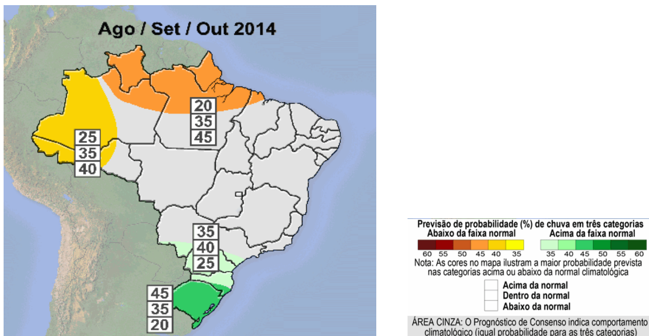
Figura 18 – Previsão climática para o trimestre ago/ set /out de 2014.
