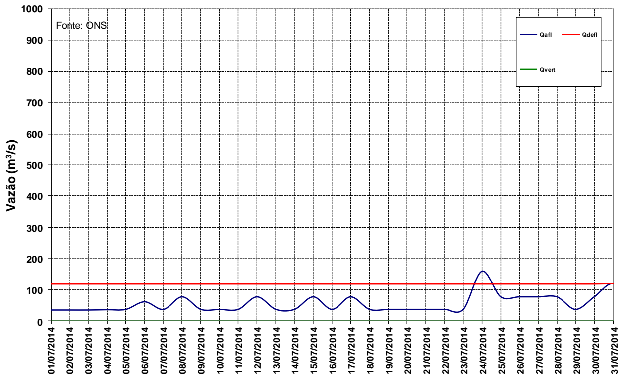
Figura 12 – Vazões na UHE Manso para o mês de julho de 2014.
