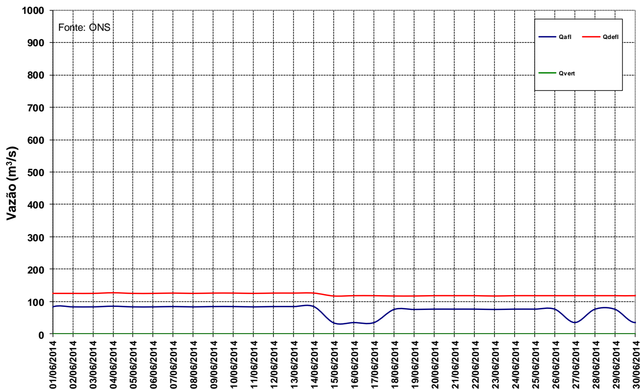
Figura 12 – Vazões na UHE Manso para o mês de junho de 2014.
