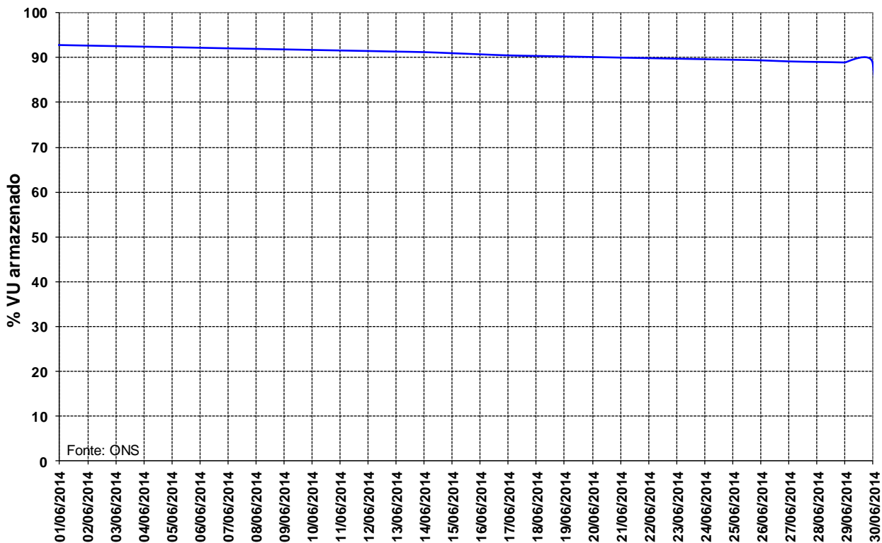
Figura 14 – Volume Útil armazenado na UHE Manso para o mês de junho de 2014.
