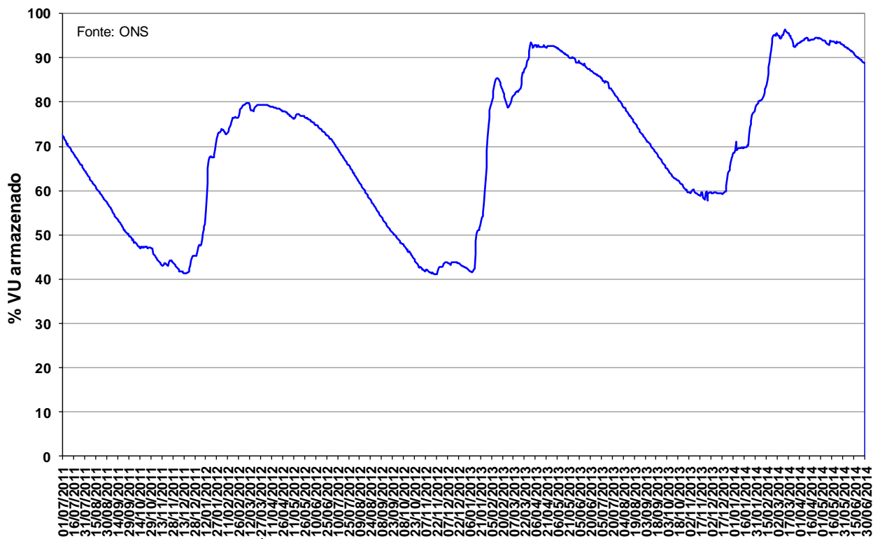
Figura 13 – Volume Útil armazenado na UHE Manso de julho de 2011 a junho de 2014.
