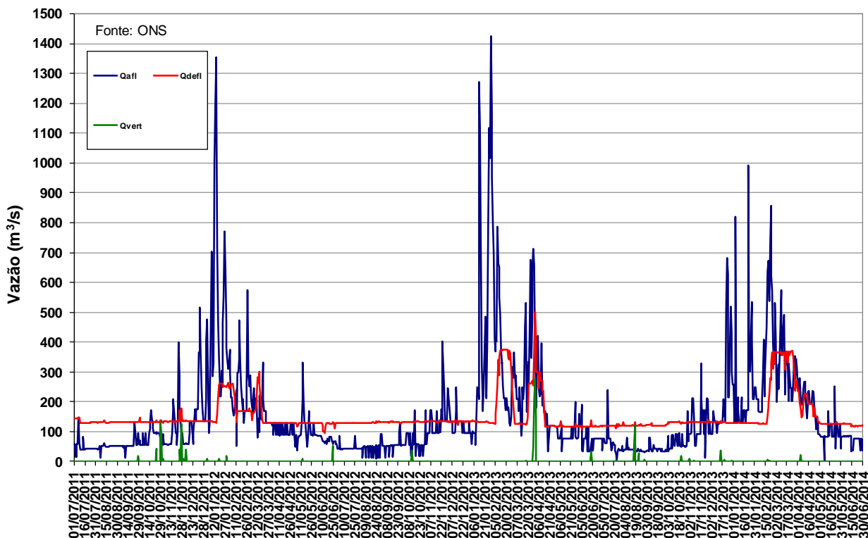
Figura 11 – Vazões na UHE Manso de julho de 2011 a junho de 2014.
