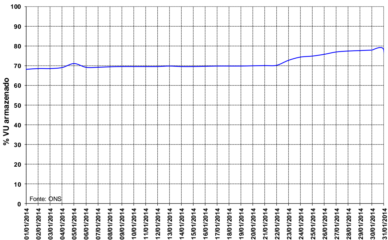
Figura 14 – Volume Útil armazenado na UHE Manso para o mês de janeiro de 2014.
