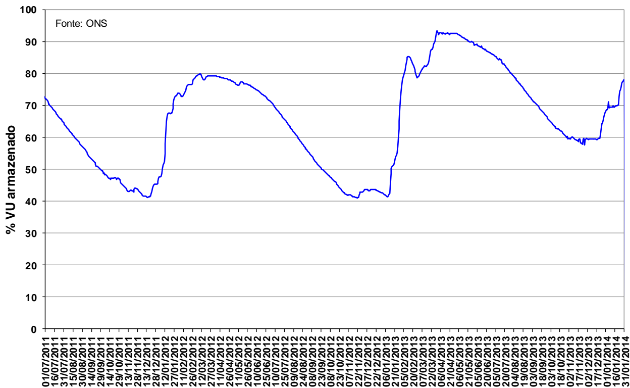
Figura 13 – Volume Útil armazenado na UHE Manso de julho de 2011 a janeiro de 2014.
