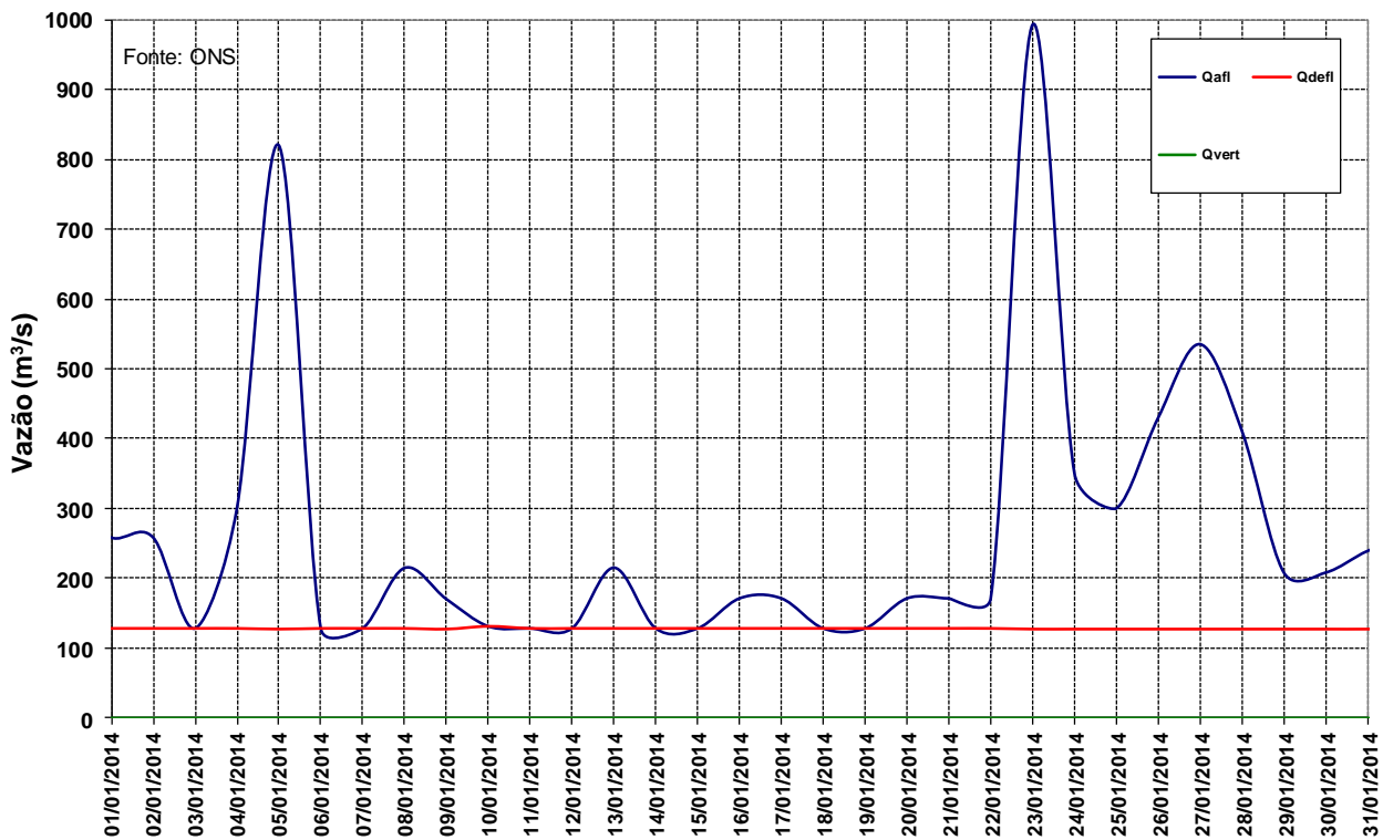
Figura 12 – Vazões na UHE Manso para o mês de janeiro de 2014.
