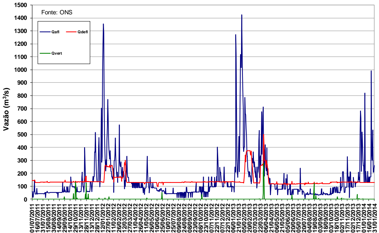
Figura 11 – Vazões na UHE Manso de julho de 2011 a janeiro de 2014.
