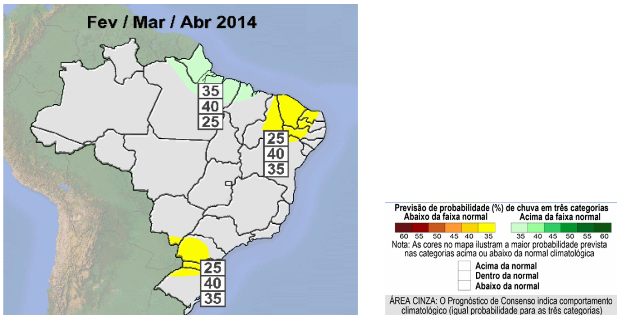
Figura 20 – Previsão climática para o trimestre fev/ mar /abr de 2014.
