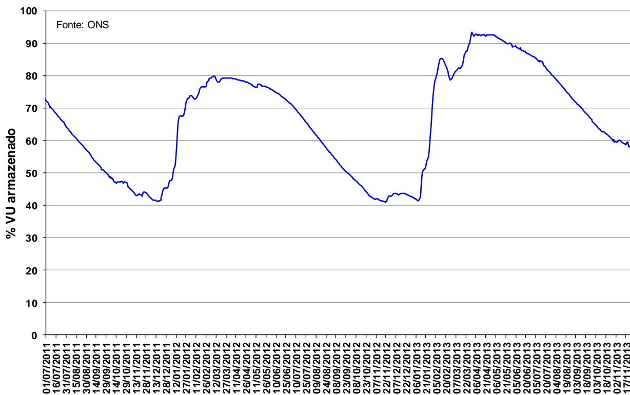
Figura 13 – Volume Útil armazenado na UHE Manso de julho de 2011 a novembro de 2013.
