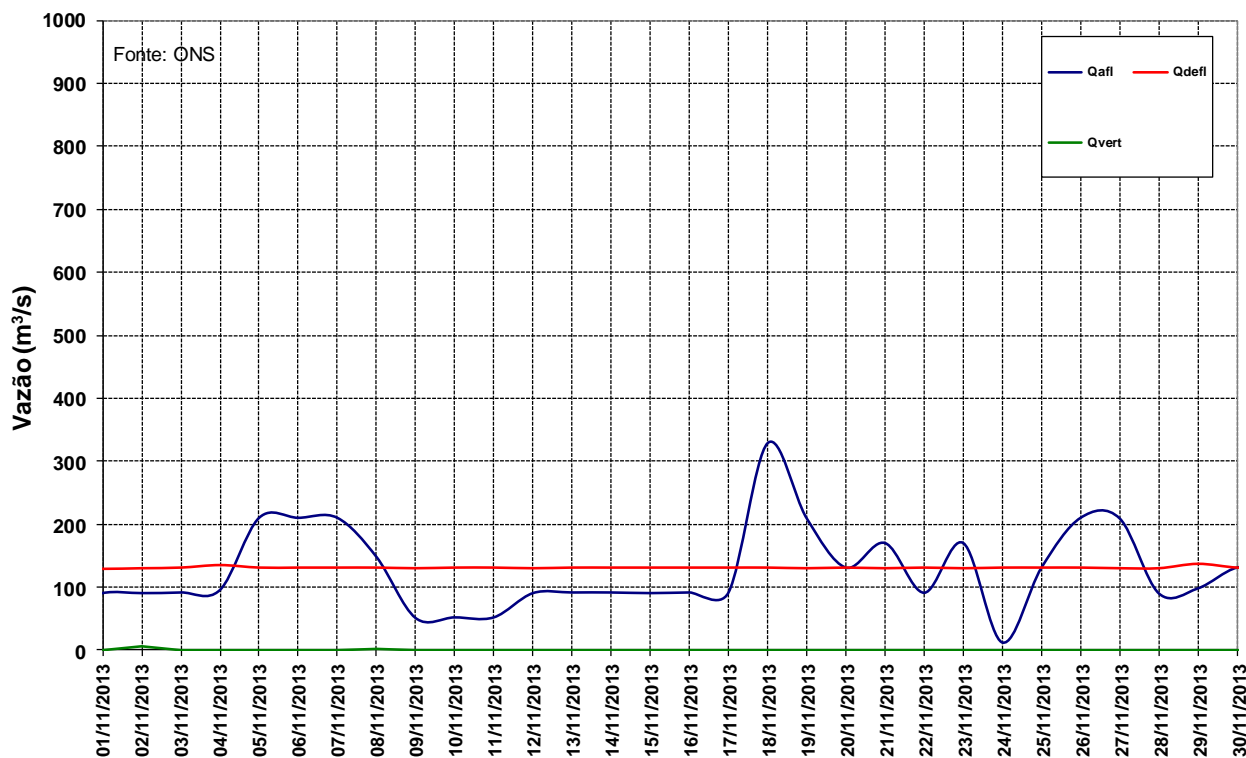
Figura 12 – Vazões na UHE Manso para o mês de novembro de 2013.
