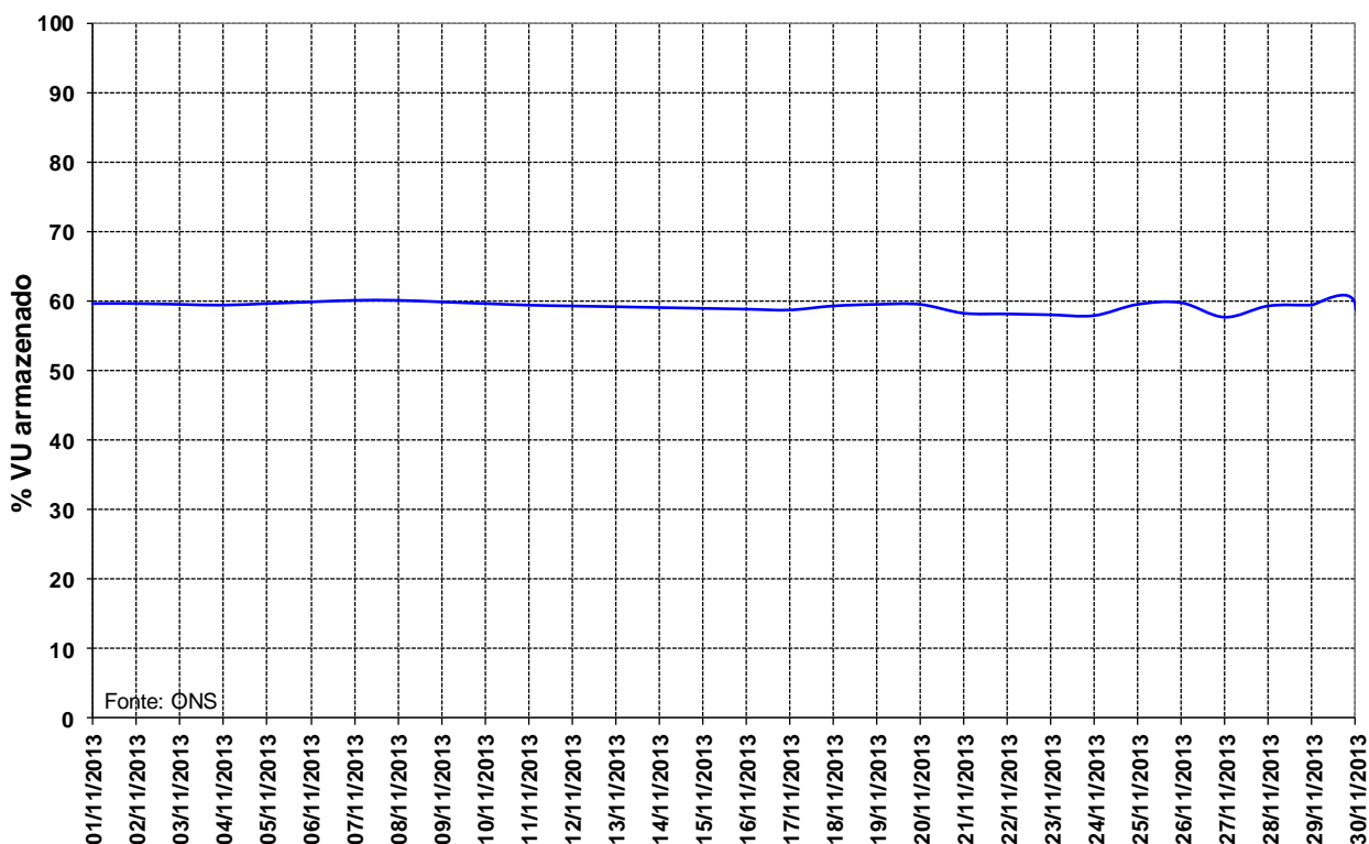
Figura 14 – Volume Útil armazenado na UHE Manso para o mês de novembro de 2013.
