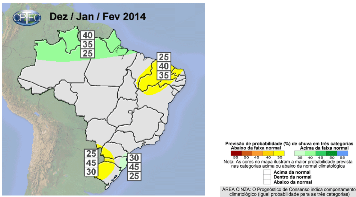
Figura 20 – Previsão climática para o trimestre dez 2013 / jan / fev de 2014.
