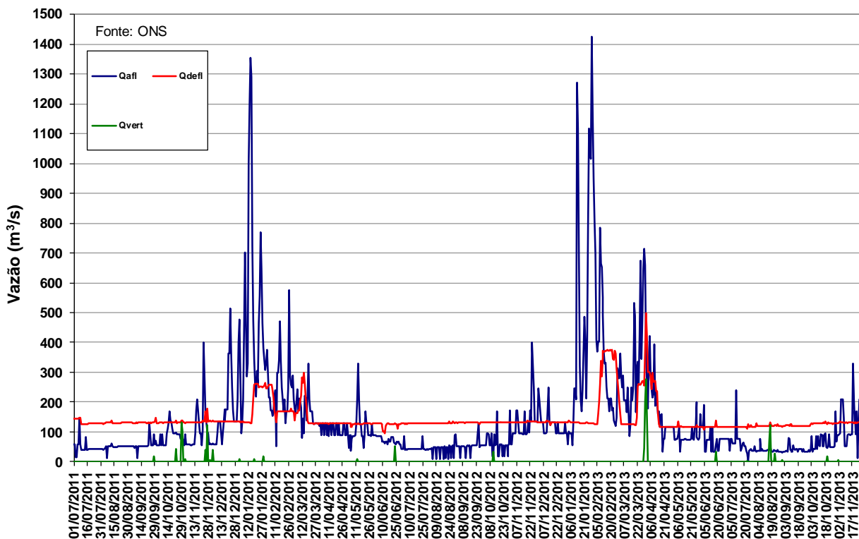
Figura 11 – Vazões na UHE Manso de julho de 2011 a novembro de 2013.
