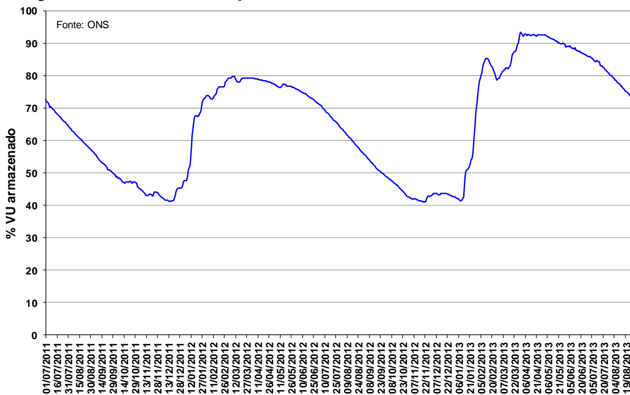
Figura 13 – Volume Útil armazenado na UHE Manso de julho de 2011 a agosto de 2013.
