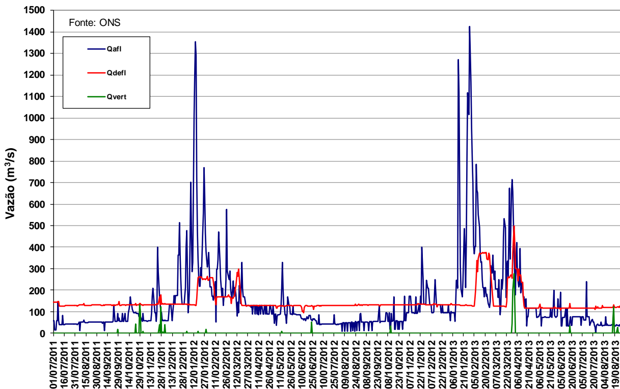
Figura 11 – Vazões na UHE Manso de julho de 2011 a agosto de 2013.
