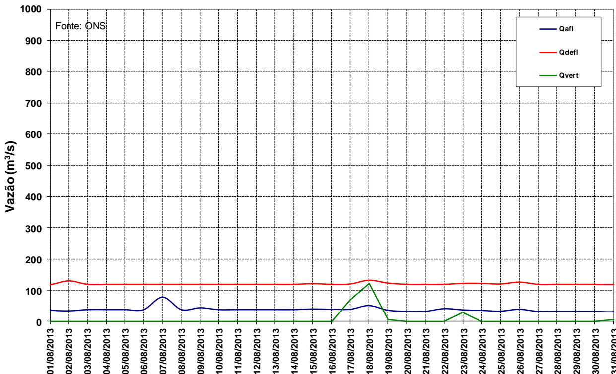
Figura 12 – Vazões na UHE Manso para o mês de agosto de 2013.
