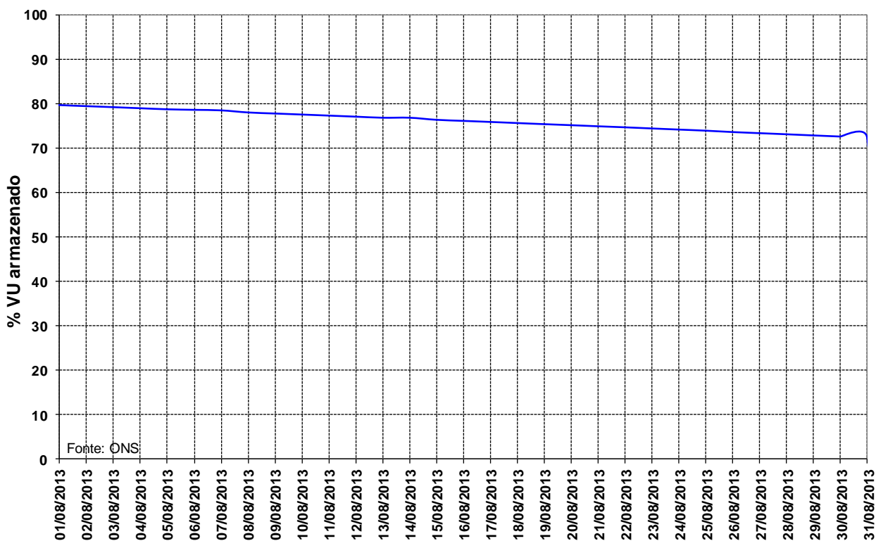
Figura 14 – Volume Útil armazenado na UHE Manso para o mês de agosto de 2013.
