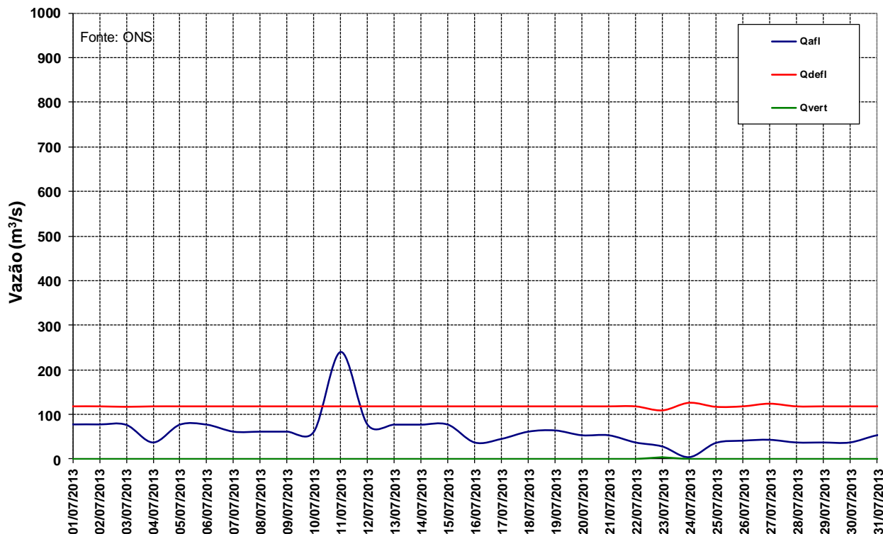
Figura 12 – Vazões na UHE Manso para o mês de julho de 2013.
