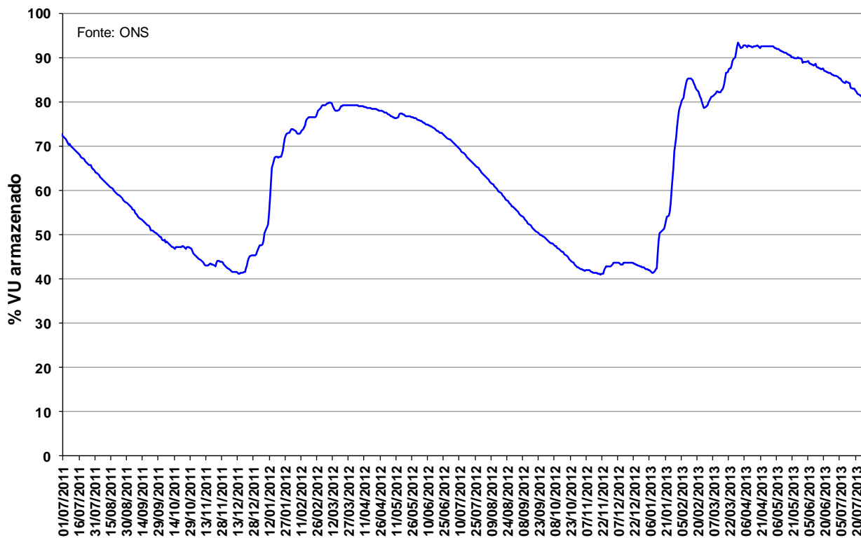
Figura 13 – Volume Útil armazenado na UHE Manso de julho de 2011 a julho de 2013.
