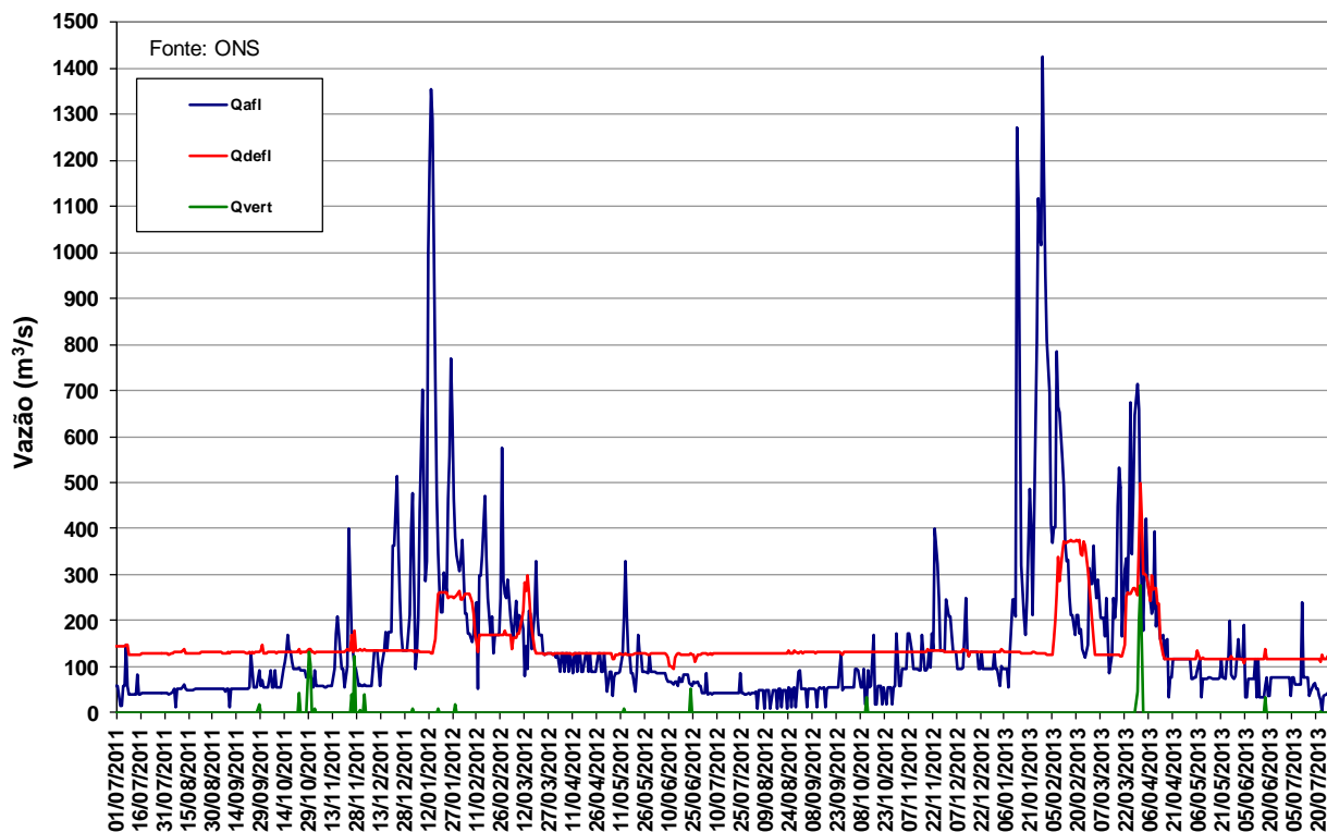
Figura 11 – Vazões na UHE Manso de julho de 2011 a julho de 2013.
