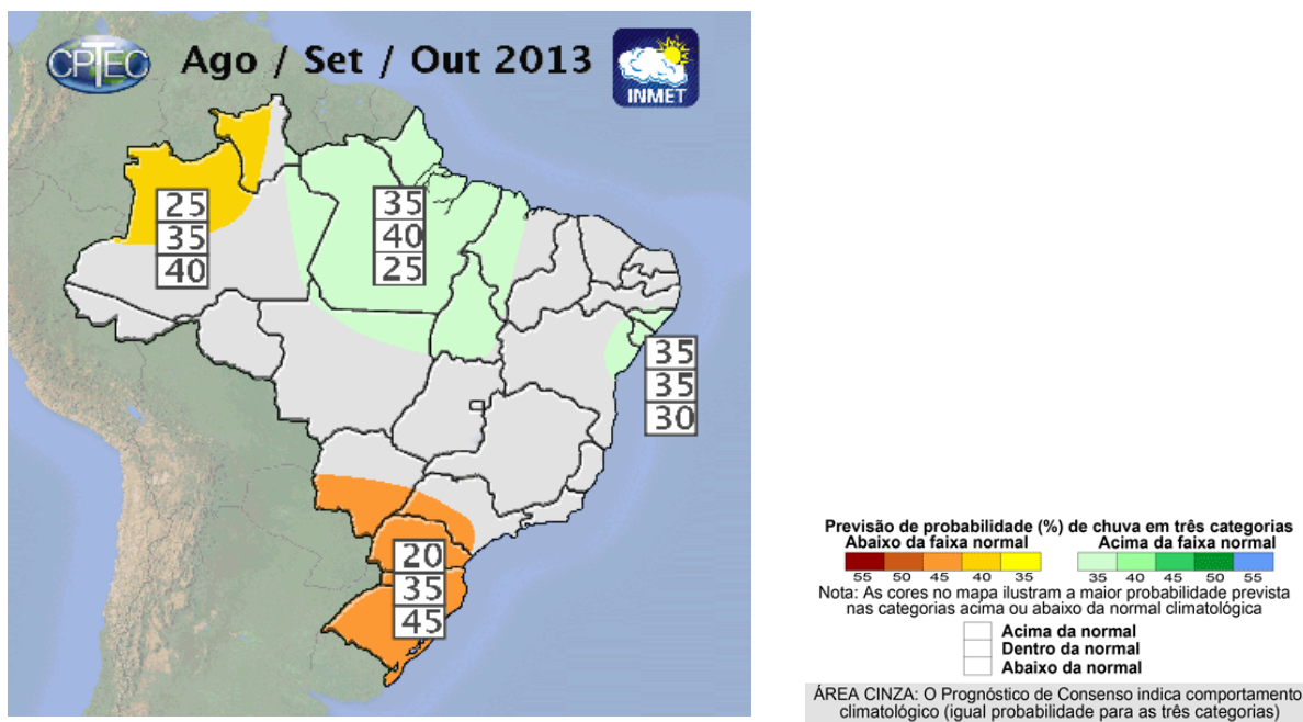
Figura 20 – Previsão climática para o trimestre ago / set / out de 2013.
