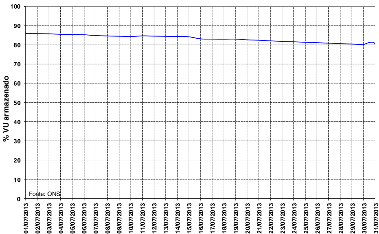
Figura 14 – Volume Útil armazenado na UHE Manso para o mês de julho de 2013.
