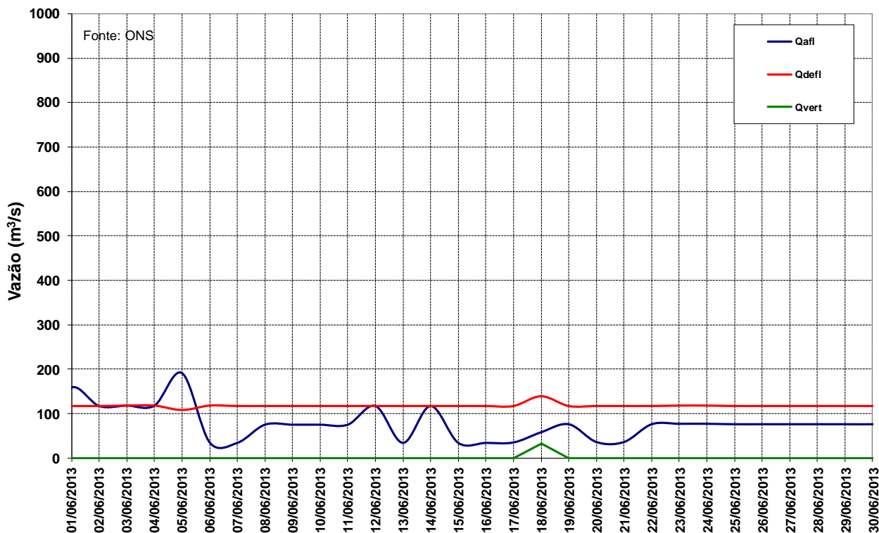
Figura 12 – Vazões na UHE Manso para o mês de junho de 2013.
