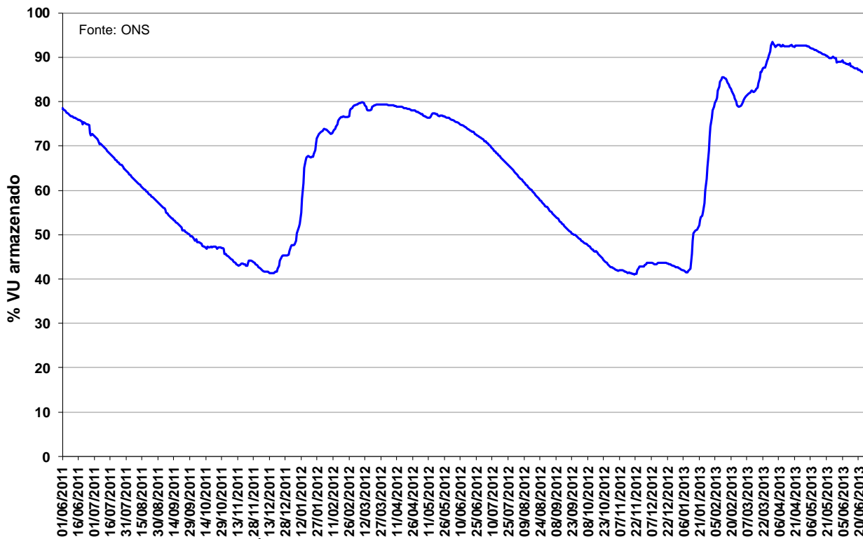
Figura 13 – Volume Útil armazenado na UHE Manso de junho de 2011 a junho de 2013.
