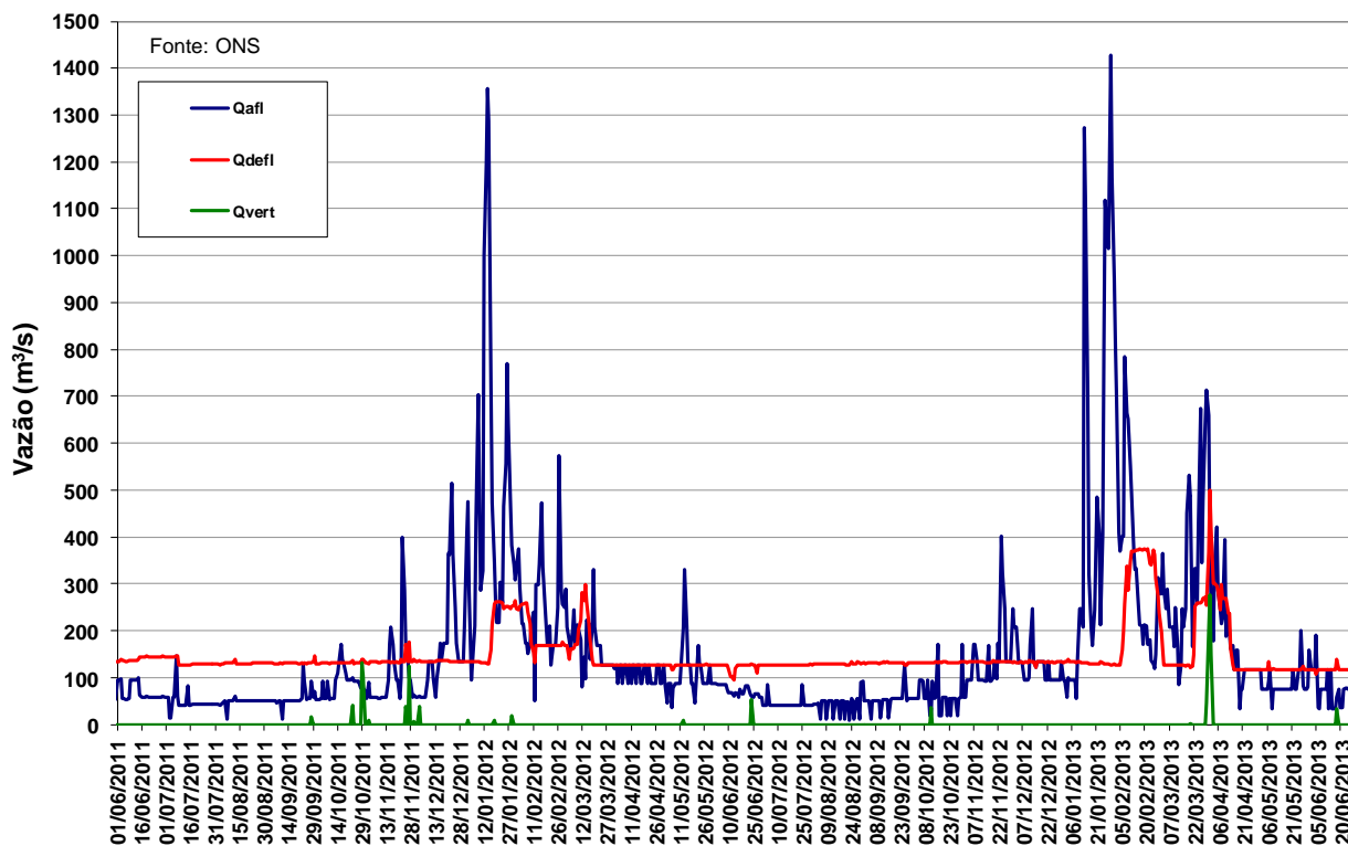
Figura 11 – Vazões na UHE Manso de junho de 2011 a junho de 2013.
