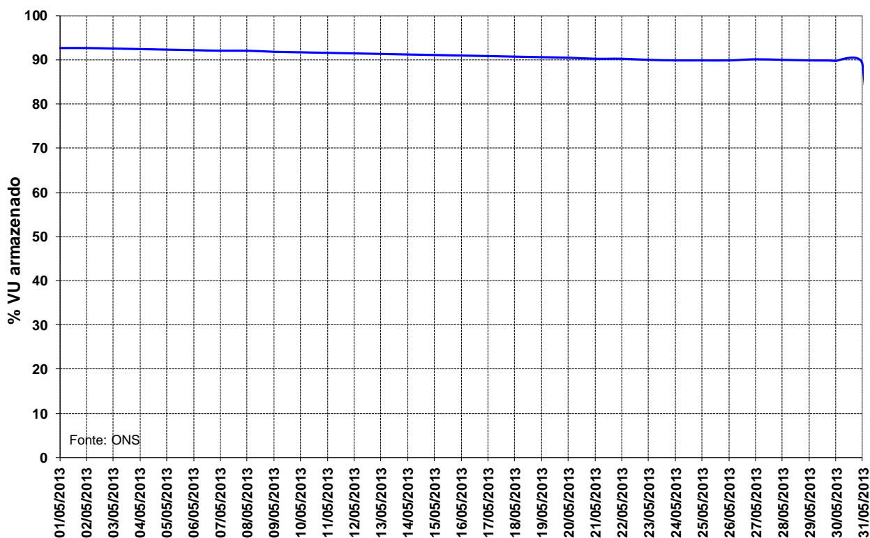
Figura 14 – Volume Útil armazenado na UHE Manso para o mês de maio de 2013.
