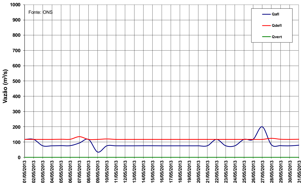
Figura 12 – Vazões na UHE Manso para o mês de maio de 2013.
