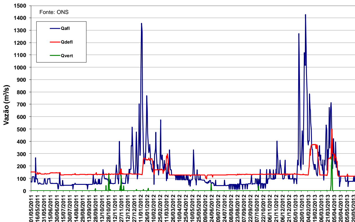
Figura 11 – Vazões na UHE Manso de maio de 2011 a maio de 2013.
