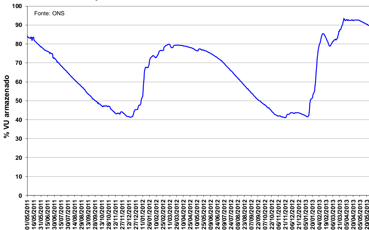
Figura 13 – Volume Útil armazenado na UHE Manso de maio de 2011 a maio de 2013.
