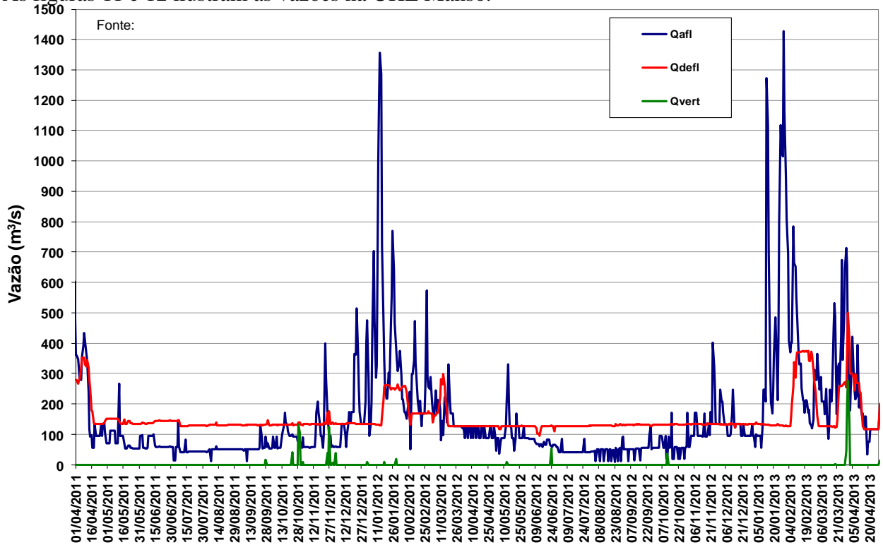
Figura 11 – Vazões na UHE Manso de abril de 2011 a abril de 2013.
