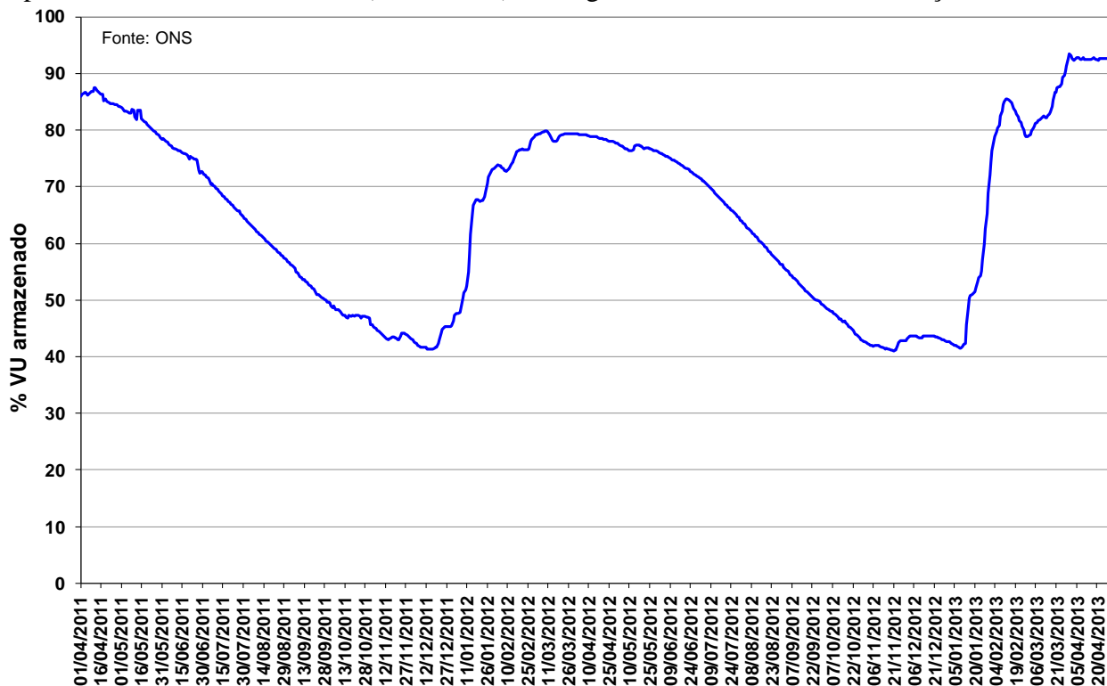
Figura 13 – Volume Útil armazenado na UHE Manso de abril de 2011 a abril de 2013.
