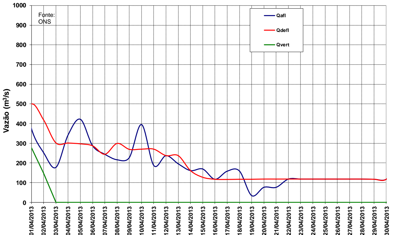
Figura 12 – Vazões na UHE Manso para o mês de abril de 2013.
