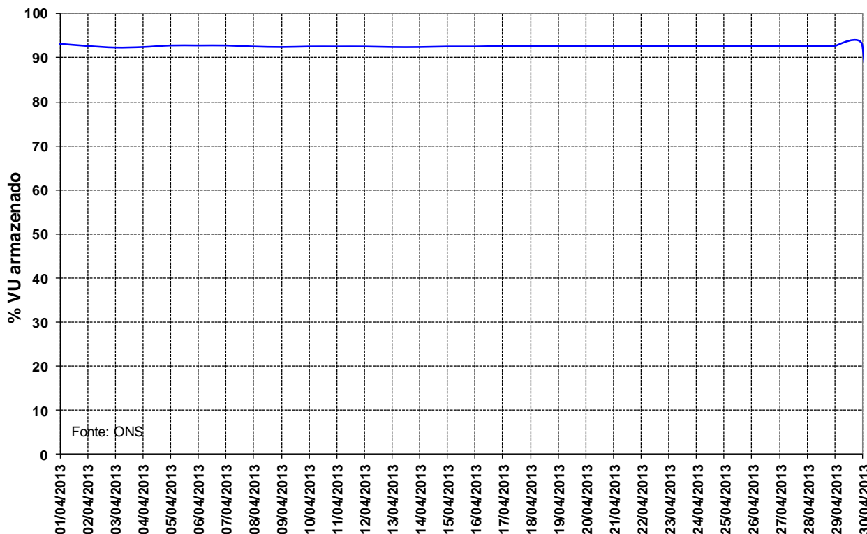
Figura 14 – Volume Útil armazenado na UHE Manso para o mês de abril de 2013.
