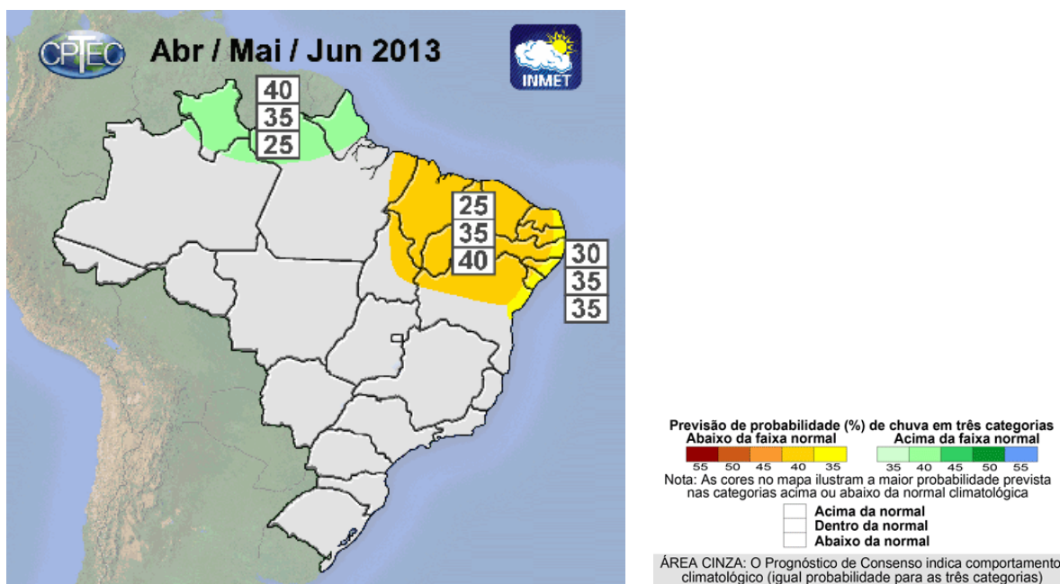
Figura 20 – Previsão climática para o trimestre abr / mai / jun de 2013.
