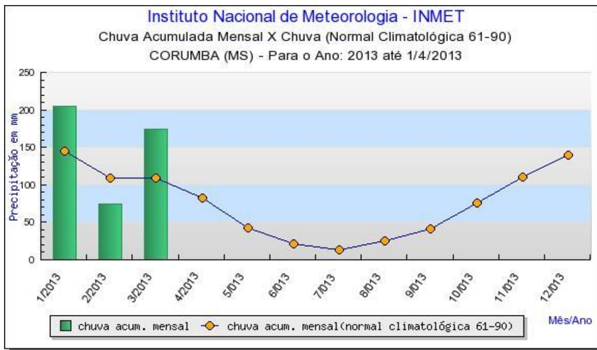
Figura 17 - Precipitação acumulada mensal em 2013 X Média climatológica (61-90) em Corumbá/MS
