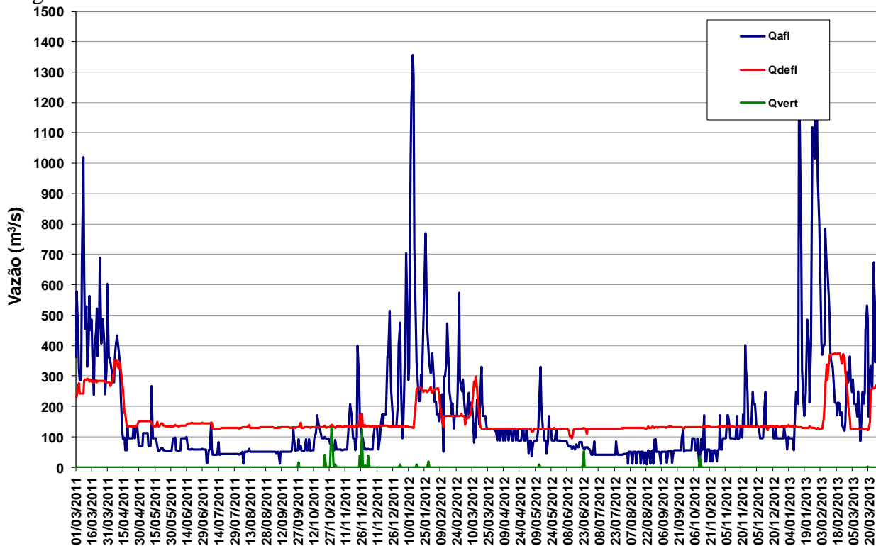
Figura 11 – Vazões na UHE Manso de março de 2011 a março de 2013.
