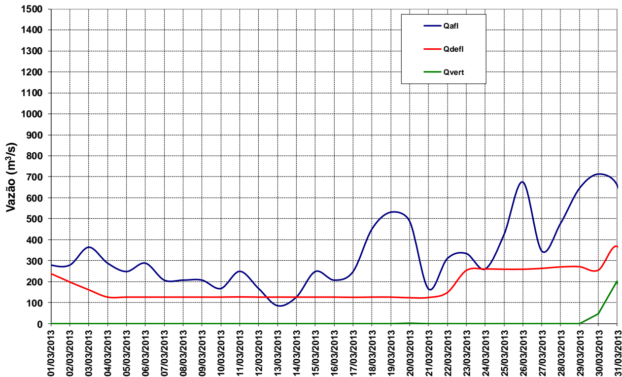
Figura 12 – Vazões na UHE Manso para o mês de março de 2013.
