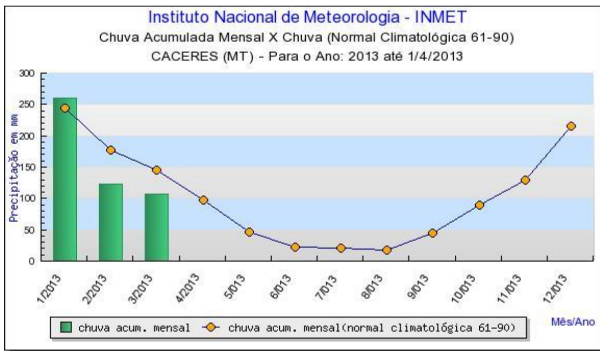
Figura 18 - Precipitação acumulada mensal em 2013 X Média climatológica (61-90) em Cáceres/MT
