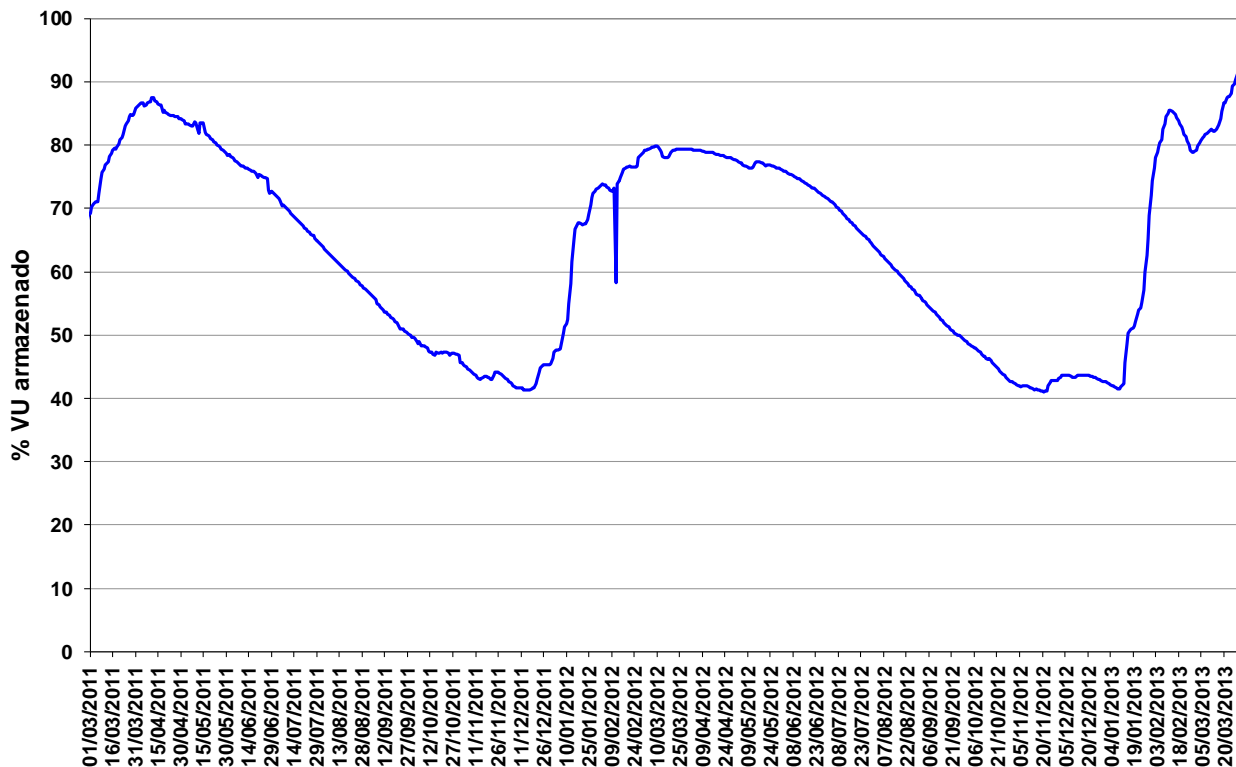
Figura 13 – Volume Útil armazenado na UHE Manso de março de 2011 a março de 2013.
