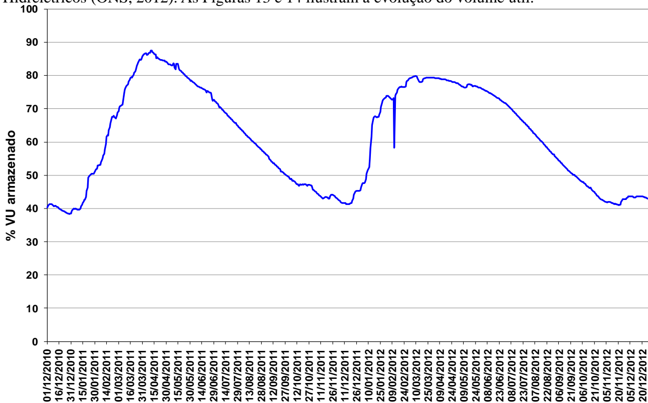
Figura 13 – Volume Útil armazenado na UHE Manso de dezembro de 2010 a dezembro de 2012.
