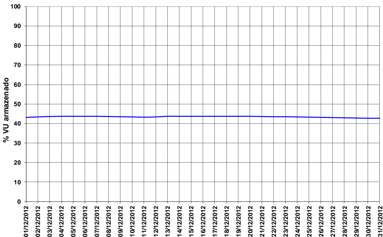
Figura 14 – Volume Útil armazenado na UHE Manso para o mês de dezembro de 2012.
