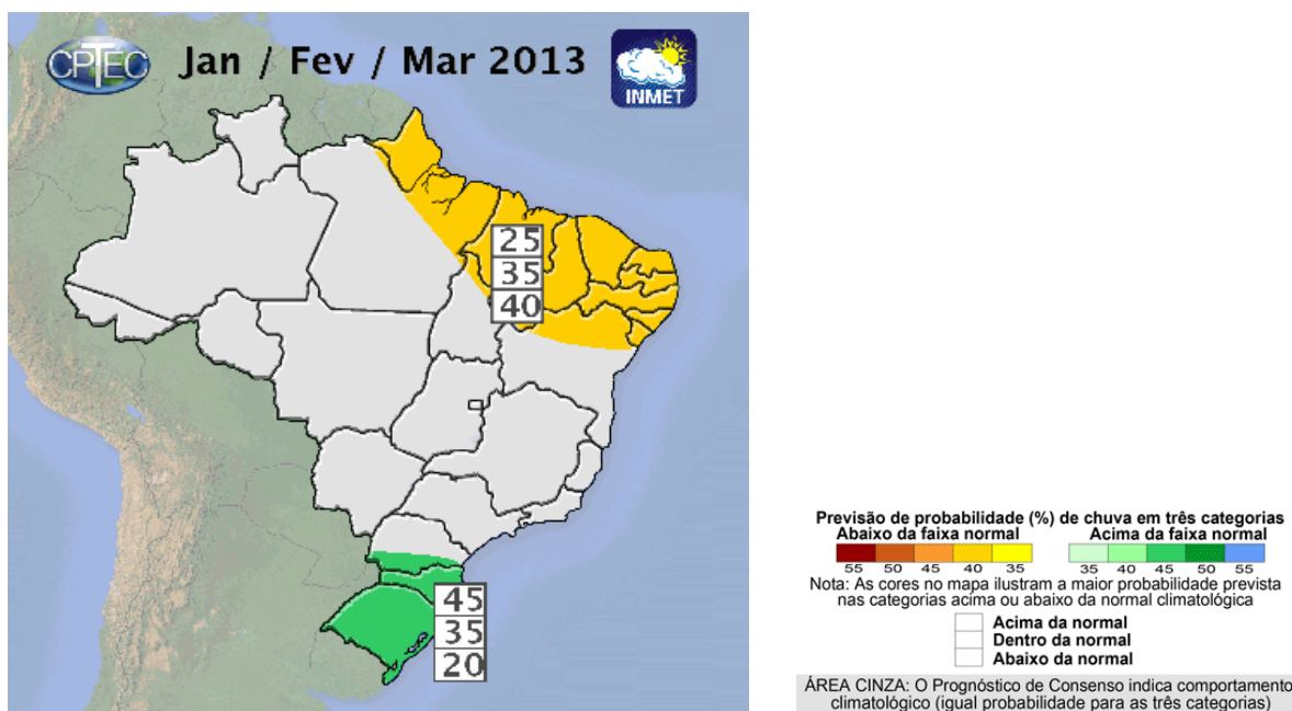
Figura 20 – Previsão climática para o trimestre jan / fev / mar de 2013.
