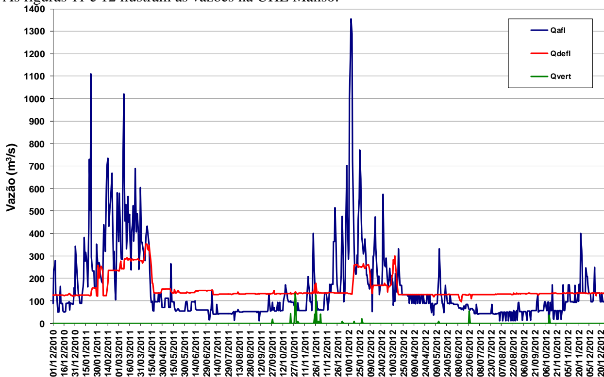
Figura 11 – Vazões na UHE Manso de dezembro de 2010 a dezembro de 2012.
