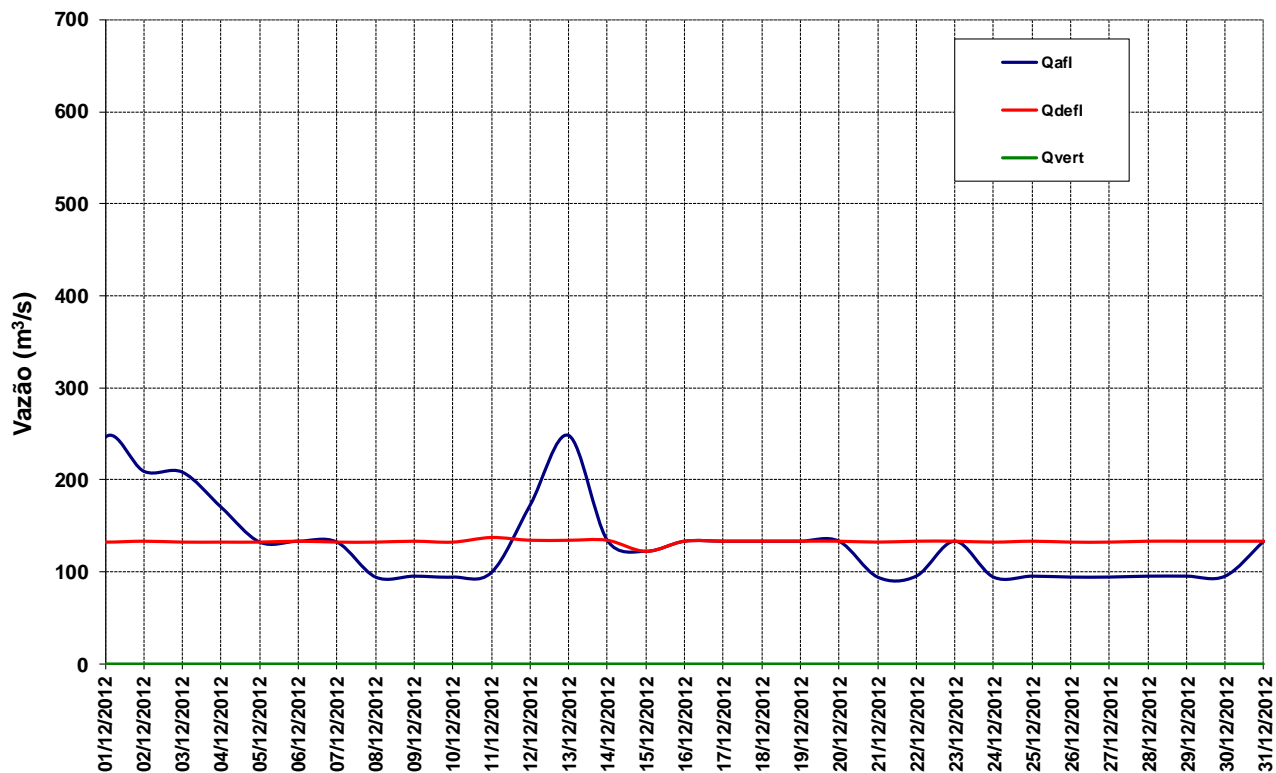
Figura 12 – Vazões na UHE Manso para o mês de dezembro de 2012.
