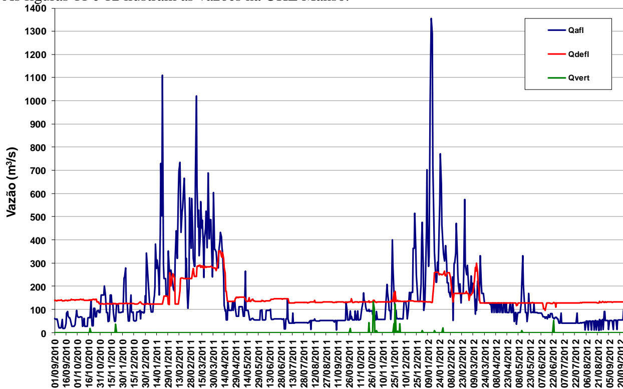
Figura 11 – Vazões na UHE Manso de setembro de 2010 a setembro de 2012.
