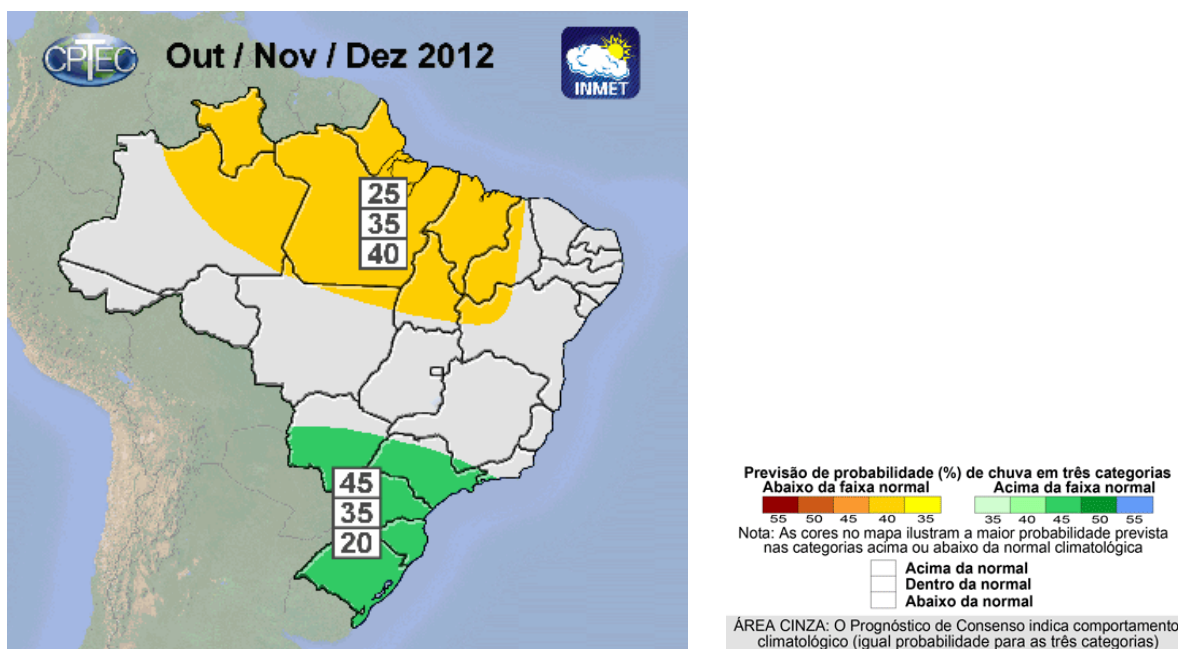
Figura 20 – Previsão climática para o trimestre out / nov / dez de 2012.
