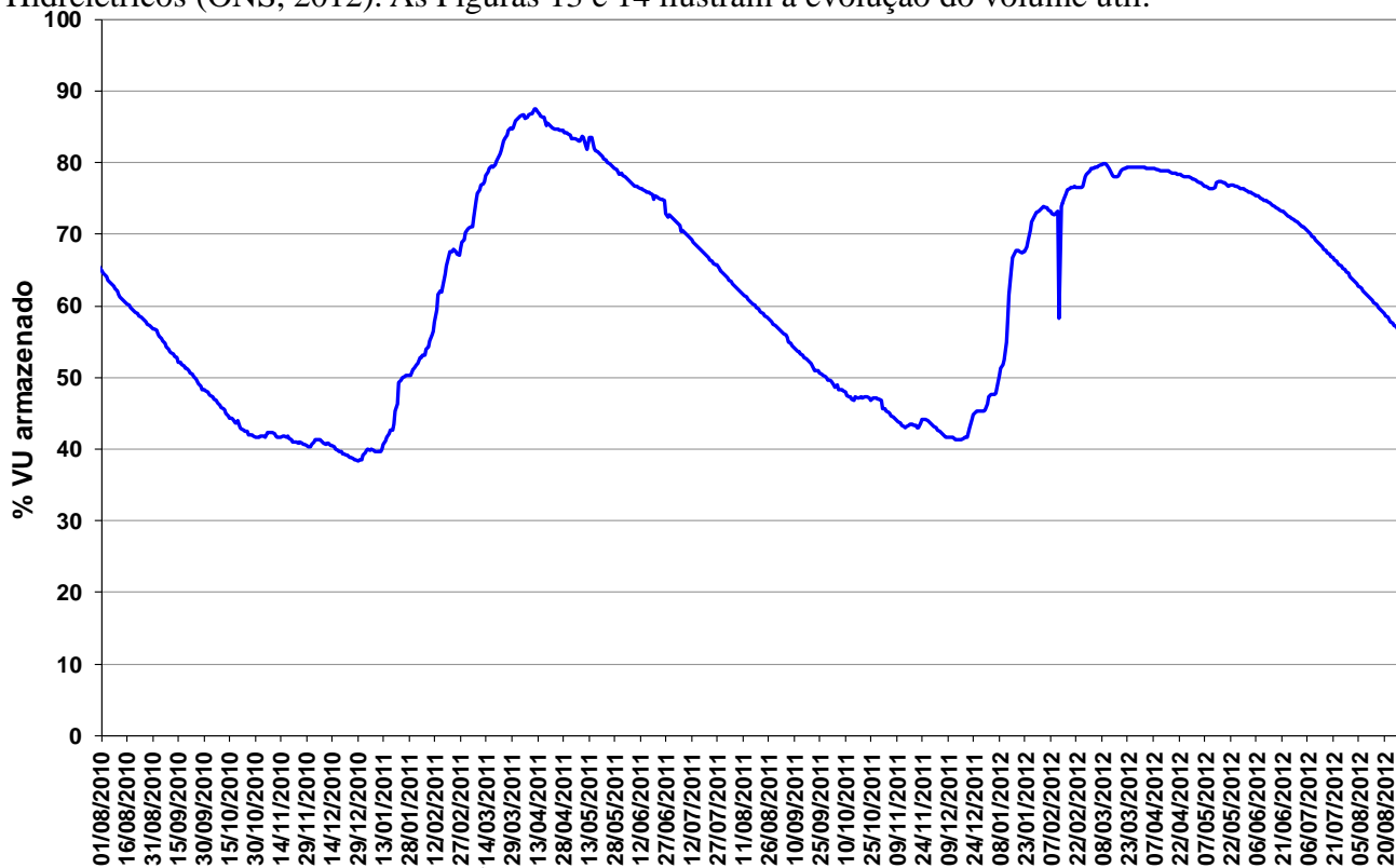
Figura 13 – Volume Útil na UHE Manso de agosto de 2010 a agosto de 2012.
