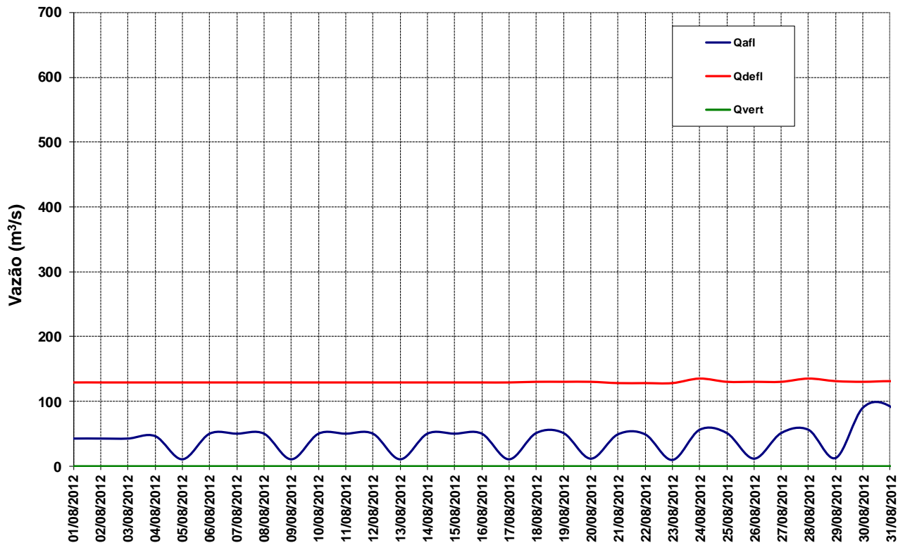
Figura 12 – Vazões na UHE Manso para o mês de agosto de 2012.
