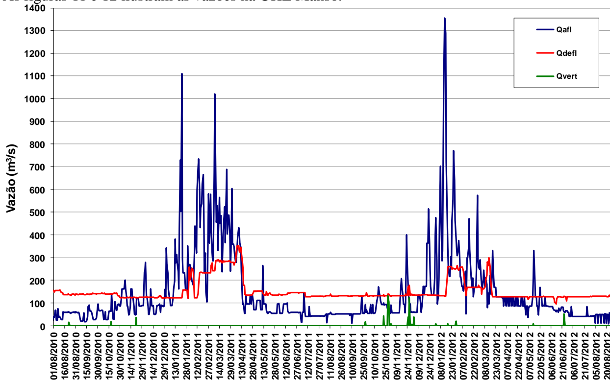
Figura 11 – Vazões na UHE Manso de agosto de 2010 a agosto de 2012.
