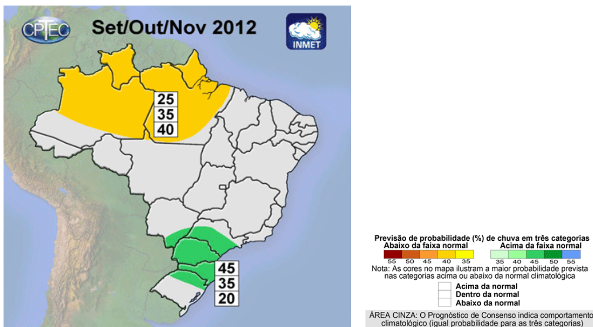
Figura 20 – Previsão climática para o trimestre set / out / nov de 2012.
