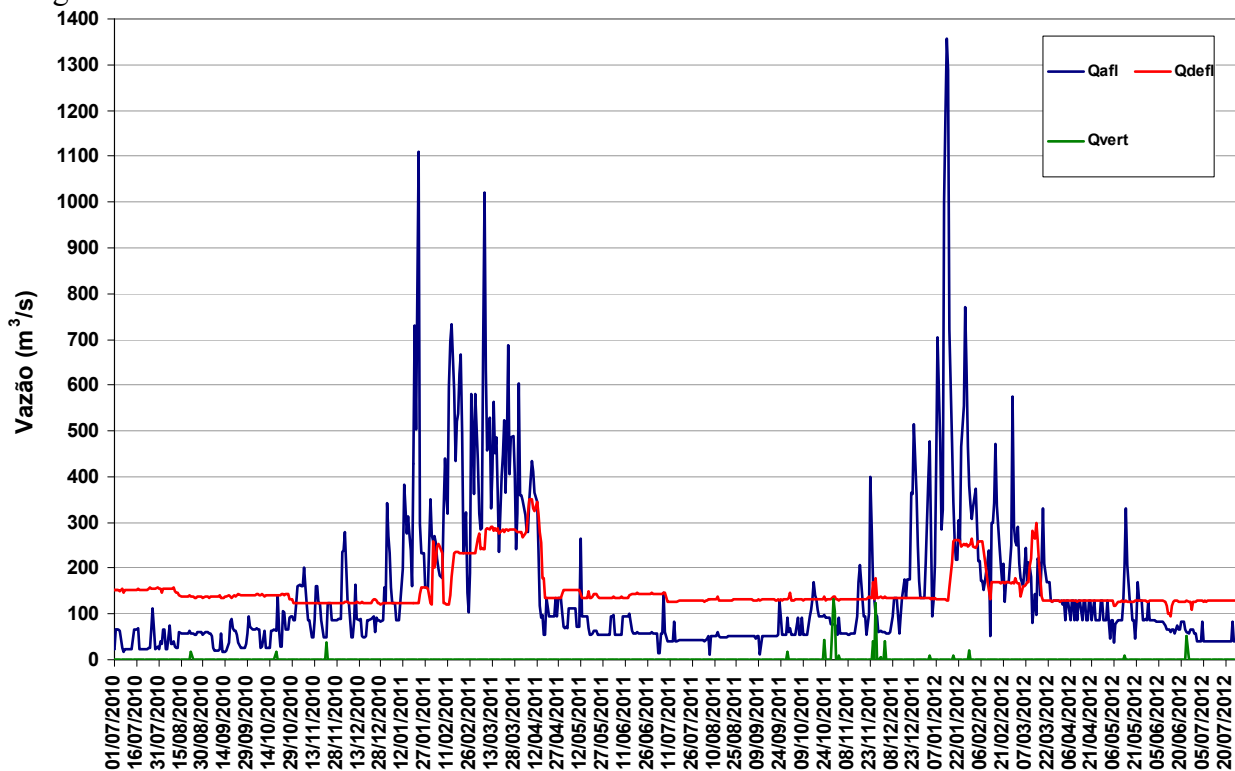
Figura 11 – Vazões na UHE Manso de julho de 2010 a julho de 2012.
