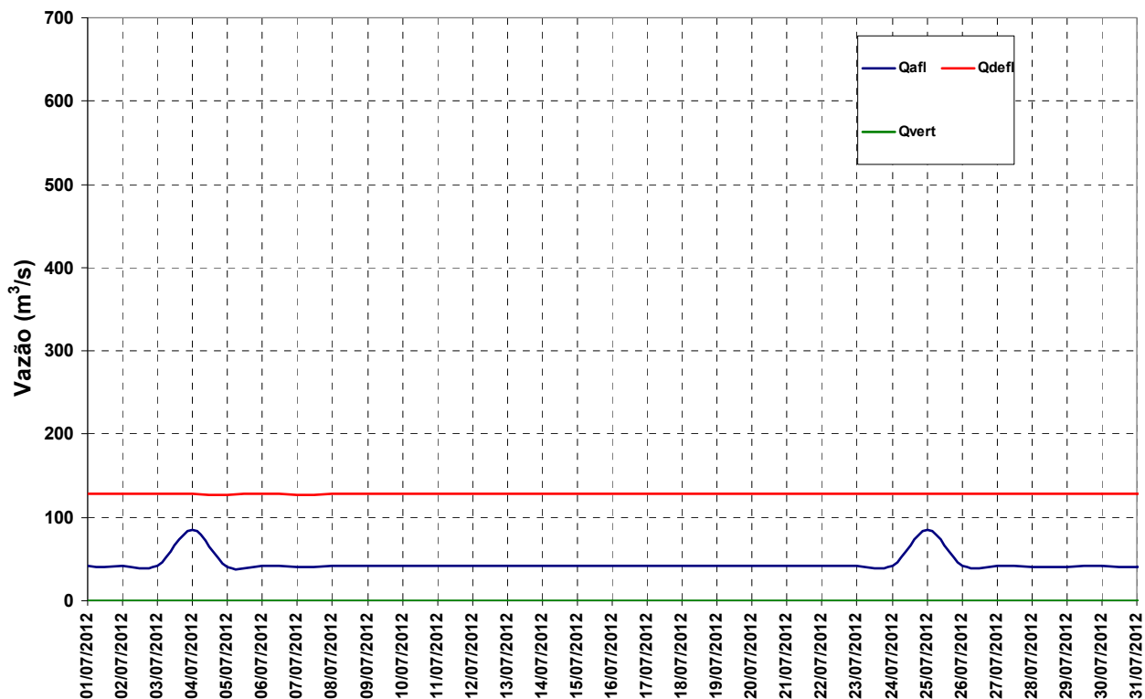
Figura 12 – Vazões na UHE Manso para o mês de julho de 2012.
