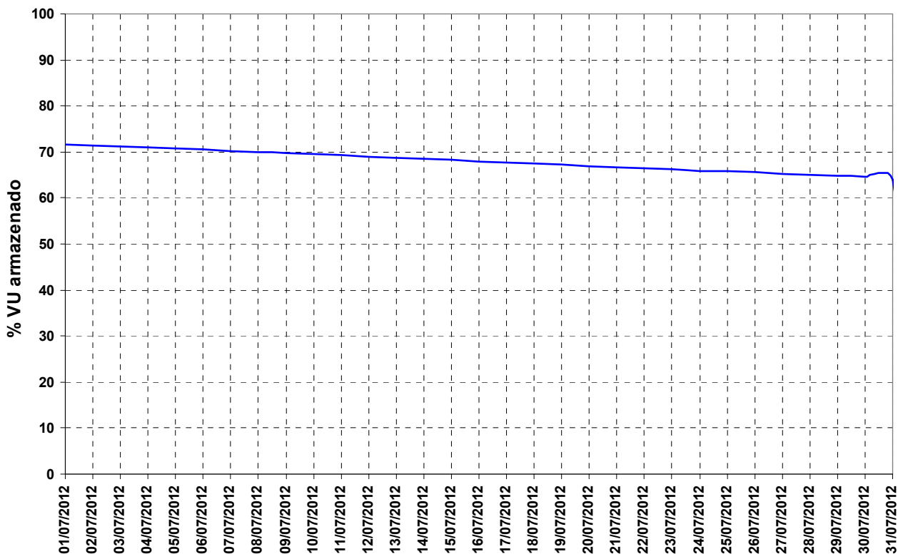
Figura 14 – Volume Útil na UHE Manso para o mês de julho de 2012.
