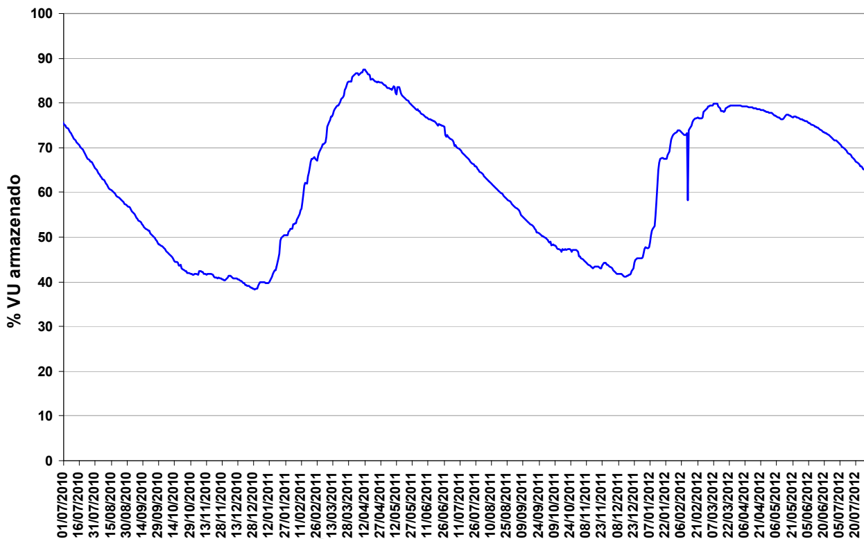
Figura 13 – Volume Útil na UHE Manso de julho de 2010 a julho de 2012.
