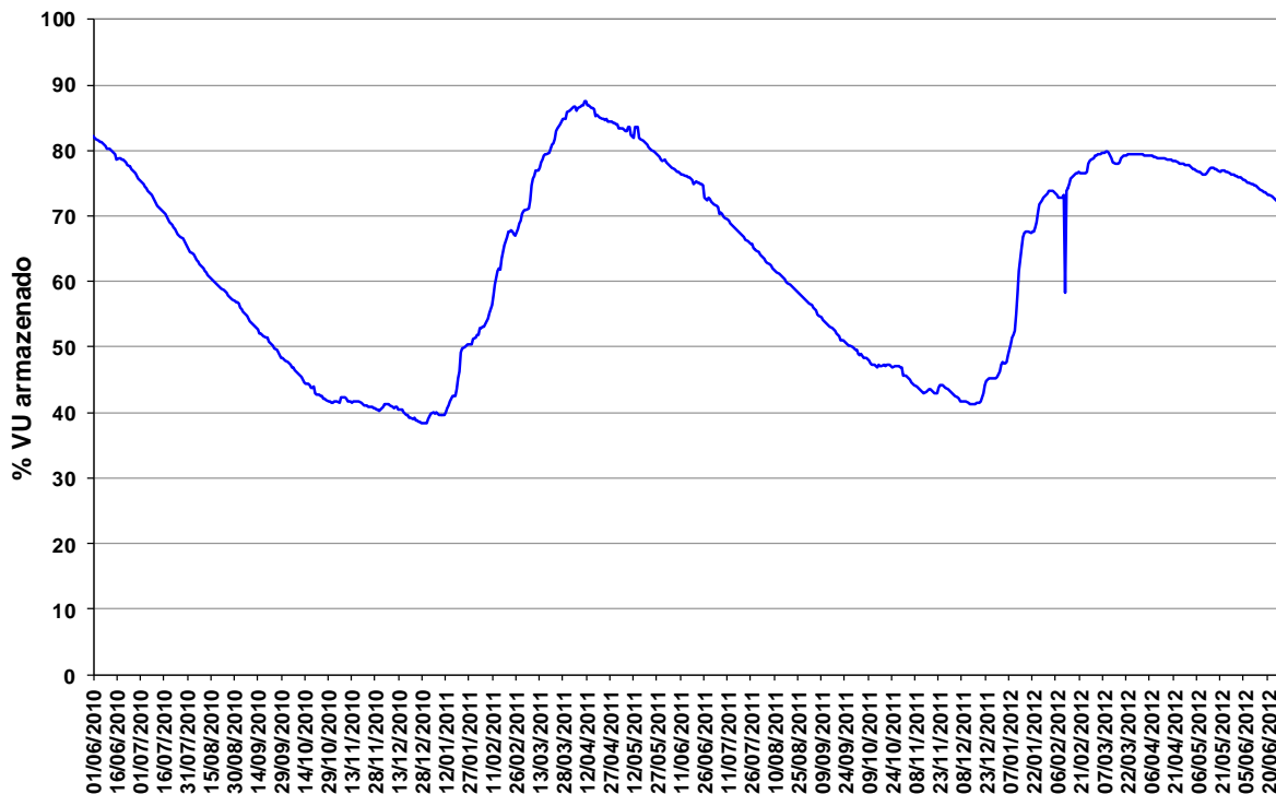
Figura 13 – Volume Útil na UHE Manso de junho de 2010 a junho de 2012.
