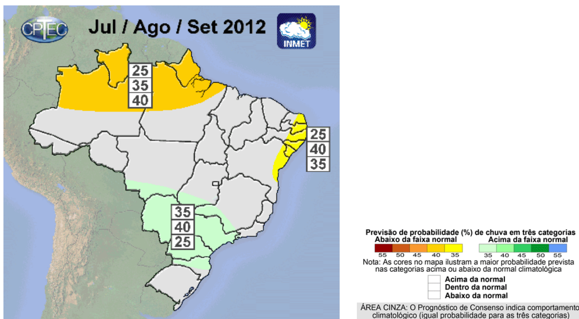
Figura 20 – Previsão climática para o trimestre jul / ago / set de 2012.
