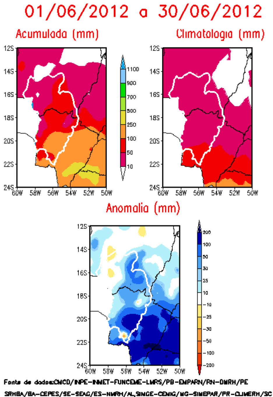
Figura 16 – Precipitação mensal acumulada, média climatológica e anomalia de precipitação na BAP, no período de 01/06/12 a 30/06/12.
