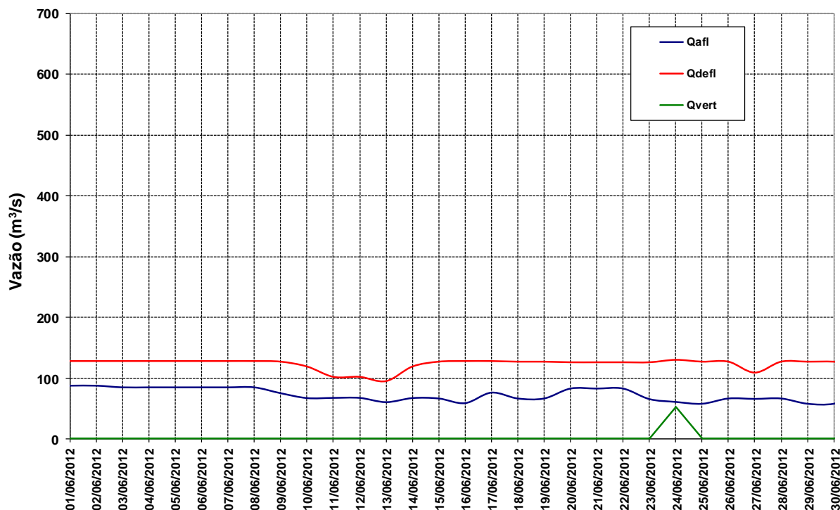
Figura 12 – Vazões na UHE Manso para o mês de junho de 2012.
