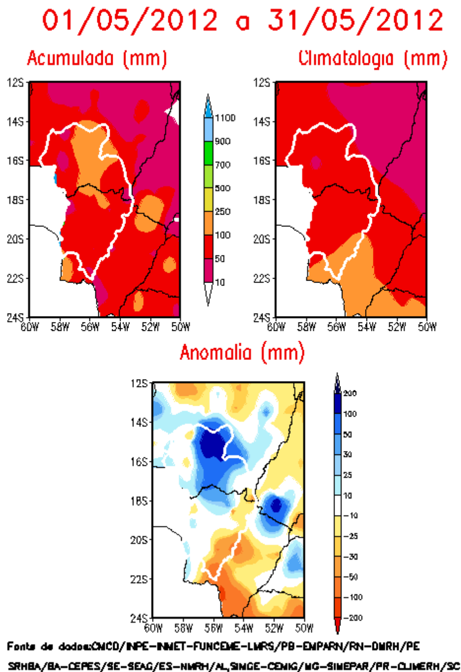
Figura 15 – Precipitação mensal acumulada, média climatológica e anomalia de precipitação na BAP, no período de 01/05/12 a 31/05/12.
