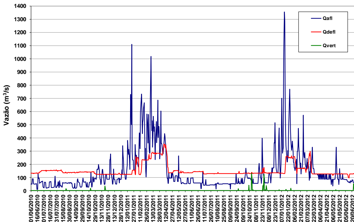
Figura 11 – Vazões na UHE Manso de junho de 2010 a junho de 2012.
