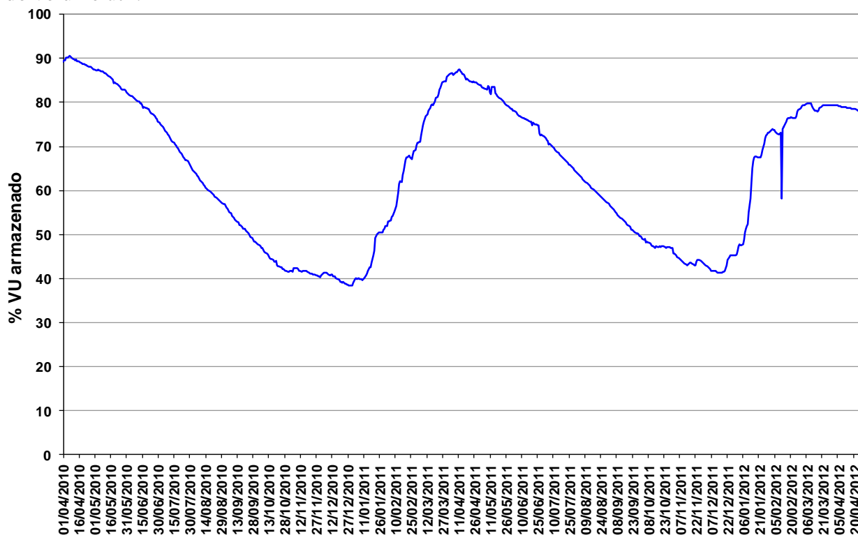
Figura 13 – Volume Útil na UHE Manso de abril de 2010 a abril de 2012.
