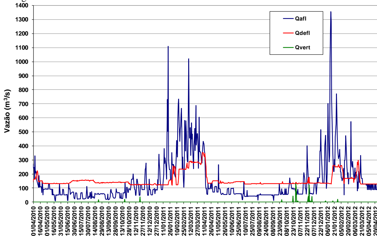
Figura 11 – Vazões na UHE Manso de abril de 2010 a abril de 2012.
