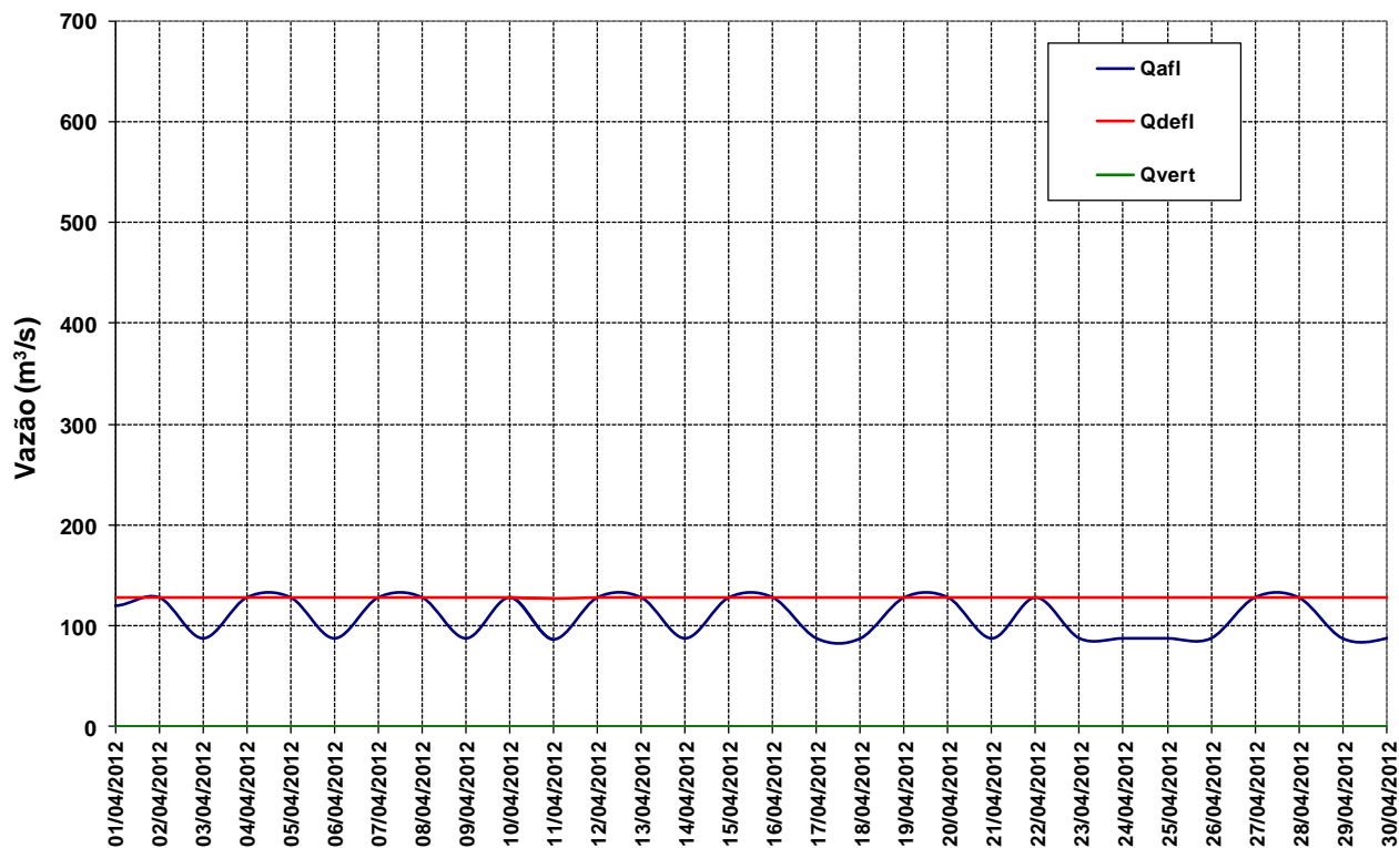
Figura 12 – Vazões na UHE Manso para o mês de abril de 2012.
