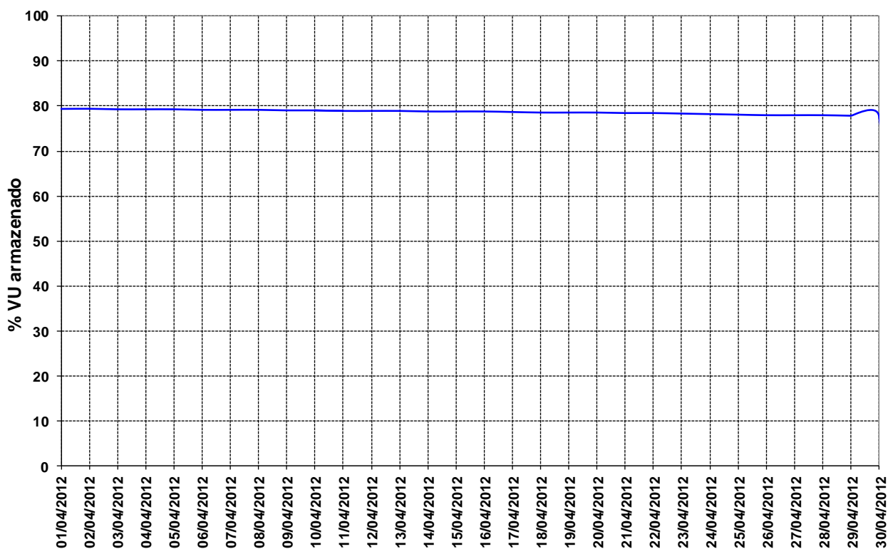
Figura 14 – Volume Útil na UHE Manso para o mês de abril de 2012.
