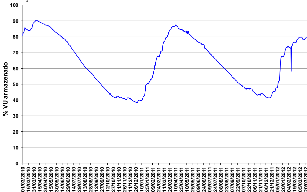
Figura 13 – Volume Útil na UHE Manso de março de 2010 a março de 2012.
