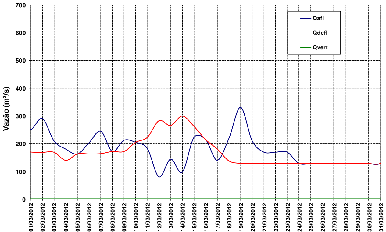
Figura 12 – Vazões na UHE Manso para o mês de março de 2012.
