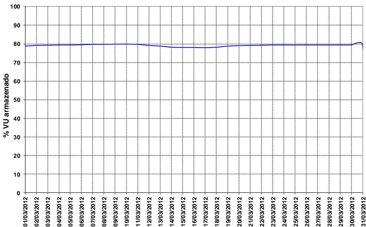
Figura 14 – Volume Útil na UHE Manso para o mês de março de 2012.
