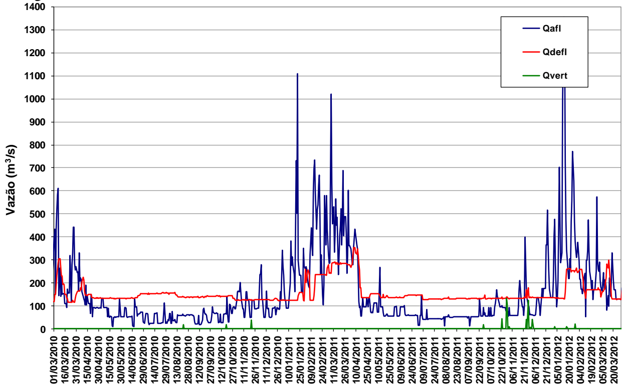
Figura 11 – Vazões na UHE Manso de março de 2010 a março de 2012.
