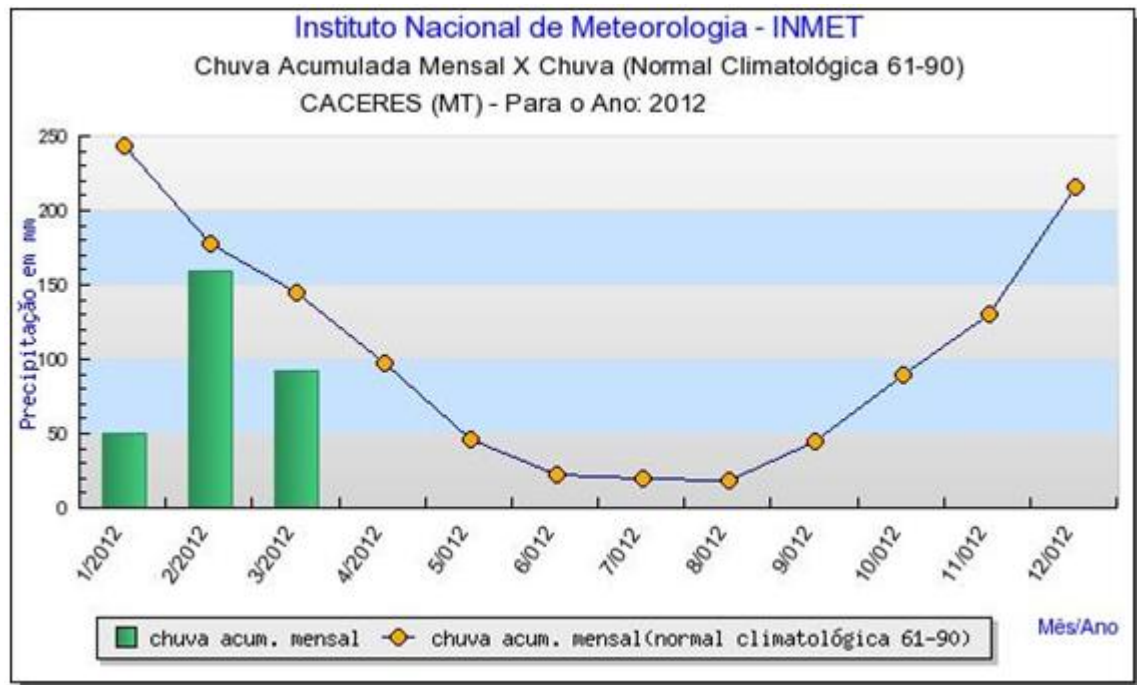
Figura 18 - Precipitação acumulada mensal em 2012 X Média climatológica (61-90) em Cáceres/MT
