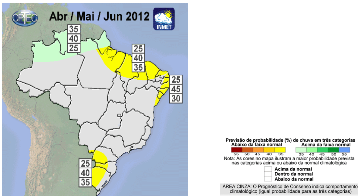
Figura 20 – Previsão climática para o trimestre abr / mai / jun de 2012.
