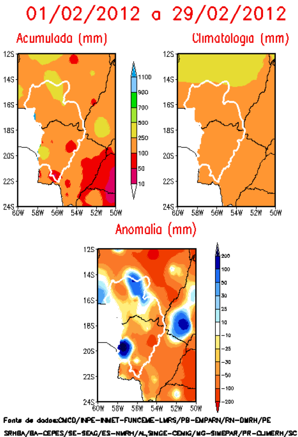
Figura 15 – Precipitação mensal acumulada, média climatológica e anomalia de precipitação na BAP, no período de 01/02/12 a 29/02/12.
