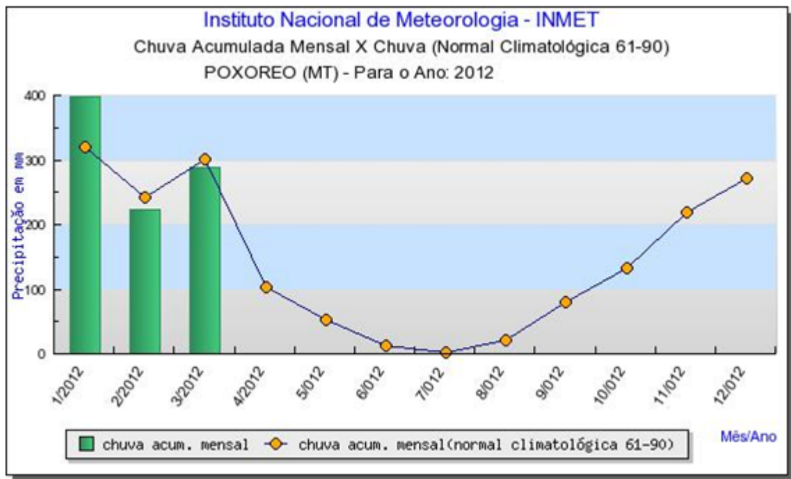
Figura 17 - Precipitação acumulada mensal em 2012 X Média climatológica (61-90) em Poxoréo/MT
