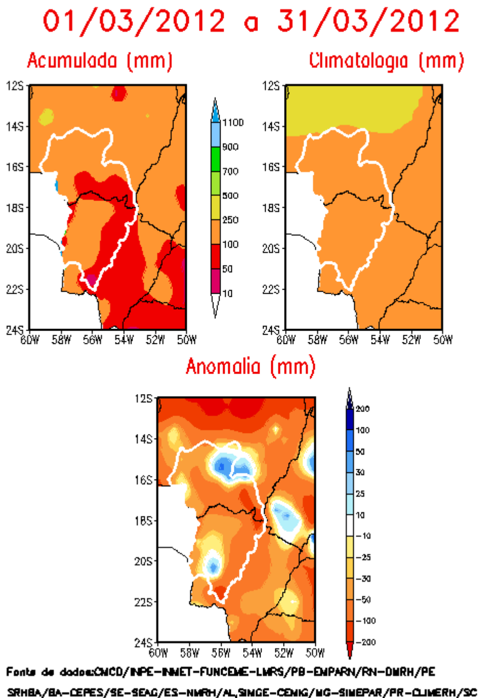
Figura 16 – Precipitação mensal acumulada, média climatológica e anomalia de precipitação na BAP, no período de 01/03/12 a 31/03/12.
