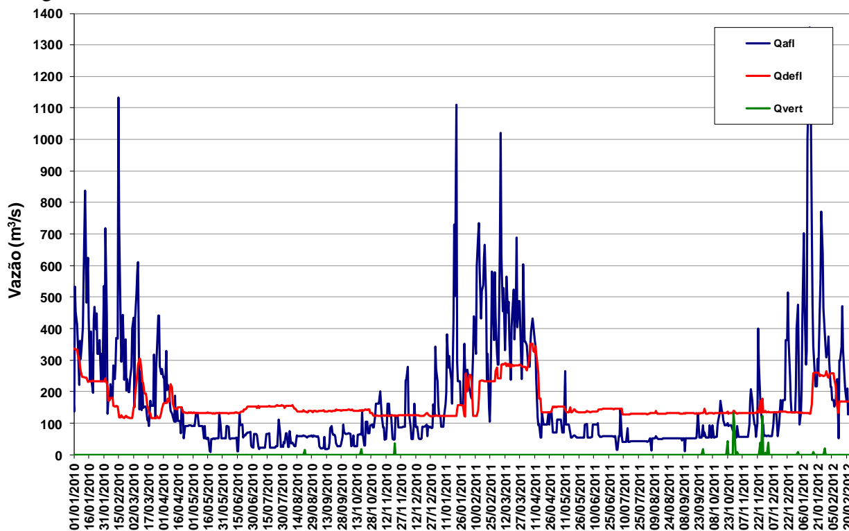
Figura 11 – Vazões na UHE Manso de janeiro de 2010 a fevereiro de 2012.
