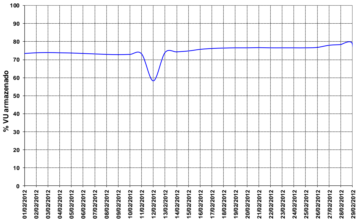
Figura 14 – Volume Útil na UHE Manso para o mês de fevereiro de 2012.
