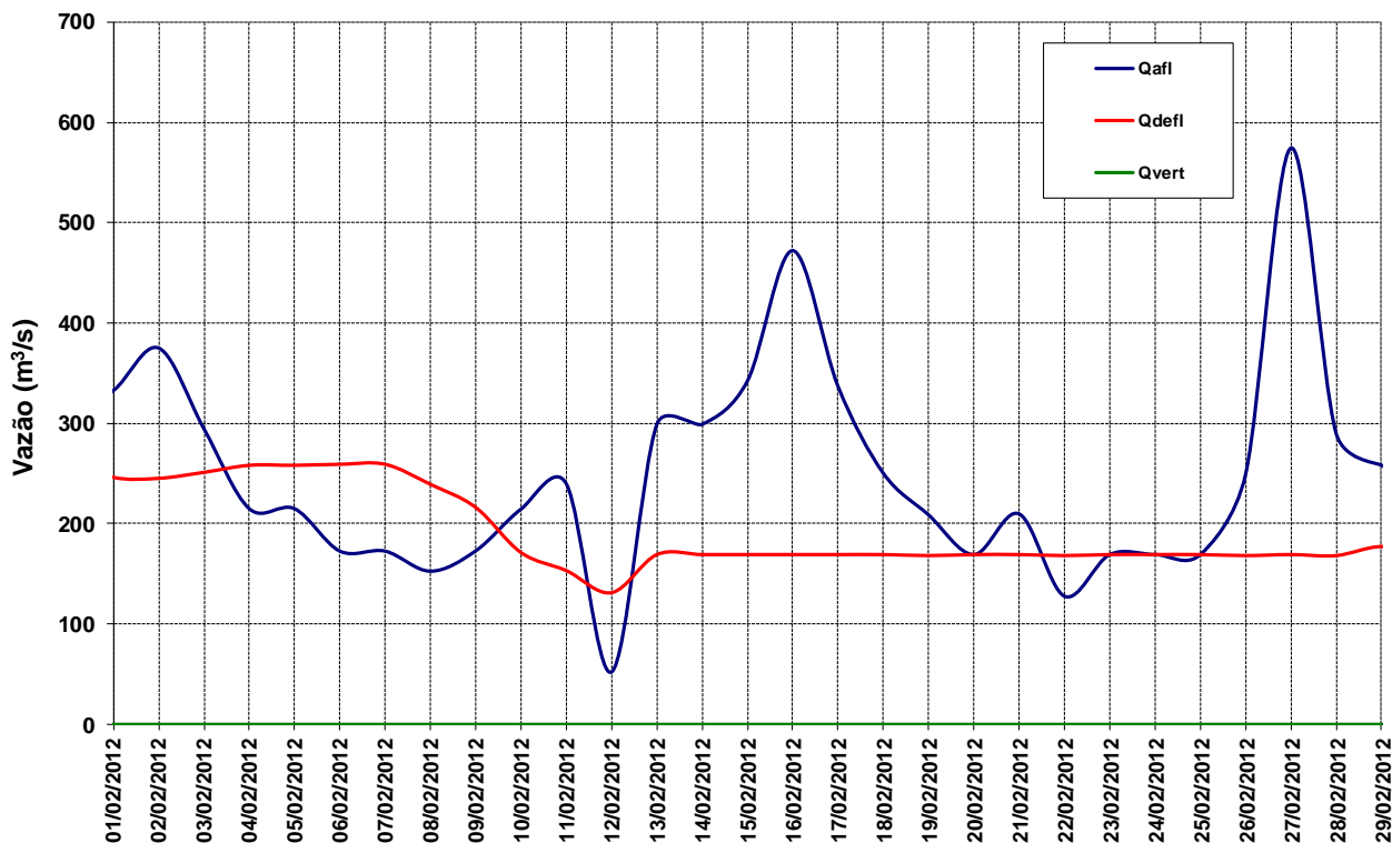
Figura 12 – Vazões na UHE Manso para o mês de fevereiro de 2012.
