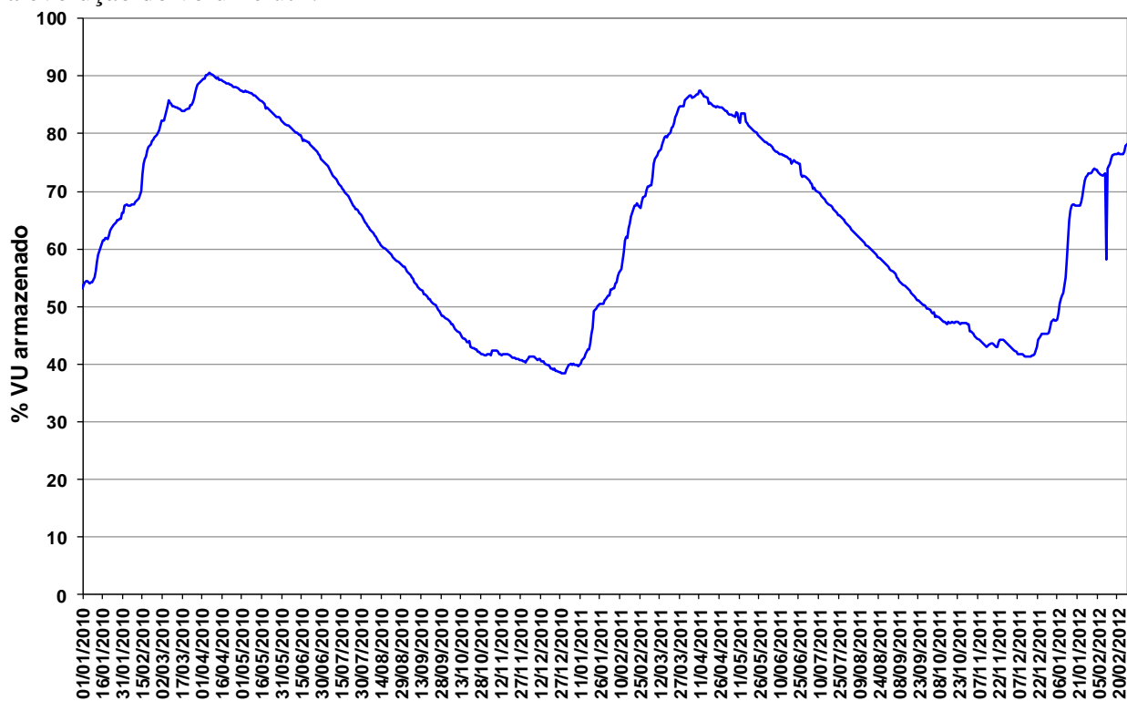
Figura 13 – Volume Útil na UHE Manso de janeiro de 2010 a fevereiro de 2012.
