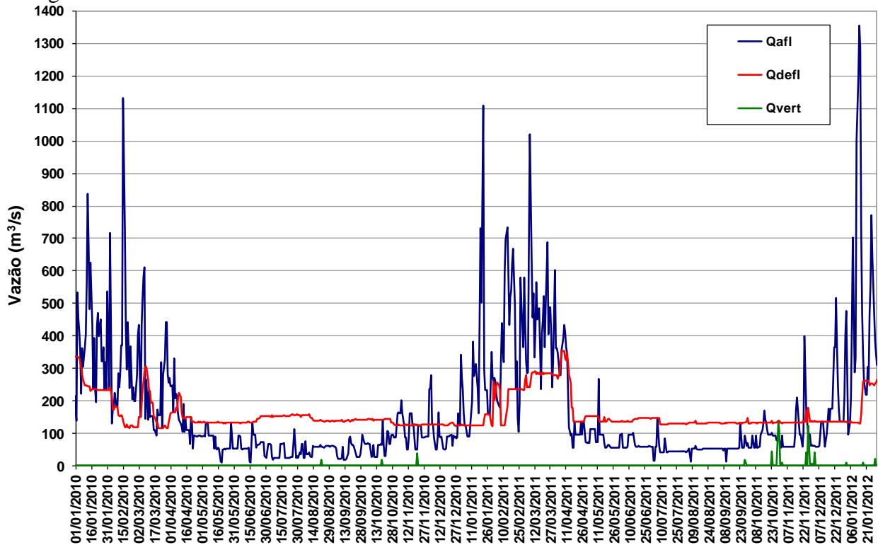
Figura 11 – Vazões na UHE Manso de janeiro de 2010 a janeiro de 2012.
