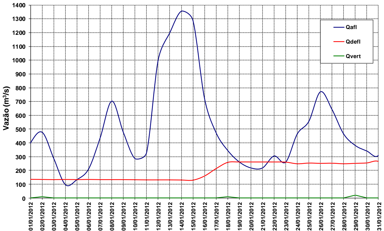
Figura 12 – Vazões na UHE Manso para o mês de janeiro de 2012.
