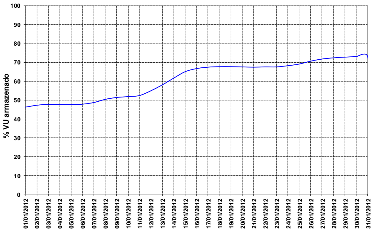
Figura 14 – Volume Útil na UHE Manso para o mês de janeiro de 2012.
