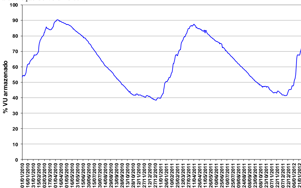
Figura 13 – Volume Útil na UHE Manso de janeiro de 2010 a janeiro de 2012.
