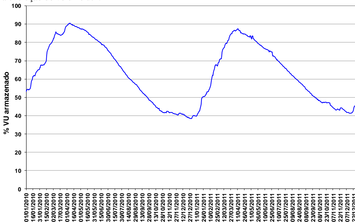
Figura 13 – Volume Útil na UHE Manso de janeiro de 2010 a dezembro de 2011.
