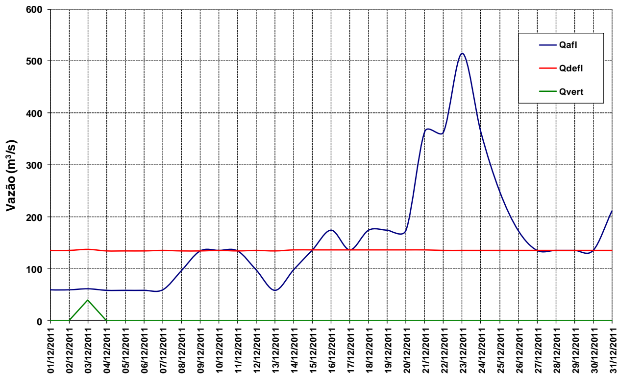
Figura 12 – Vazões na UHE Manso para o mês de dezembro de 2011.
