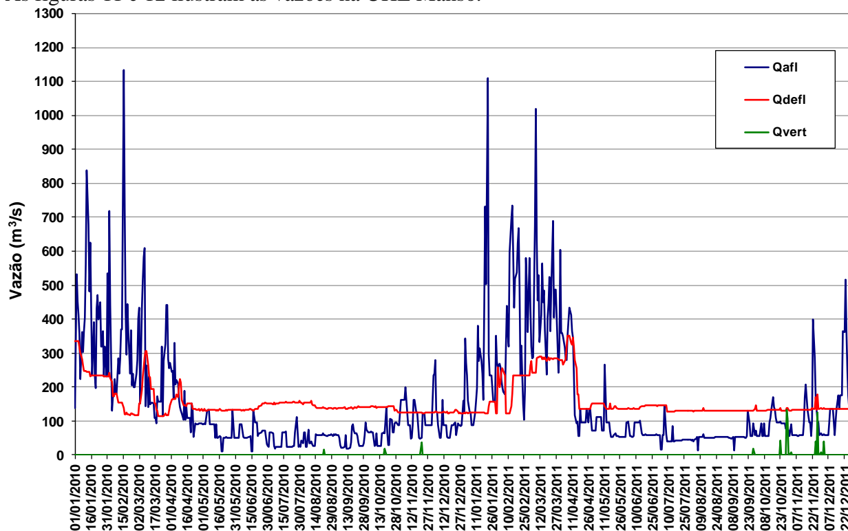
Figura 11 – Vazões na UHE Manso de janeiro de 2010 a dezembro de 2011.
