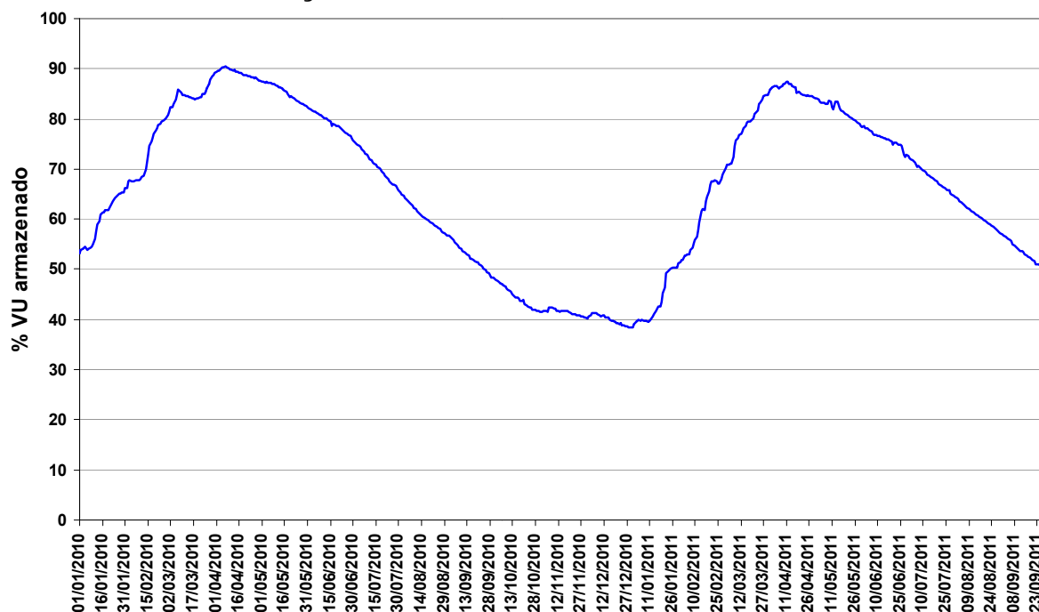
Figura 13 – Volume Útil na UHE Manso de janeiro de 2010 a setembro de 2011.
