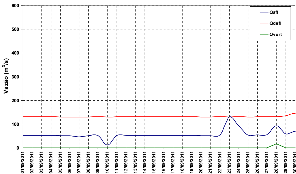
Figura 12 – Vazões na UHE Manso para o mês de setembro de 2011.
