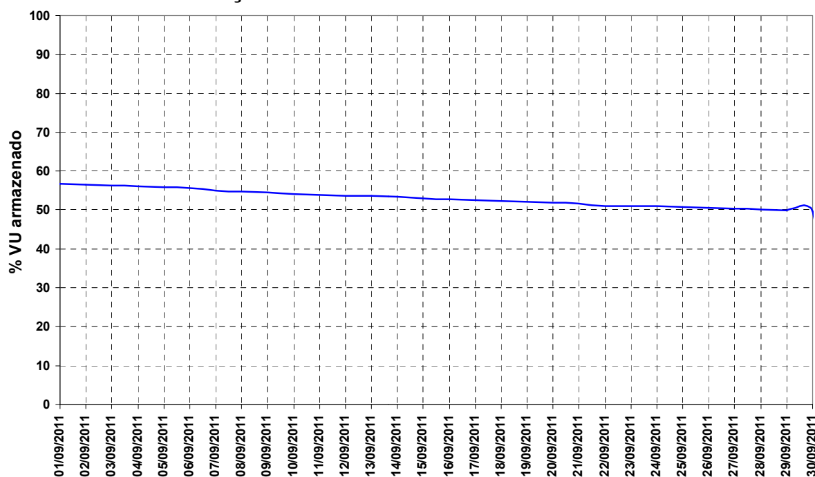
Figura 14 – Volume Útil na UHE Manso para o mês de setembro de 2011.
