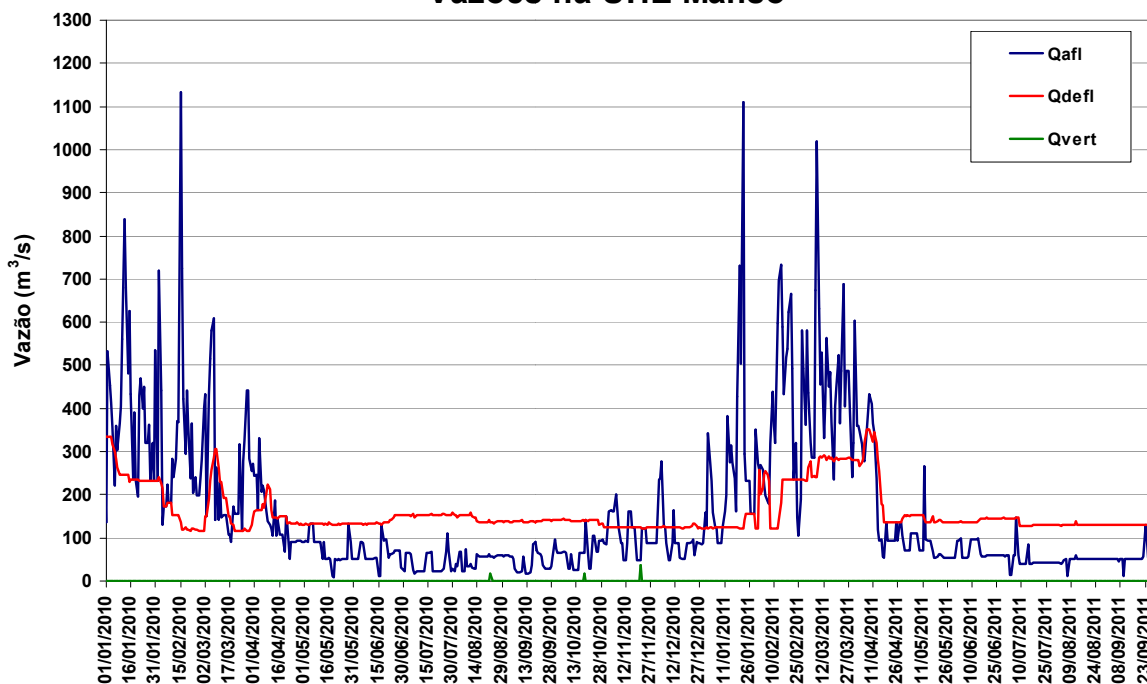
Figura 11 – Vazões na UHE Manso de janeiro de 2010 a setembro de 2011.
