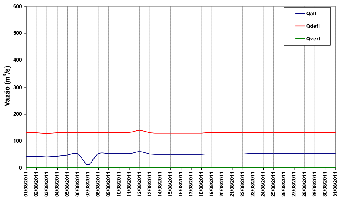
Figura 12 – Vazões na UHE Manso para o mês de agosto de 2011.
