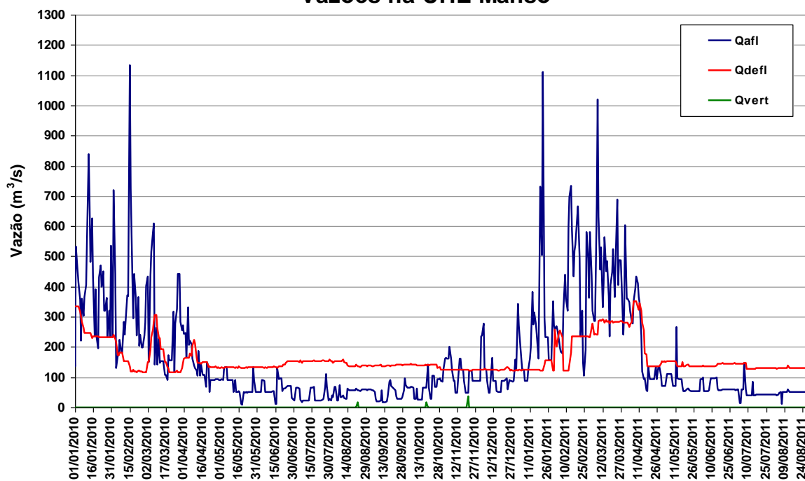
Figura 11 – Vazões na UHE Manso de janeiro de 2010 a agosto de 2011.
