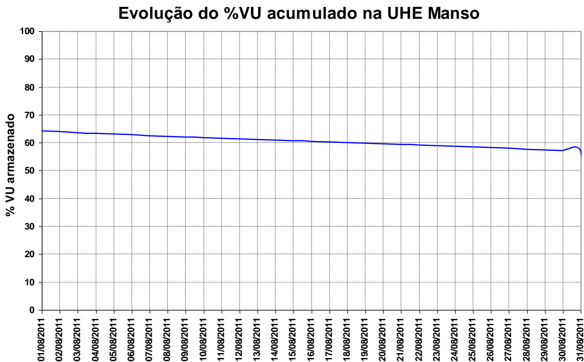
Figura 14 – Volume Útil na UHE Manso para o mês de agosto de 2011.
