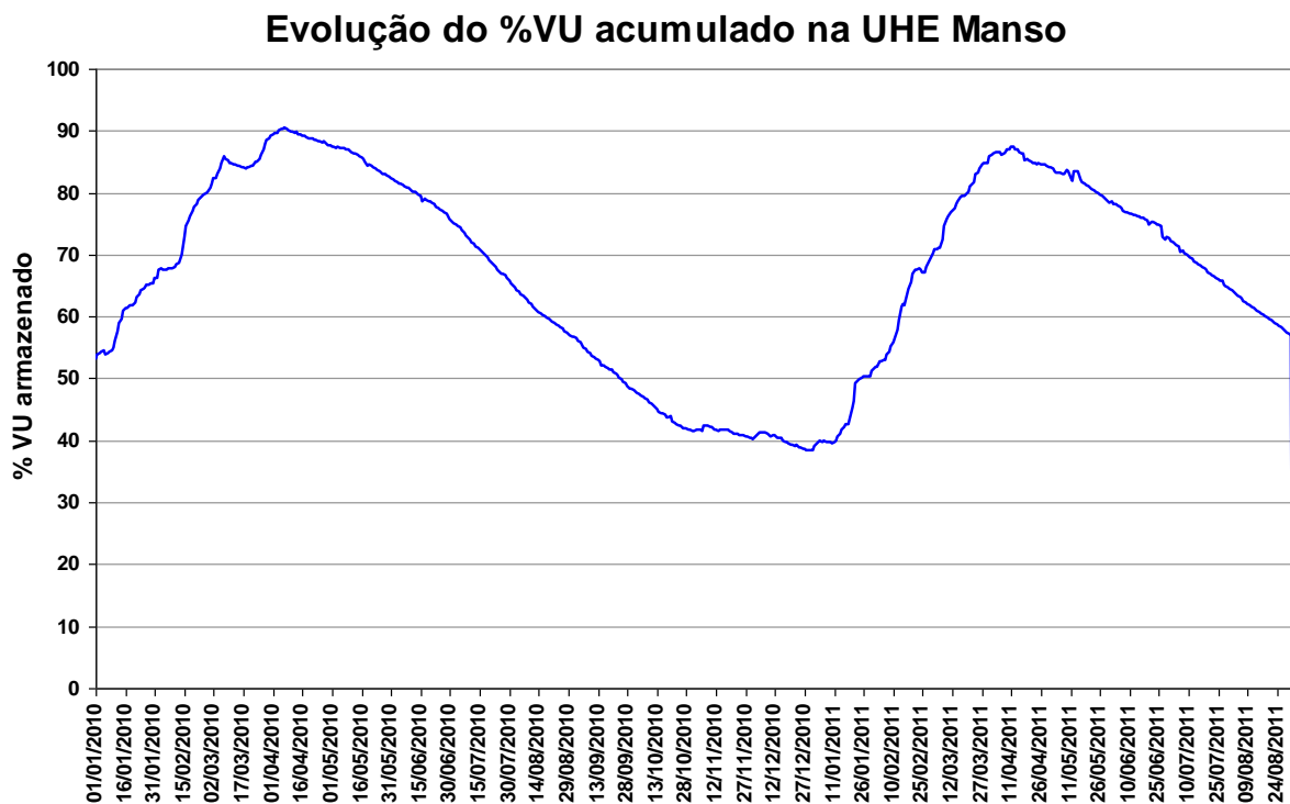
Figura 13 – Volume Útil na UHE Manso de janeiro de 2010 a agosto de 2011.
