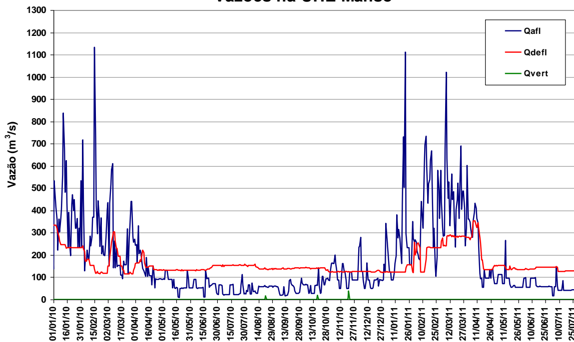
Figura 11 – Vazões na UHE Manso de janeiro de 2010 a julho de 2011.
