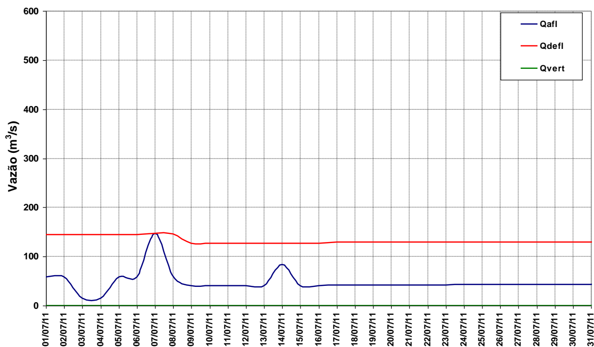
Figura 12 – Vazões na UHE Manso para o mês de julho de 2011.
