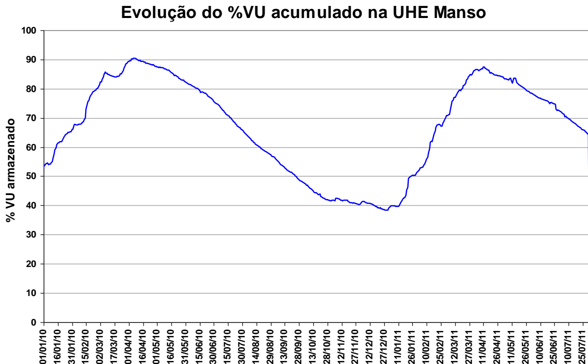
Figura 13 – Volume Útil na UHE Manso de janeiro de 2010 a julho de 2011.
