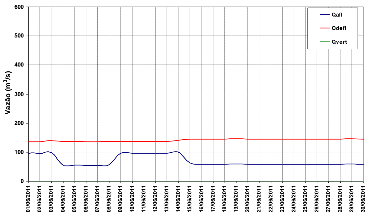
Figura 12 – Vazões na UHE Manso para o mês de junho de 2011.
