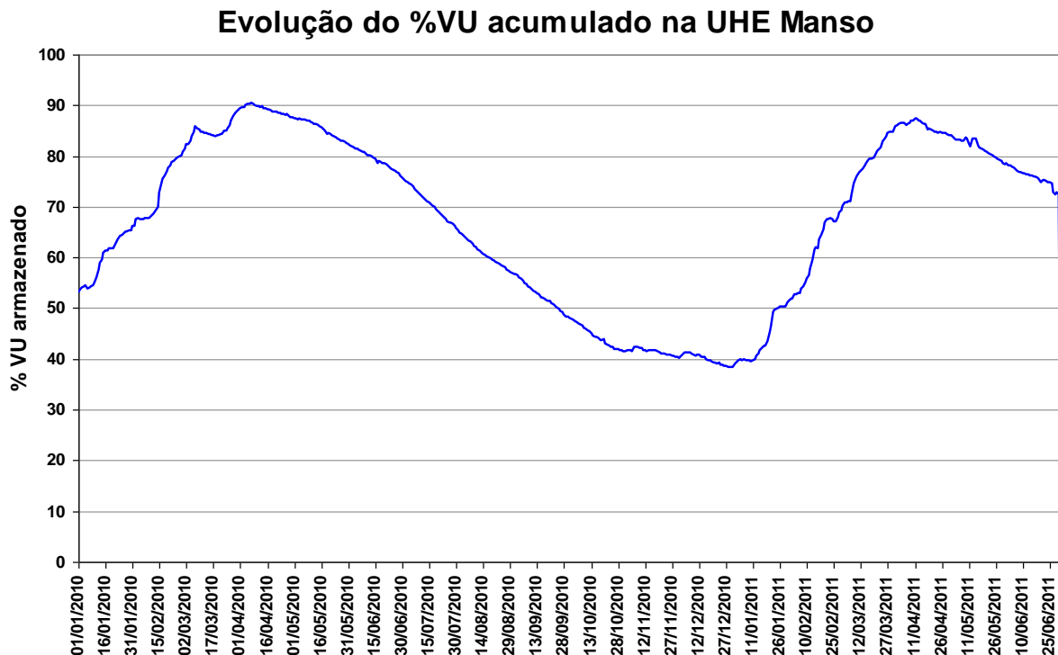
Figura 13 – Volume Útil na UHE Manso de janeiro de 2010 a junho de 2011.
