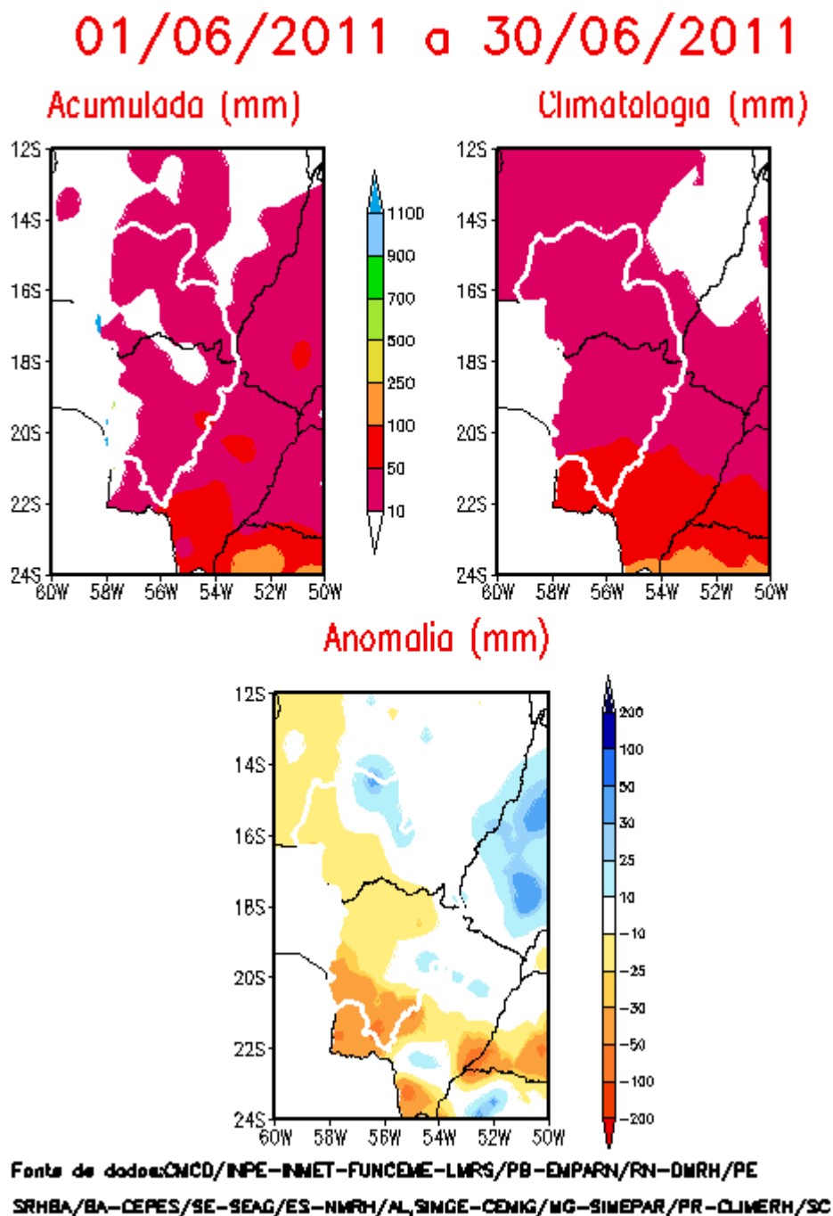
Figura 16 – Precipitação mensal acumulada, média climatológica e anomalia de precipitação na BAP, no período de 01/06/11 a 30/06/11.
