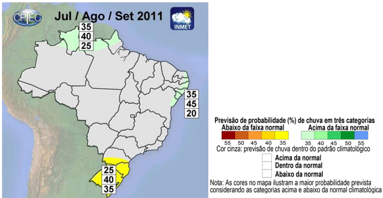
Figura 20 – Previsão climática para o trimestre jul / ago / set de 2011.
