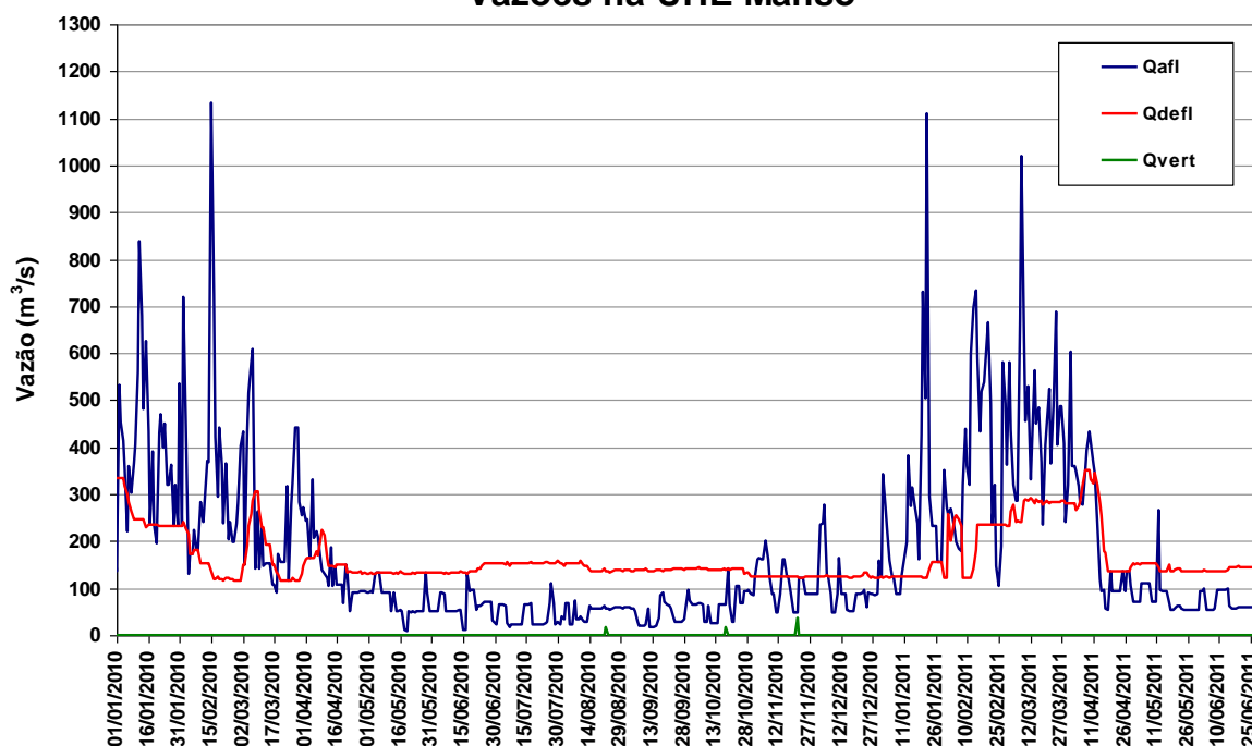
Figura 11 – Vazões na UHE Manso de janeiro de 2010 a junho de 2011.
