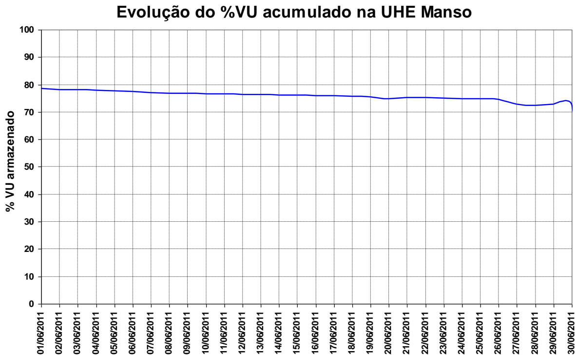
Figura 14 – Volume Útil na UHE Manso para o mês de junho de 2011.
