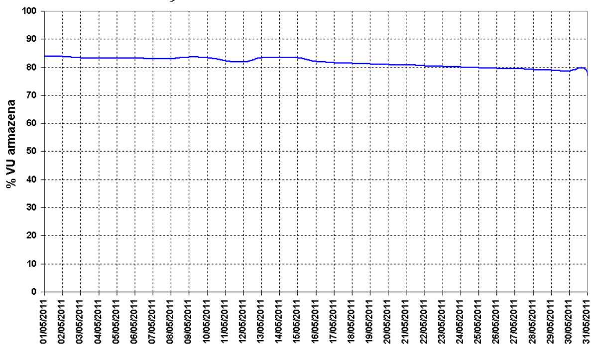
Figura 14 – Volume Útil na UHE Manso para o mês de maio de 2011.
