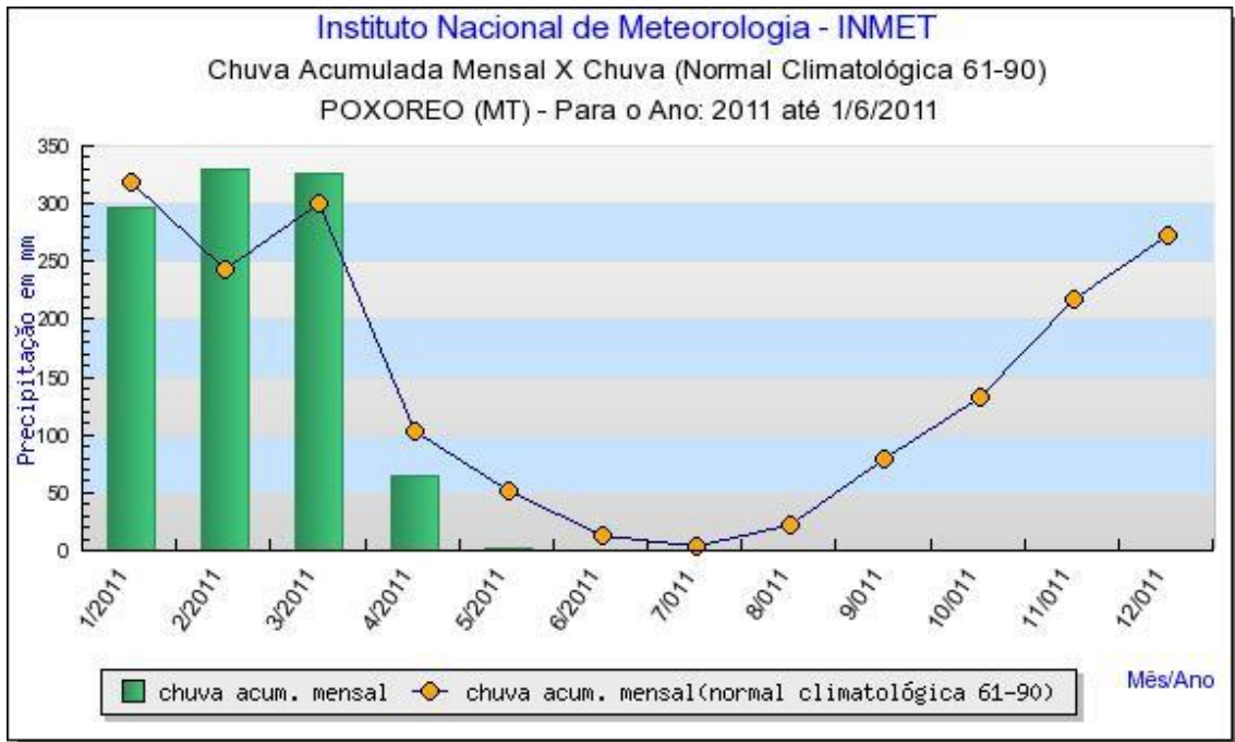
Figura 17 - Precipitação acumulada mensal em 2011 X Média climatológica (61-90) em Poxoréo/MT
