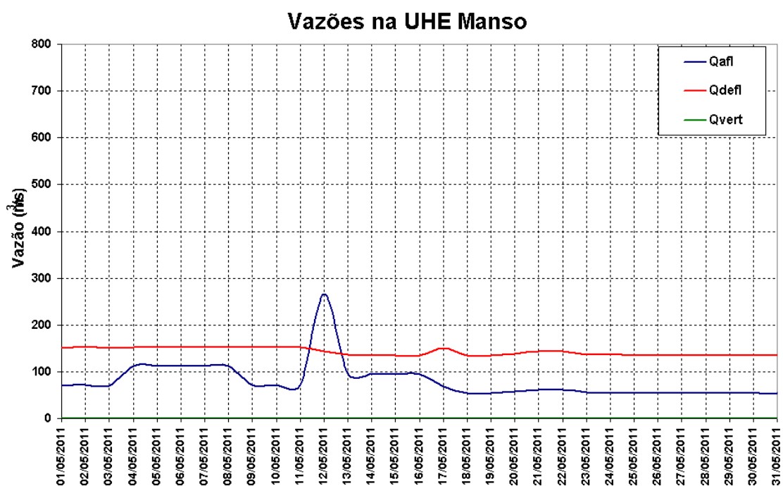
Figura 12 – Vazões na UHE Manso para o mês de maio de 2011.
