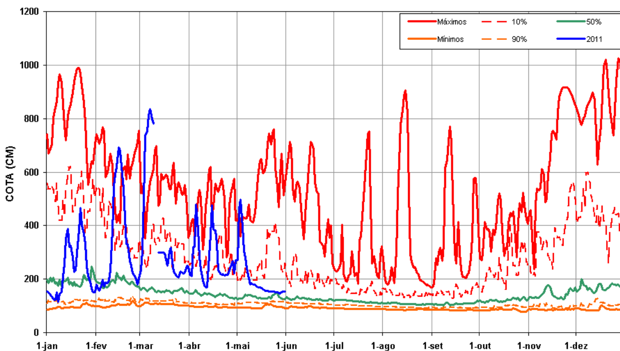
Figura 10 - Gráficos de permanência de cotas, cotas máximas, mínimas e observadas no rio Miranda, na Estrada MT – 738.
