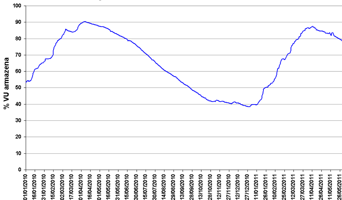
Figura 13 – Volume Útil na UHE Manso de janeiro de 2010 a maio de 2011.
