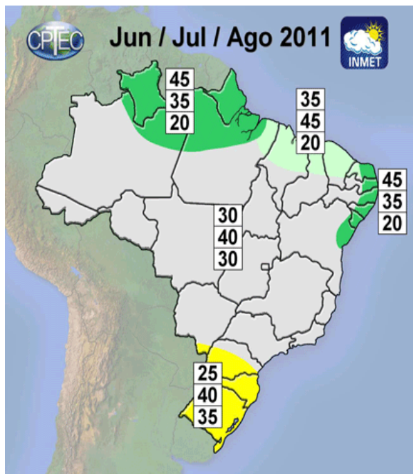
Figura 20 – Previsão climática para o trimestre jun / jul / ago de 2011.
