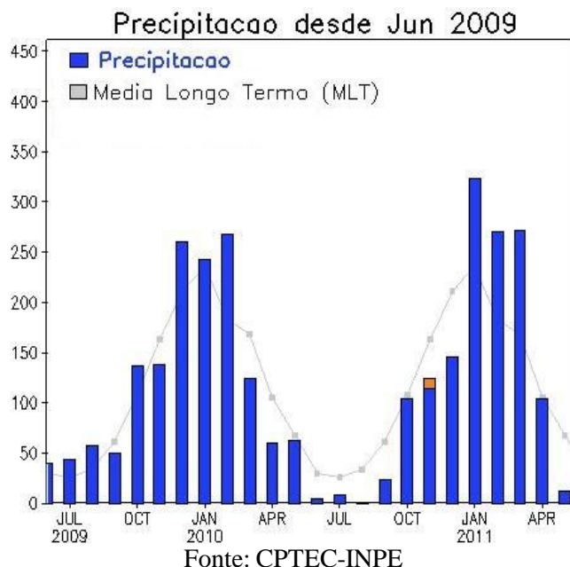
Figura 19 – Evolução da Precipitação Média na Bacia do Alto Paraguai.
