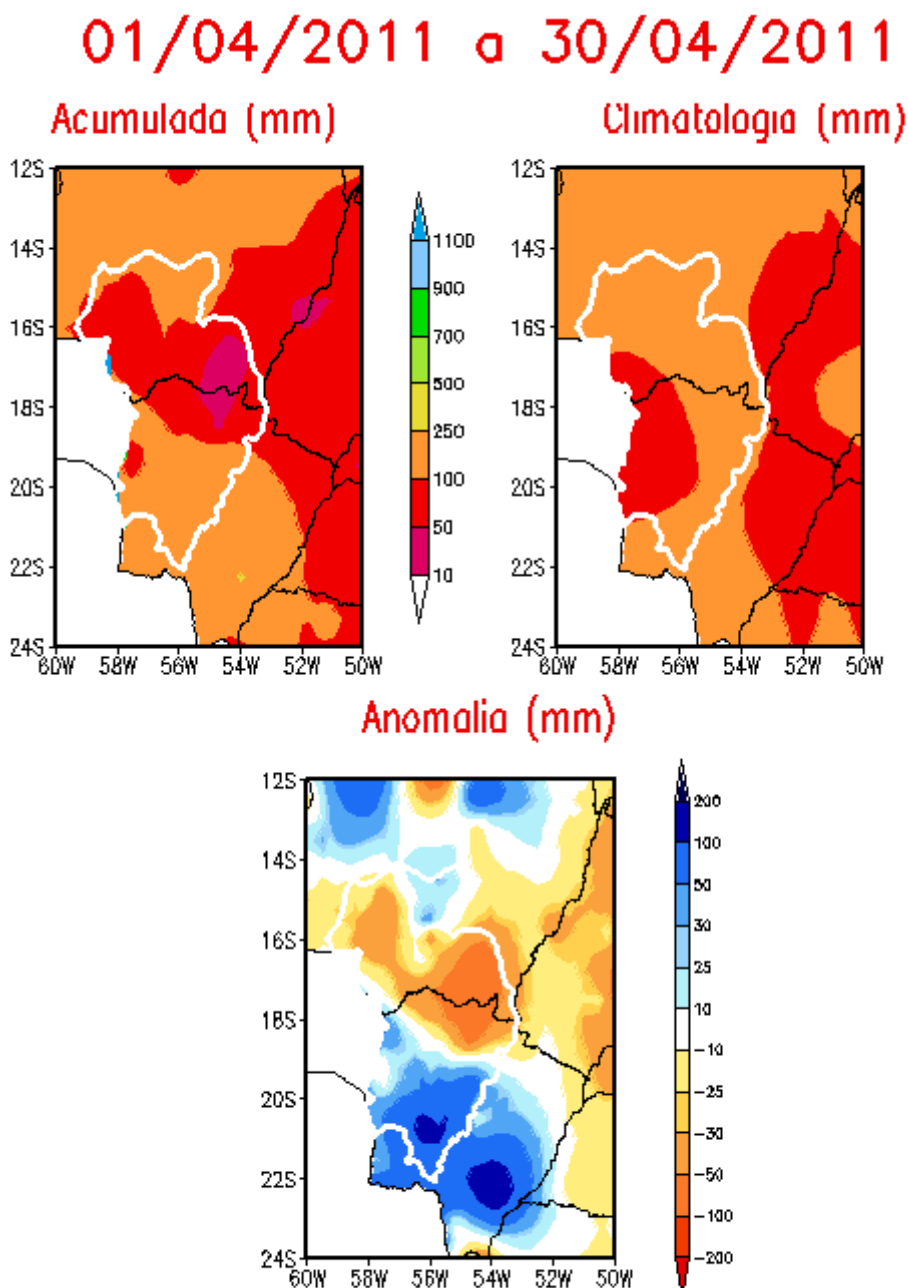
Figura 15 – Precipitação mensal acumulada, média climatológica e anomalia de precipitação na BAP, no período de 01/04/11 a 30/04/11.
