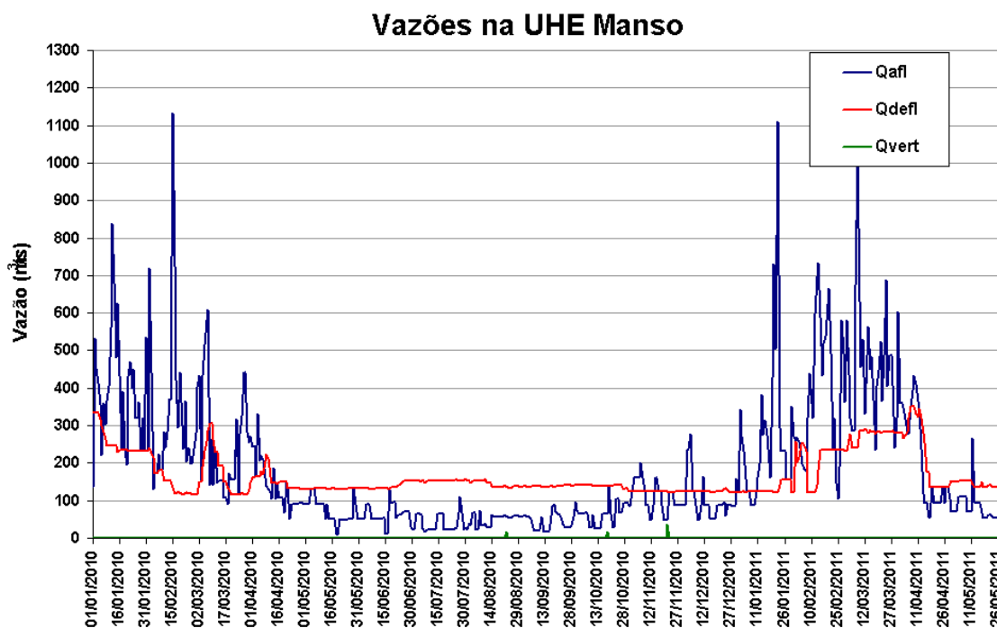
Figura 11 – Vazões na UHE Manso de janeiro de 2010 a maio de 2011.
