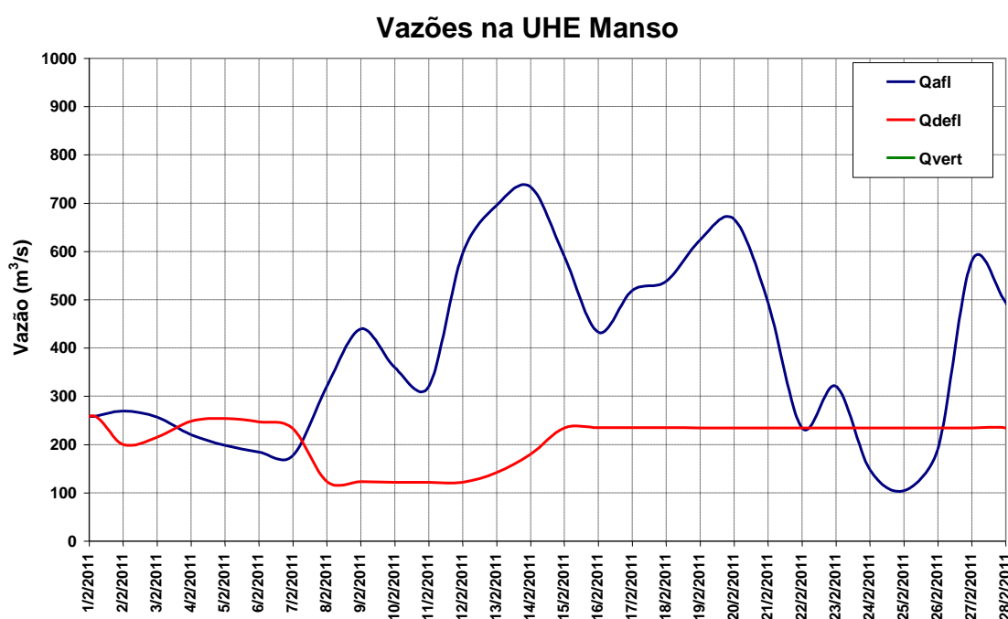
Figura 12 – Vazões na UHE Manso para o mês de fevereiro de 2011.
