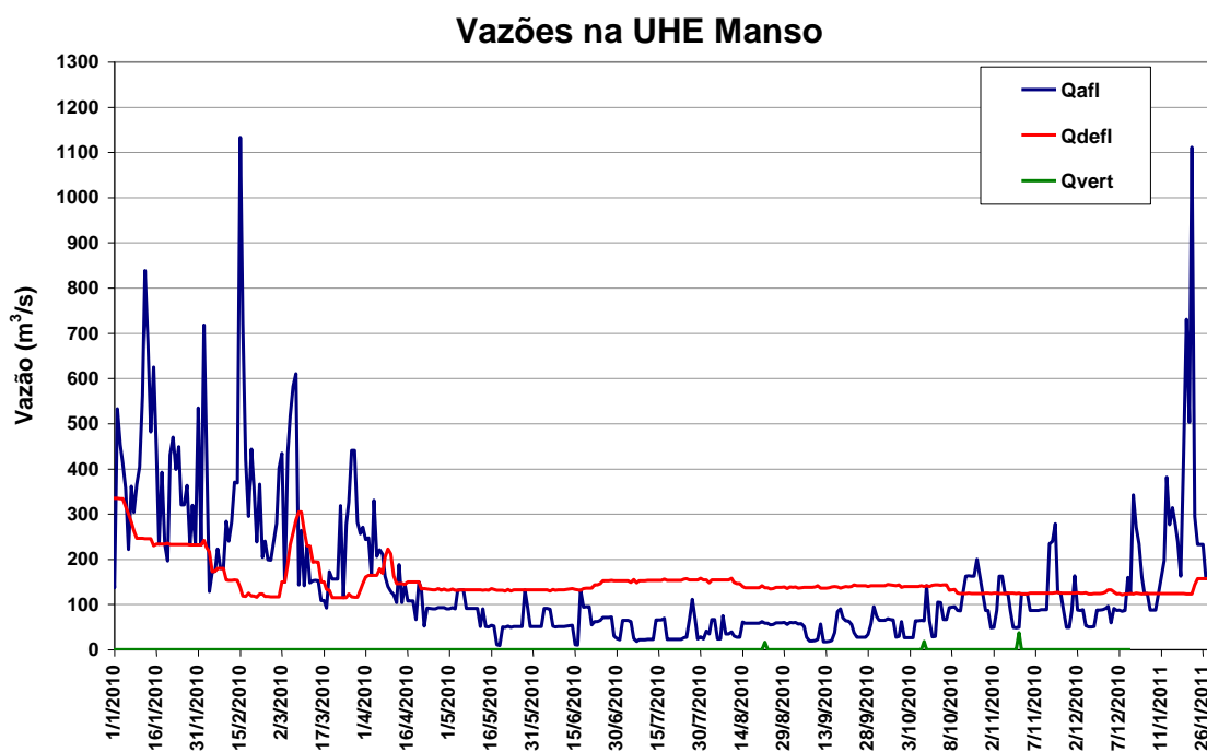
Figura 11 – Vazões na UHE Manso de janeiro de 2010 a fevereiro de 2011.
