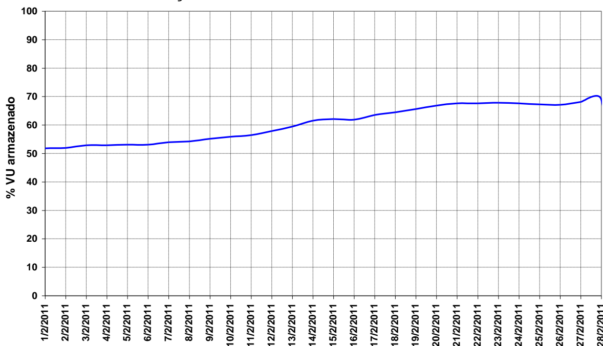
Figura 14 – Volume Útil na UHE Manso para o mês de fevereiro de 2011.
