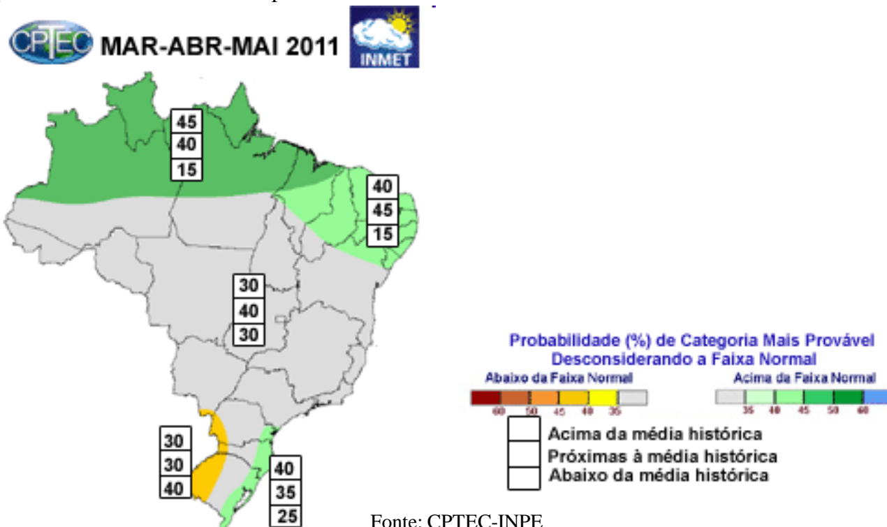
Figura 20 – Previsão climática para o trimestre mar / abr / mai de 2011.
