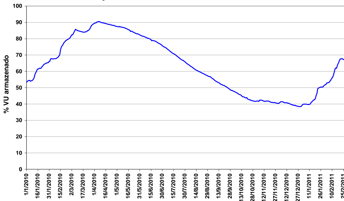
Figura 13 – Volume Útil na UHE Manso de janeiro de 2010 a fevereiro de 2011.
