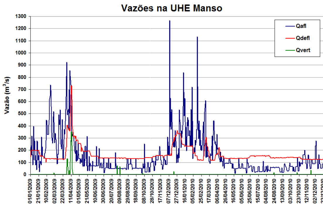
Figura 11 – Vazões na UHE Manso de janeiro de 2009 a dezembro de 2010.
