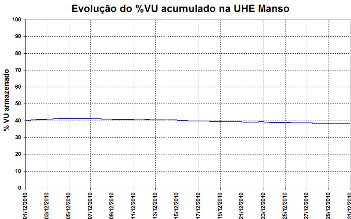
Figura 14 – Volume Útil na UHE Manso para o mês de dezembro de 2010.
