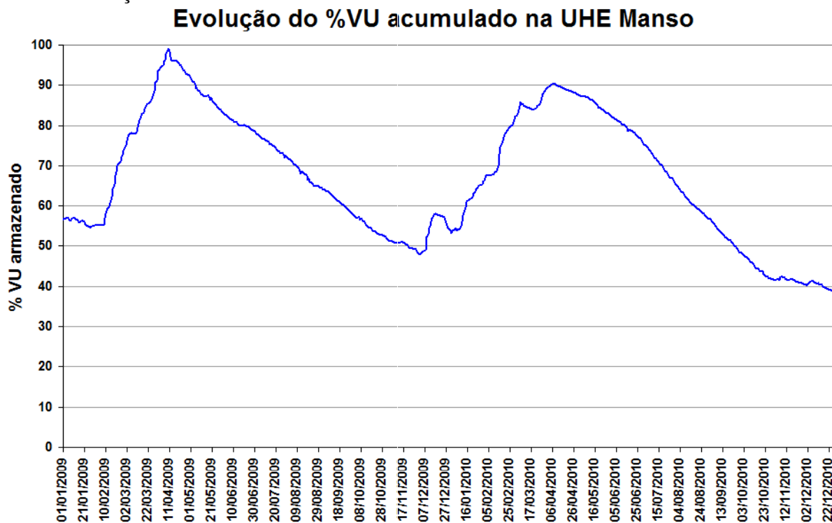
Figura 13 – Volume Útil na UHE Manso de janeiro de 2009 a dezembro de 2010.
