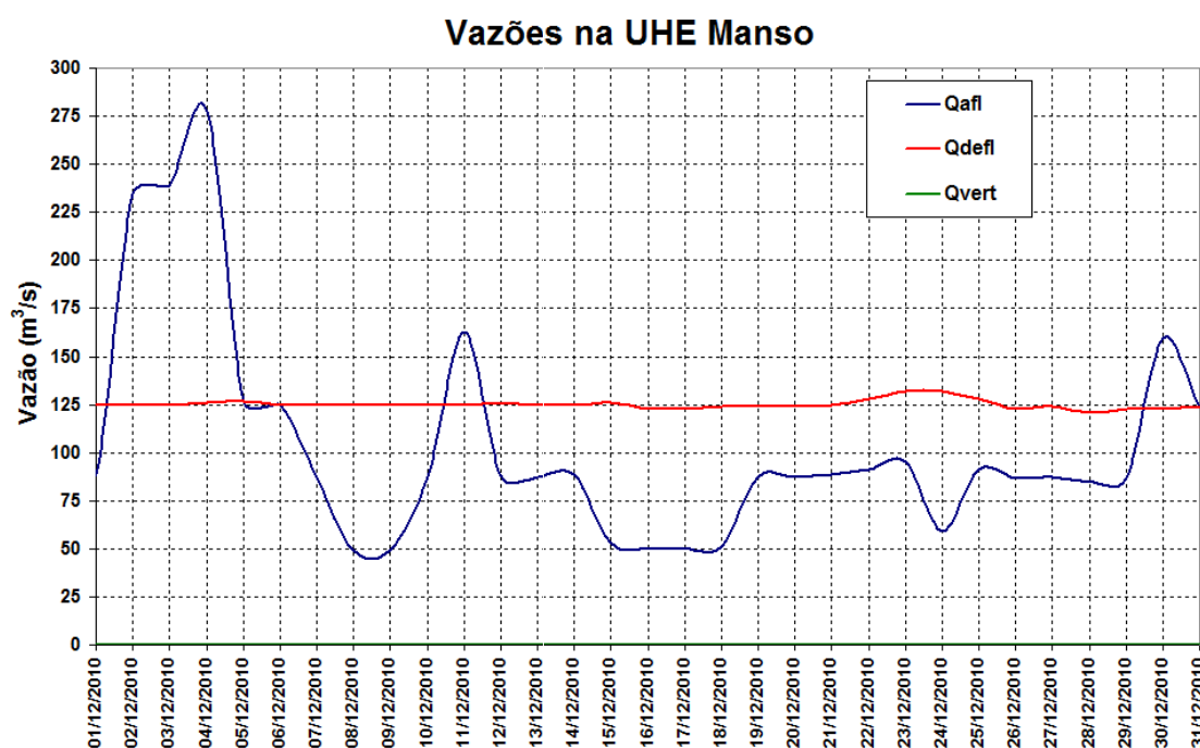
Figura 12 – Vazões na UHE Manso para o mês de dezembro de 2010.
