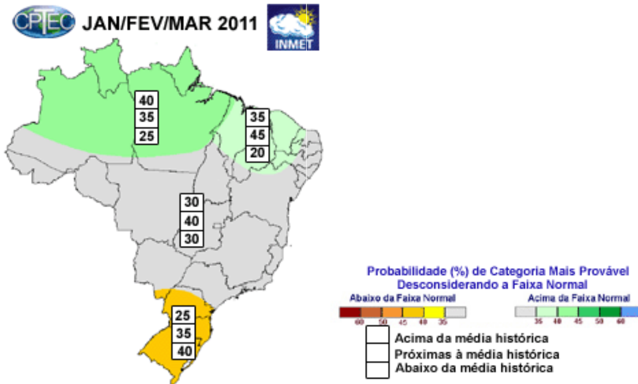
Figura 18 – Previsão climática para o trimestre jan / fev / mar de 2011.
