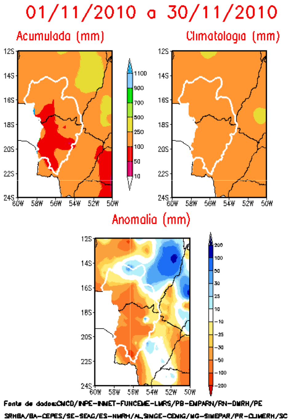
Figura 15 – Precipitação mensal acumulada, média climatológica e anomalia de precipitação na BAP, no período de 01/11/10 a 30/11/10.
