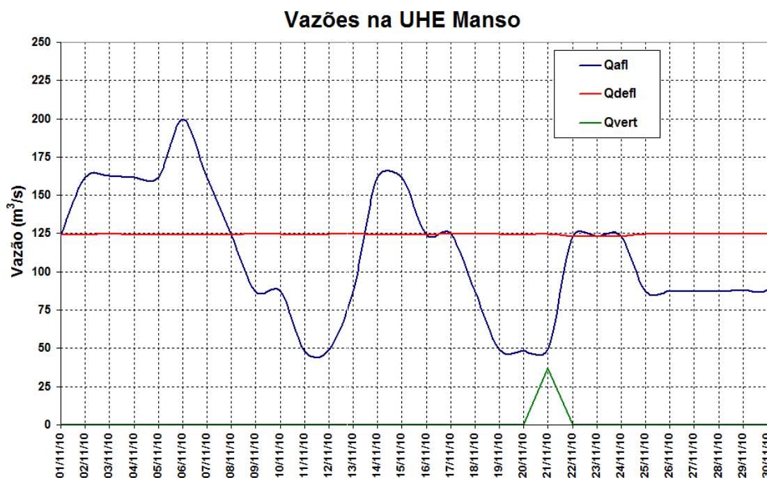
Figura 12 – Vazões na UHE Manso para o mês de novembro de 2010.
