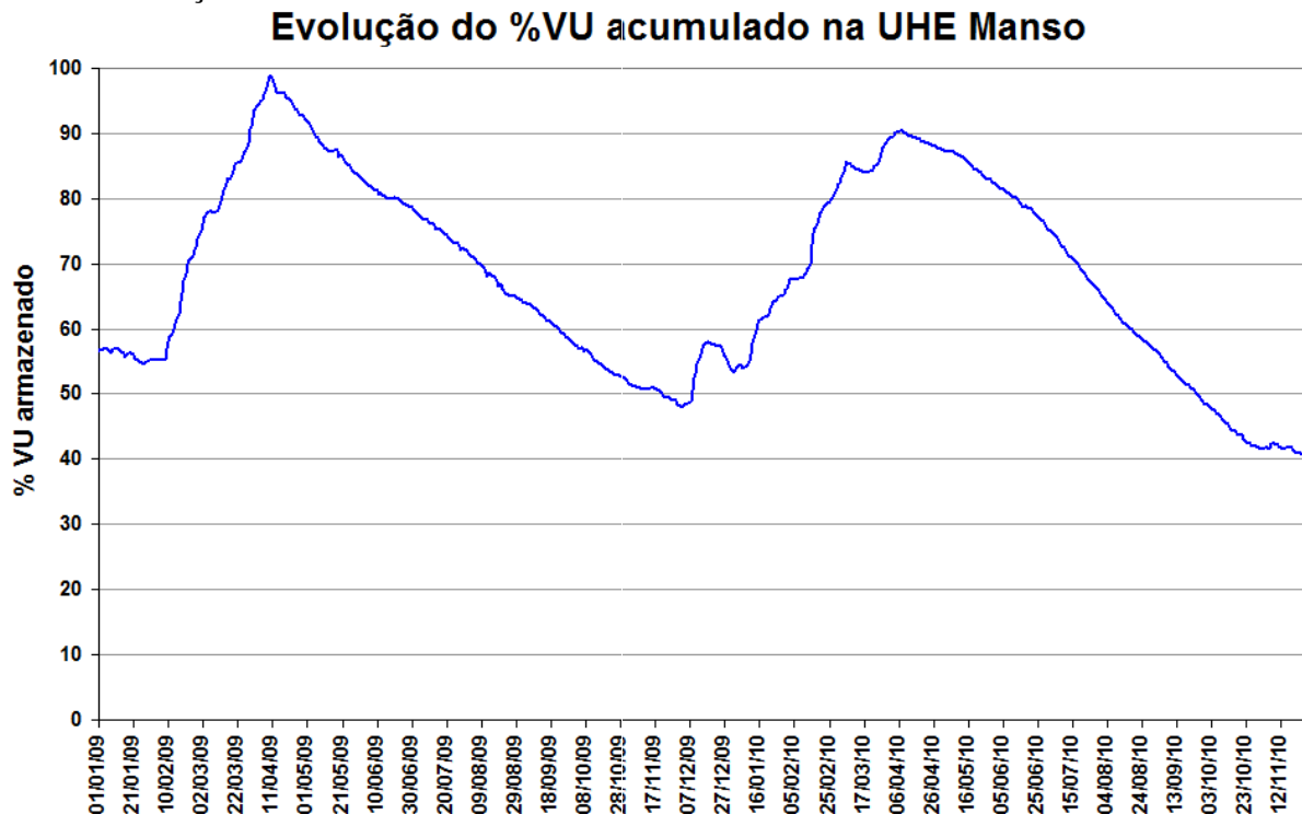
Figura 13 – Volume Útil na UHE Manso de janeiro de 2009 a novembro de 2010.
