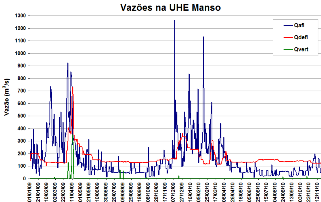
Figura 11 – Vazões na UHE Manso de janeiro de 2009 a novembro de 2010.
