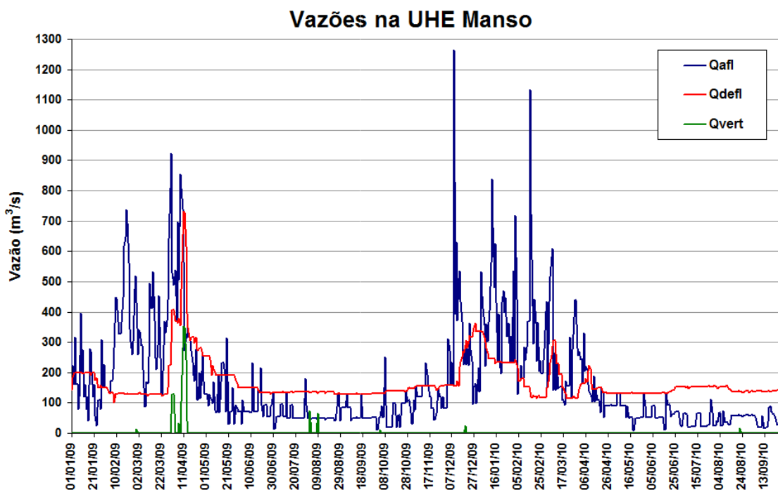
Figura 11 – Vazões na UHE Manso de janeiro de 2009 a setembro de 2010.
