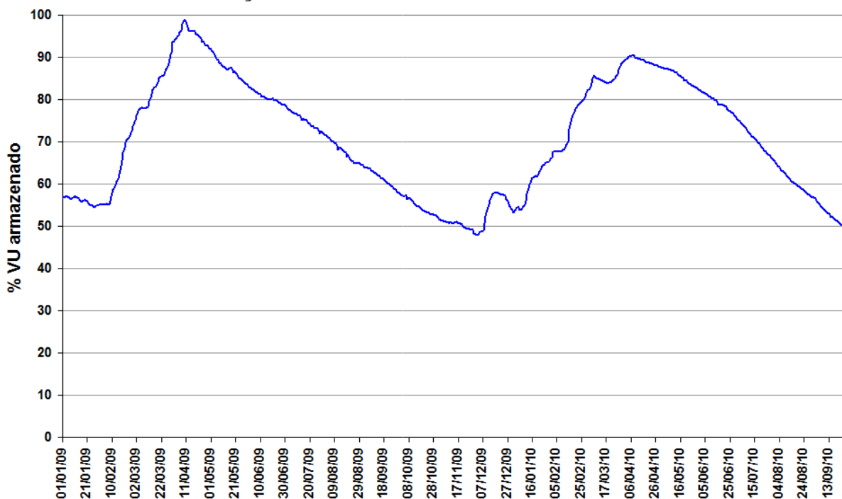
Figura 13 – Volume Útil na UHE Manso de janeiro de 2009 a setembro de 2010.
