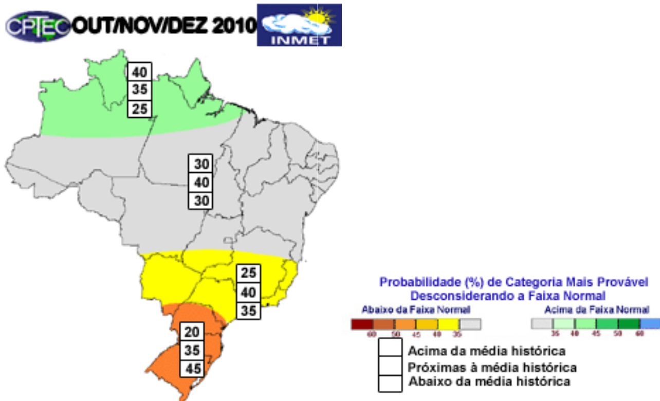
Figura 18 – Previsão climática para o trimestre out / nov / dez de 2010.
