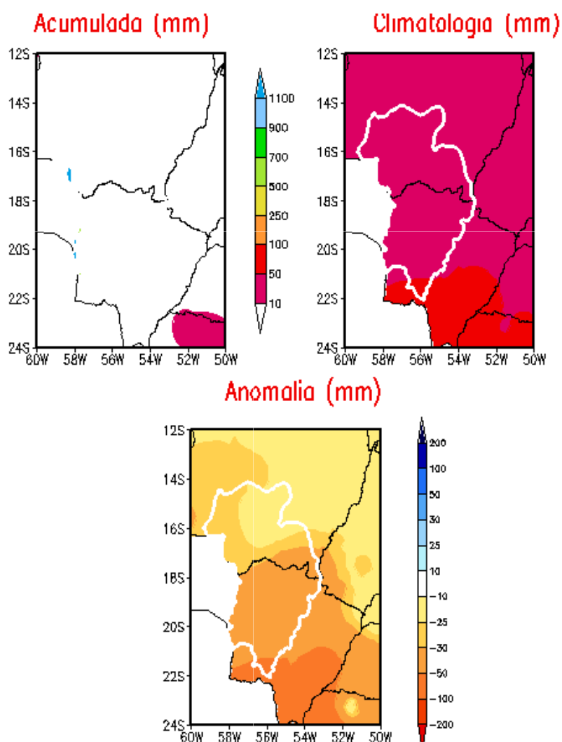
Figura 15 - Isoietas de precipitação acumulada, climatologia e de anomalias de precipitação na BAP, no período de 01/08/10 a 31/08/10.
