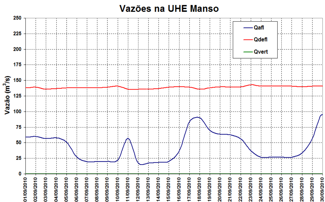
Figura 12 – Vazões na UHE Manso para o mês de setembro de 2010.
