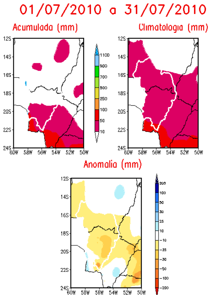
Figura 15 - Isoietas de precipitação acumulada, climatologia e de anomalias de precipitação na BAP, no período de 01/07/10 a 31/07/10.
