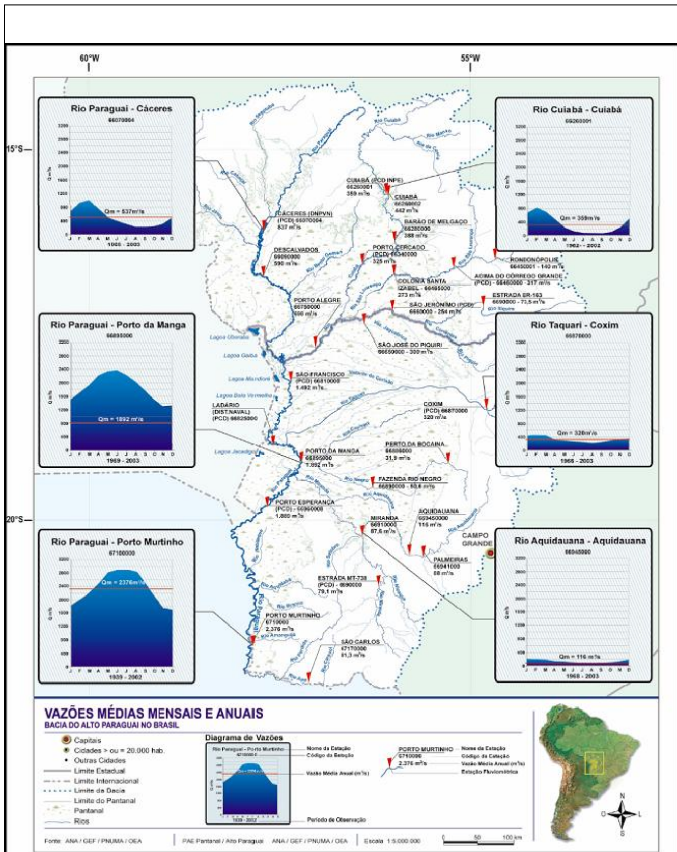
Figura 2 – Vazões médias mensais e anuais em algumas estações da bacia
