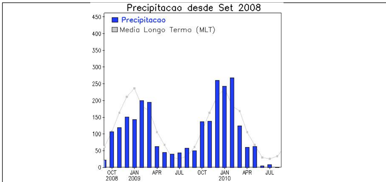
Figura 17 – Evolução da Precipitação na Bacia do Alto Paraguai.
