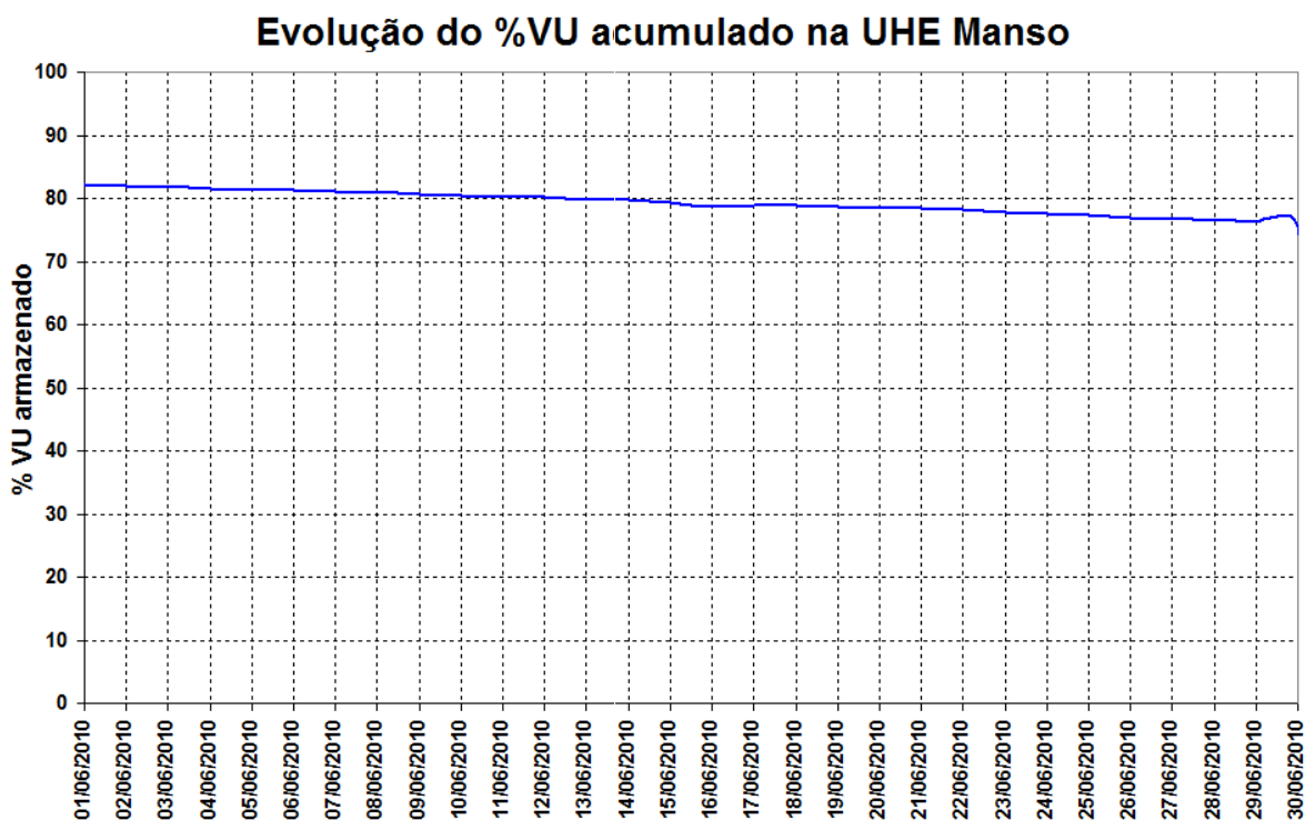
Figura 14 – Volume Util na UHE Manso para o mês de junho de 2010.
