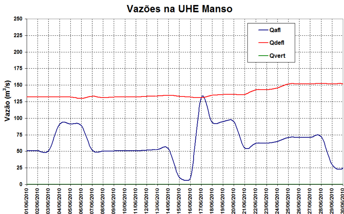
Figura 12 – Vazões na UHE Manso para o mês de junho de 2010.
