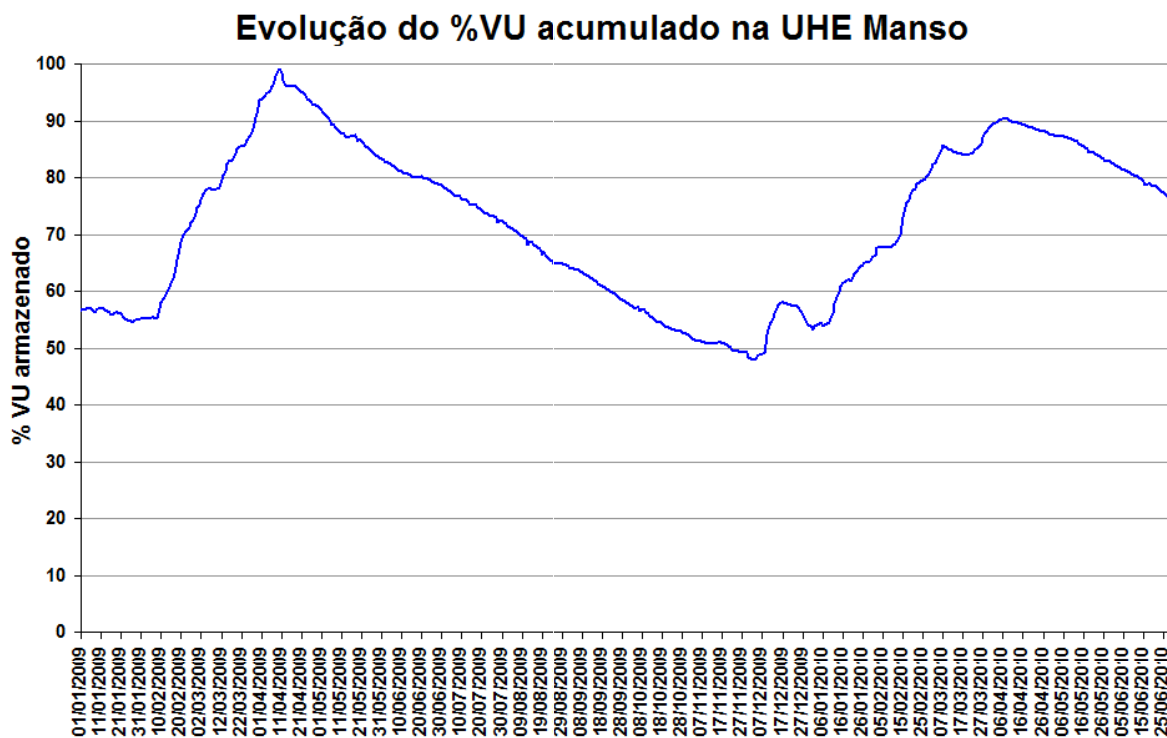
Figura 13 – Volume Util na UHE Manso de janeiro de 2009 a junho de 2010.
