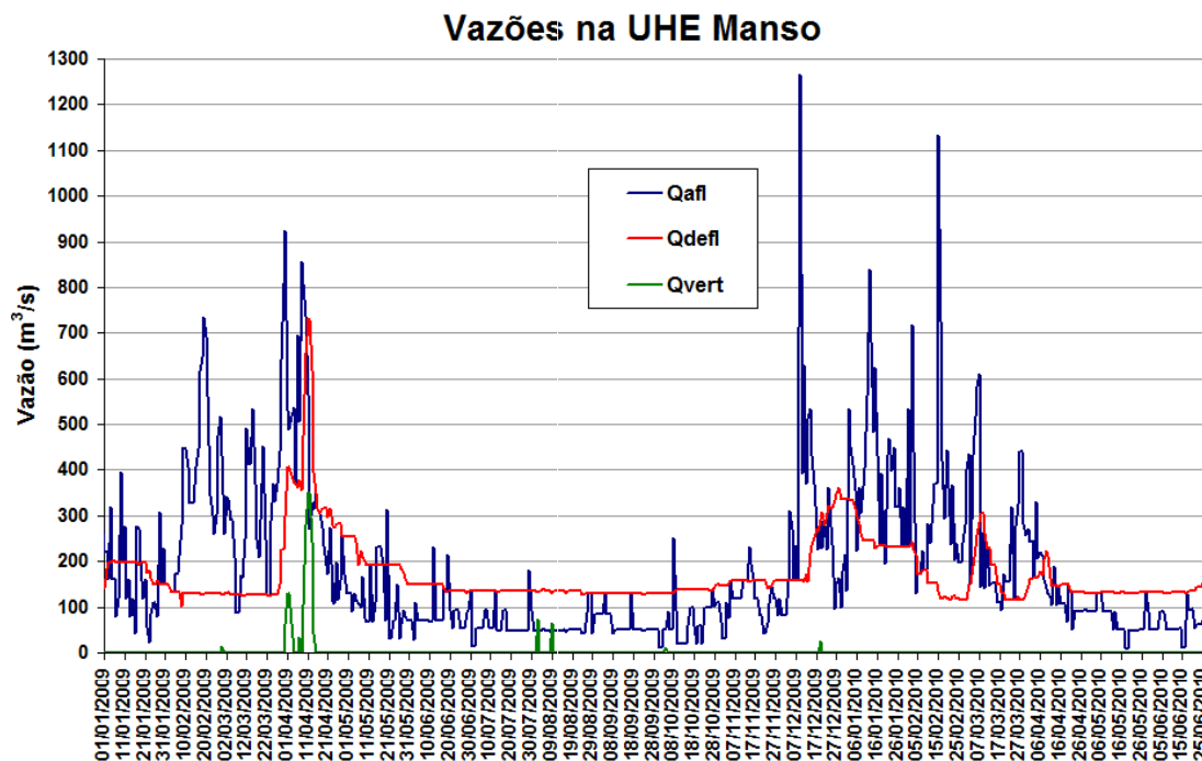
Figura 11 – Vazões na UHE Manso de janeiro de 2009 a junho de 2010.
