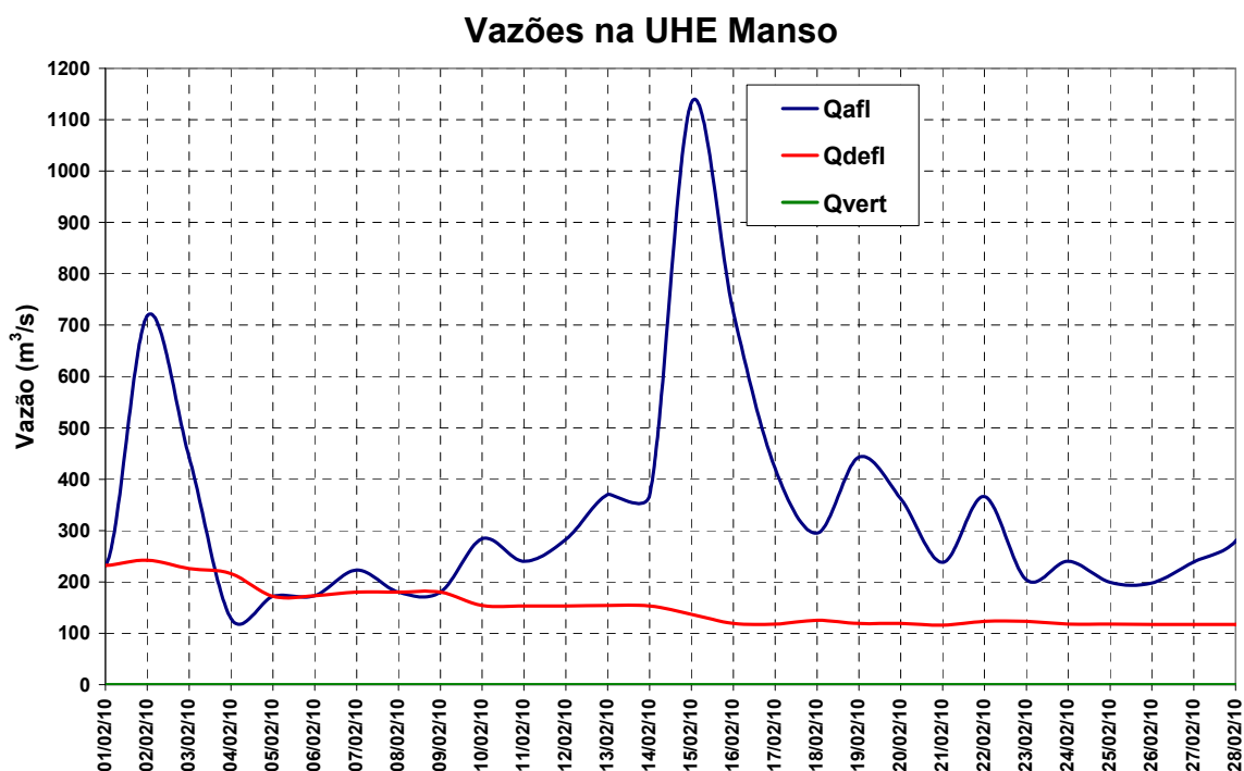
Figura 12 – Vazões na UHE Manso para o mês de fevereiro de 2010
