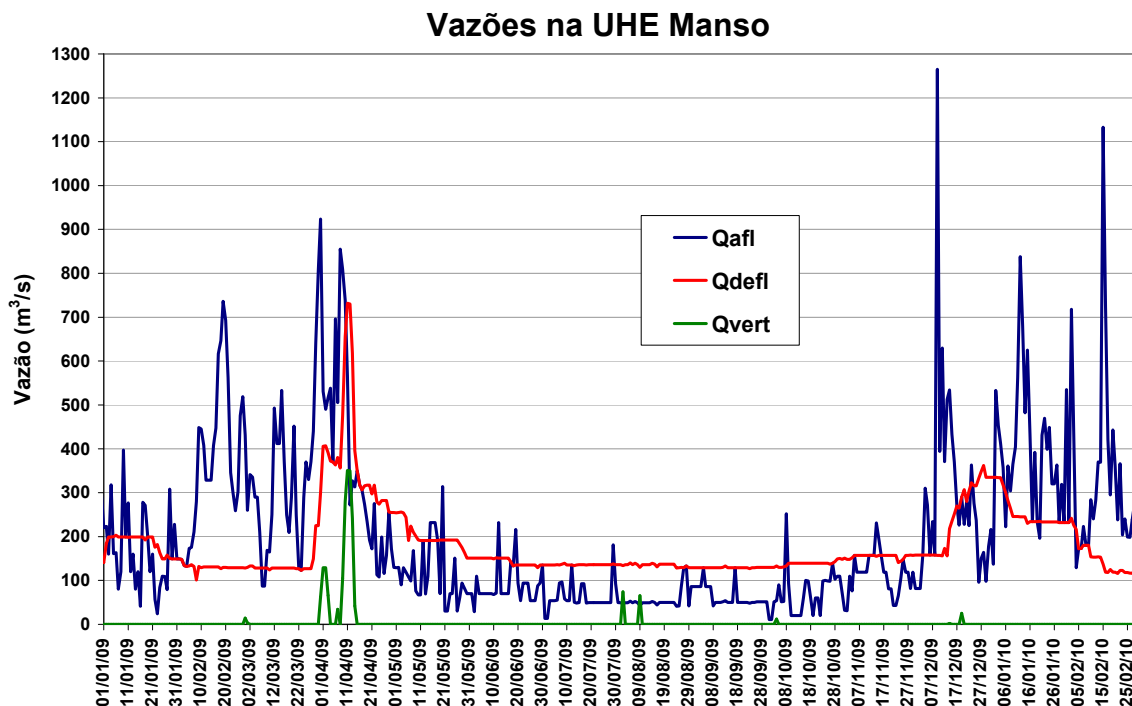
Figura 11 – Vazões na UHE Manso de janeiro de 2009 a fevereiro de 2010
