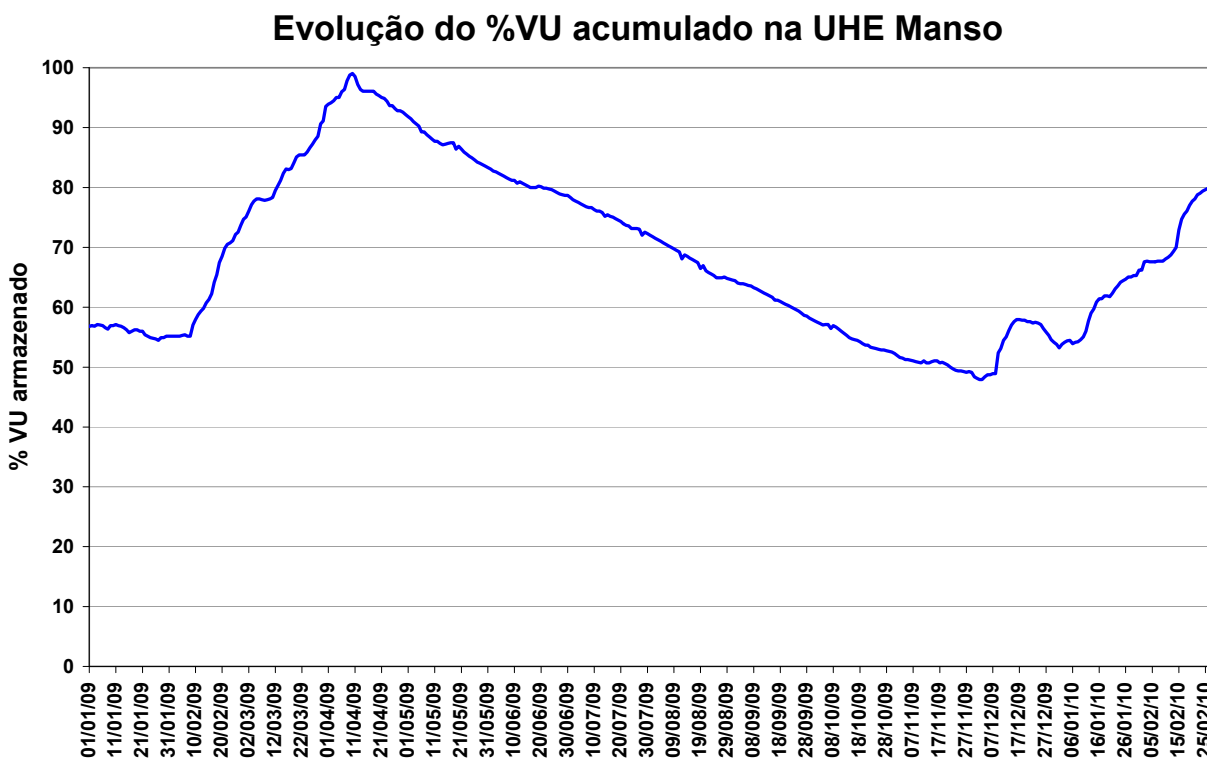
Figura 13 – Volume Útil na UHE Manso de janeiro de 2009 a fevereiro de 2010
