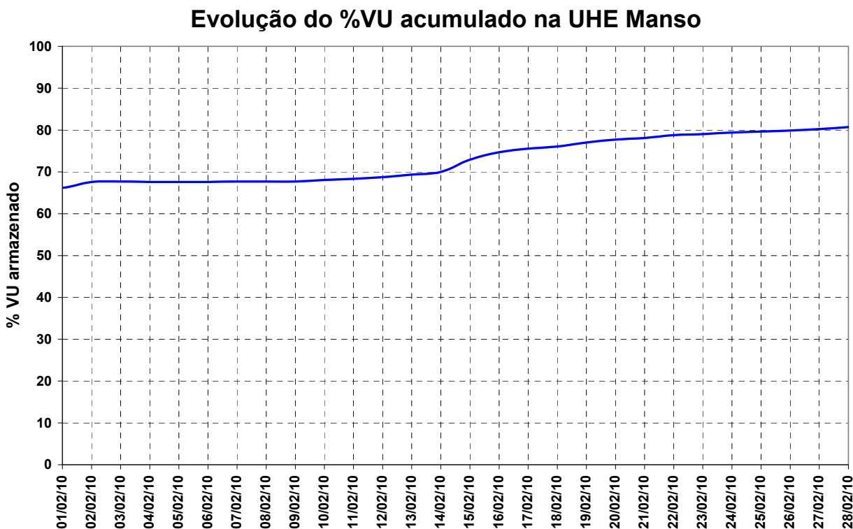
Figura 14 – Volume Útil na UHE Manso para o mês de fevereiro de 2010
