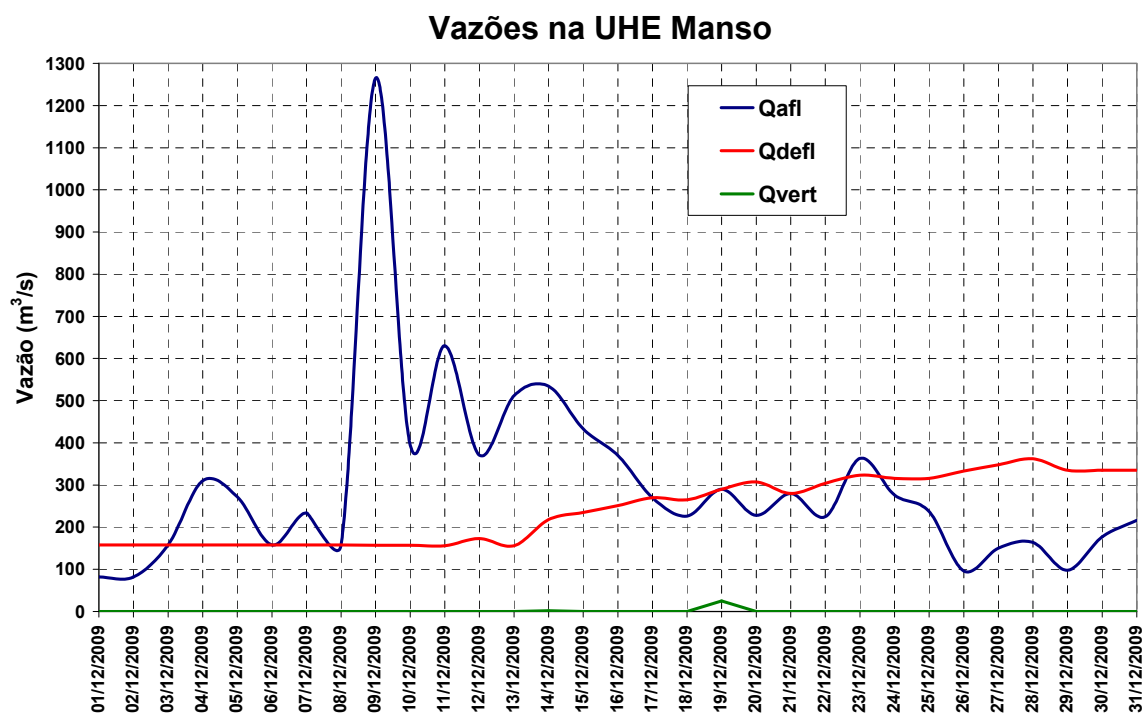
Figura 12 – Vazões na UHE Manso para o mês de dezembro de 2009
