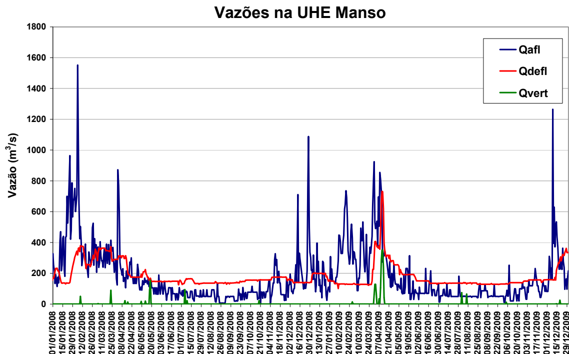
Figura 11 – Vazões na UHE Manso de janeiro de 2008 a dezembro de 2009
