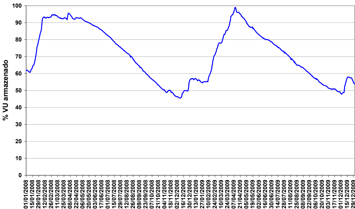
Figura 13 – Volume Útil na UHE Manso de janeiro de 2008 a dezembro de 2009
