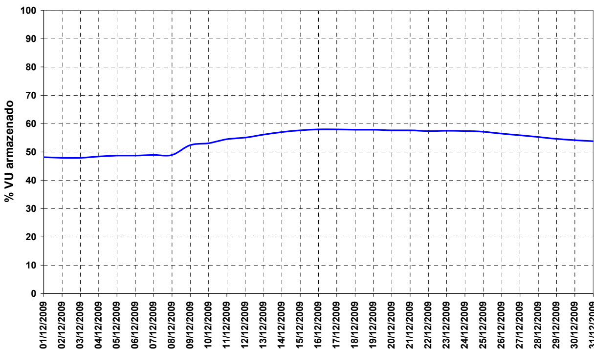
Figura 14 – Volume Útil na UHE Manso para o mês de dezembro de 2009
