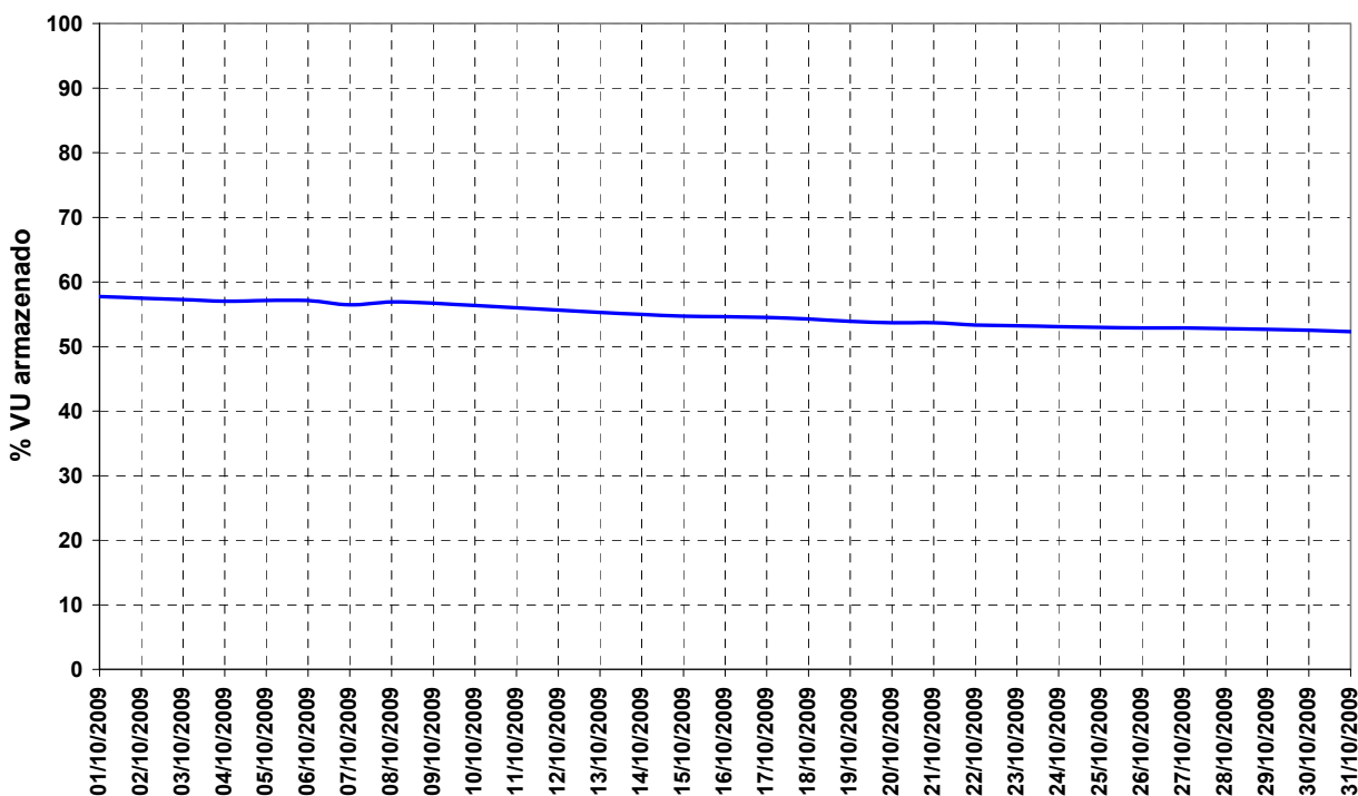
Figura 14 – Volume Útil na UHE Manso para o mês de outubro de 2009
