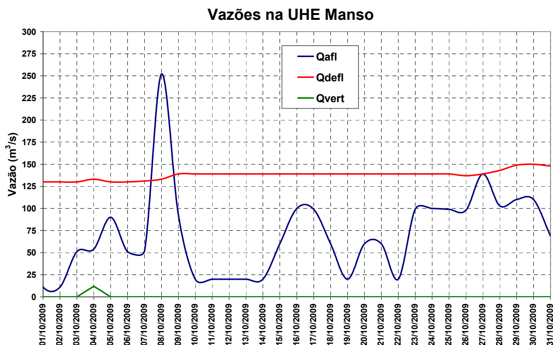
Figura 12 – Vazões na UHE Manso para o mês de outubro de 2009
