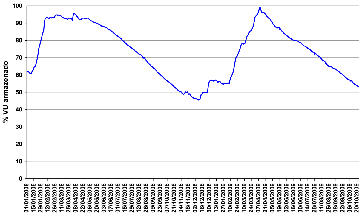
Figura 13 – Volume Útil na UHE Manso de janeiro de 2008 a outubro de 2009
