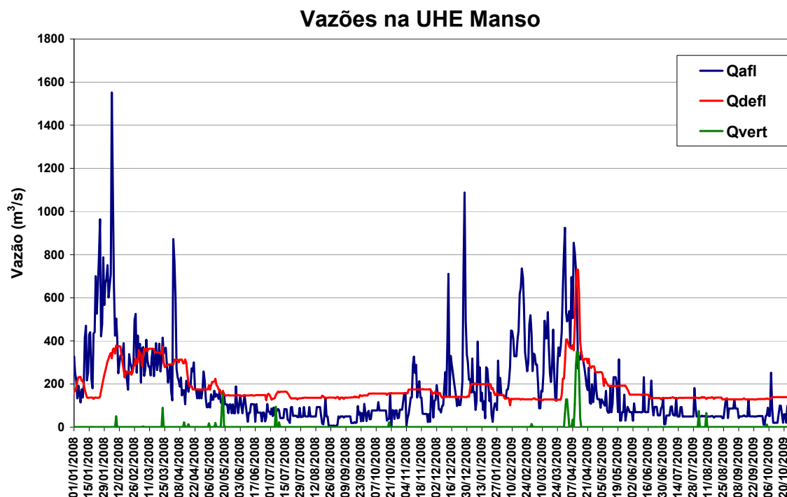
Figura 11 – Vazões na UHE Manso de janeiro de 2008 a outubro de 2009
