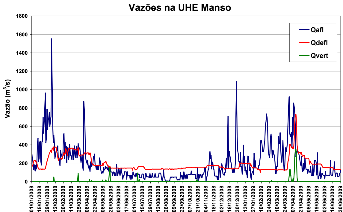
Figura 11 – Vazões na UHE Manso de janeiro de 2008 a junho de 2009
