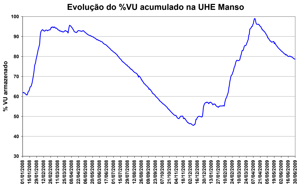
Figura 13 – Volume Útil na UHE Manso de janeiro de 2008 a junho de 2009
