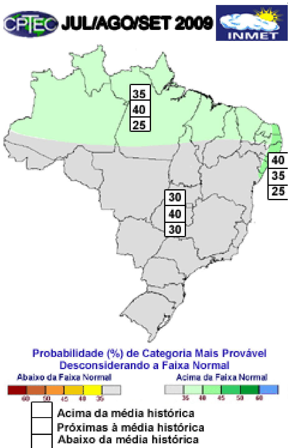
Figura 17 – Previsão climática para o trimestre jul / ago / set.
