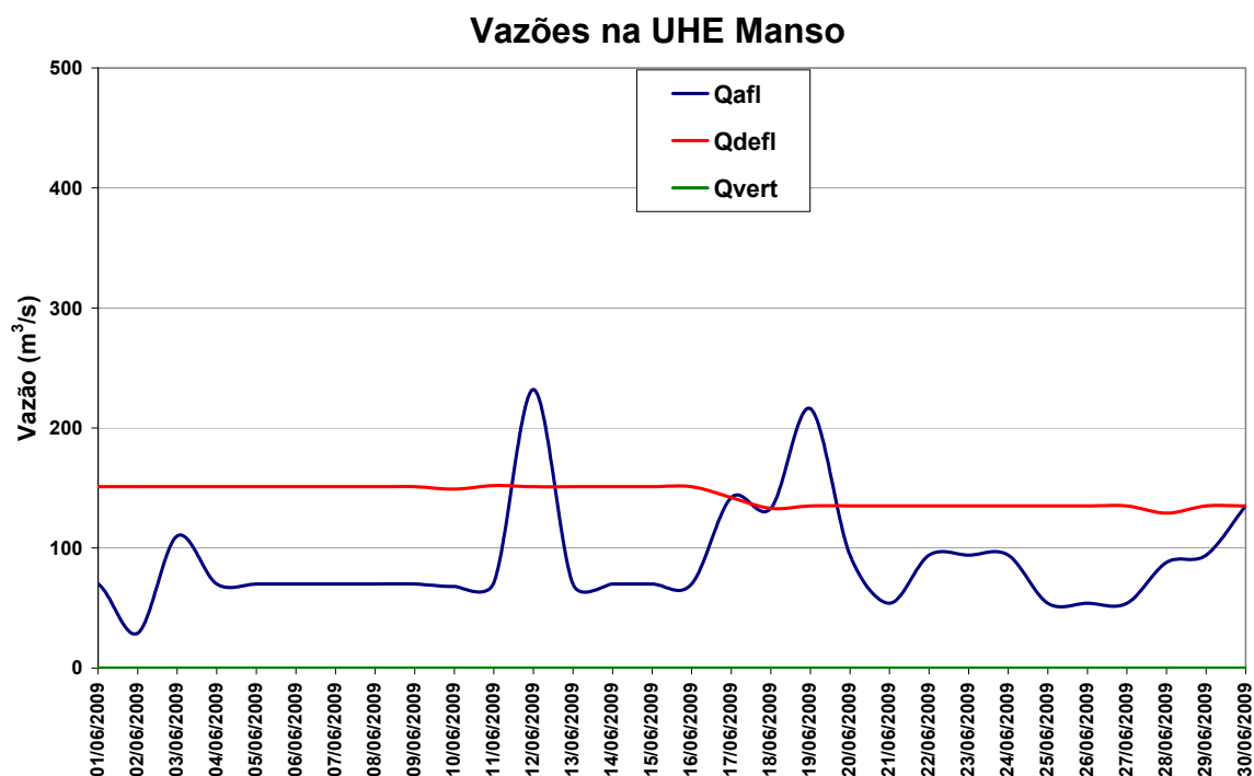
Figura 12 – Vazões na UHE Manso para o mês de junho de 2009
