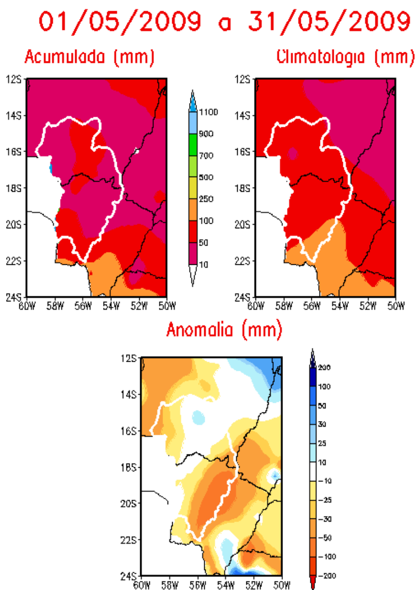
Figura 15 - Isoietas de precipitação acumulada, climatologia e de anomalias de precipitação na BAP, no período de 01/05/09 a 31/05/09.
