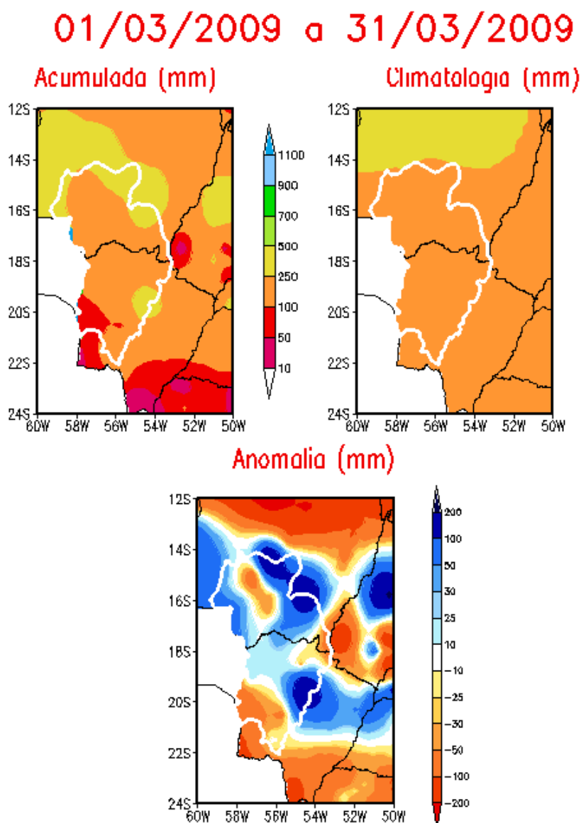
Figura 15 - Isoietas de precipitação acumulada, climatologia e de anomalias de precipitação na BAP, no período de 01/03/09 a 31/03/09.
