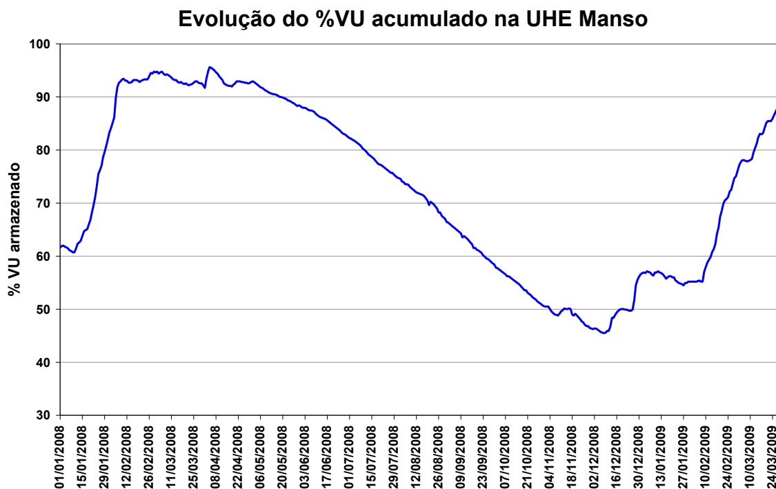
Figura 13 – Volume Útil na UHE Manso de janeiro de 2008 a março de 2009
