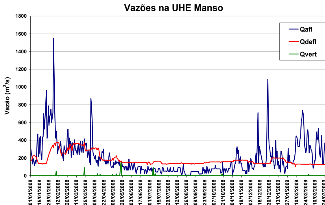
Figura 11 – Vazões na UHE Manso de janeiro de 2008 a março de 2009
