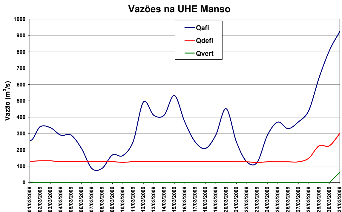
Figura 12 – Vazões na UHE Manso para o mês de março de 2009
