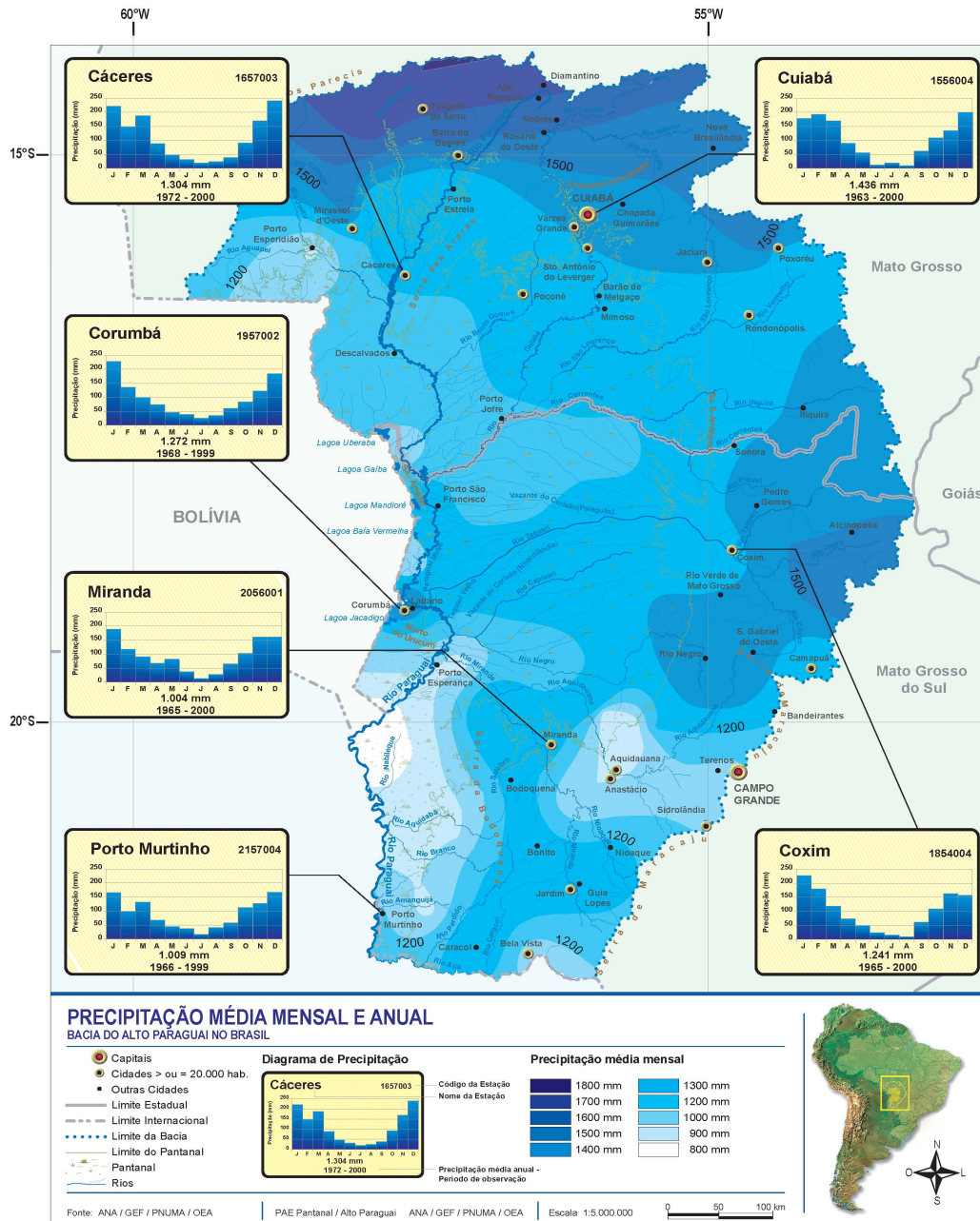
Figura 1 - Precipitação Média
