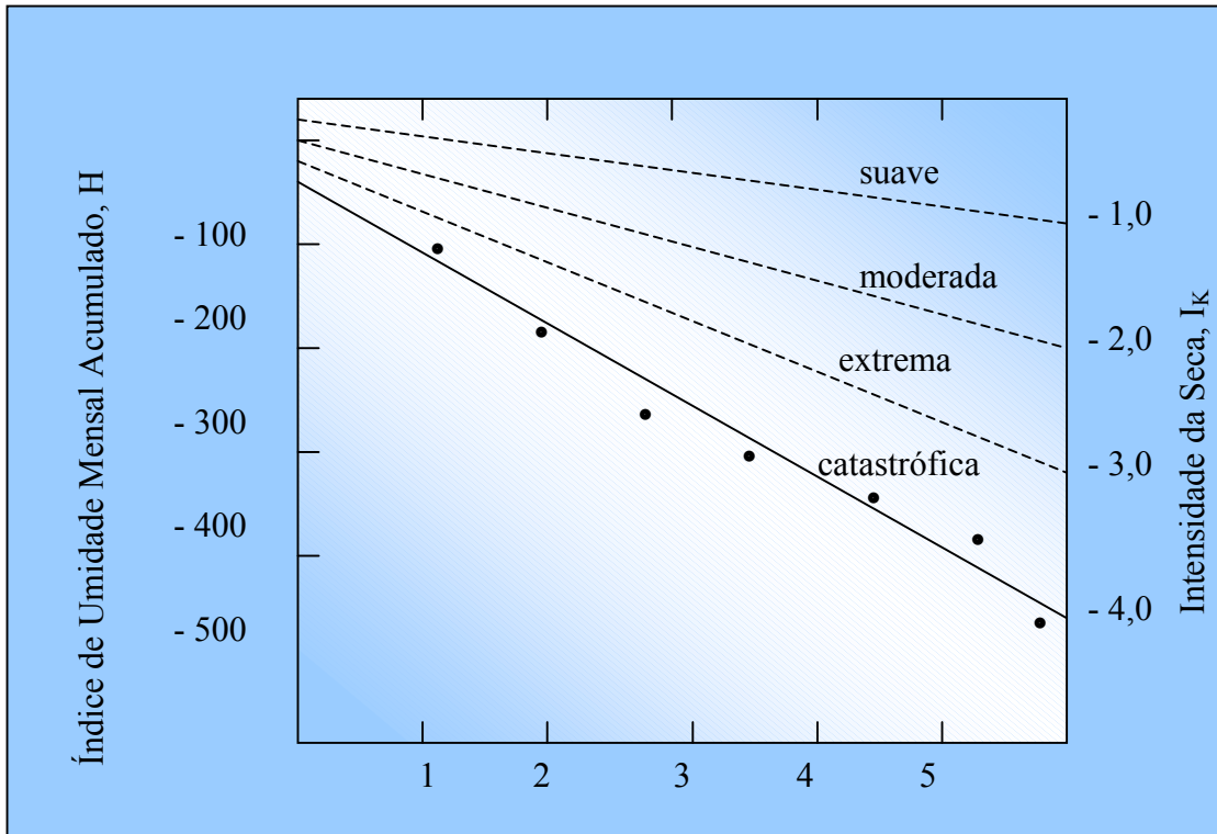
Figura 4: Valores de BMDI para o Estado do Ceará
