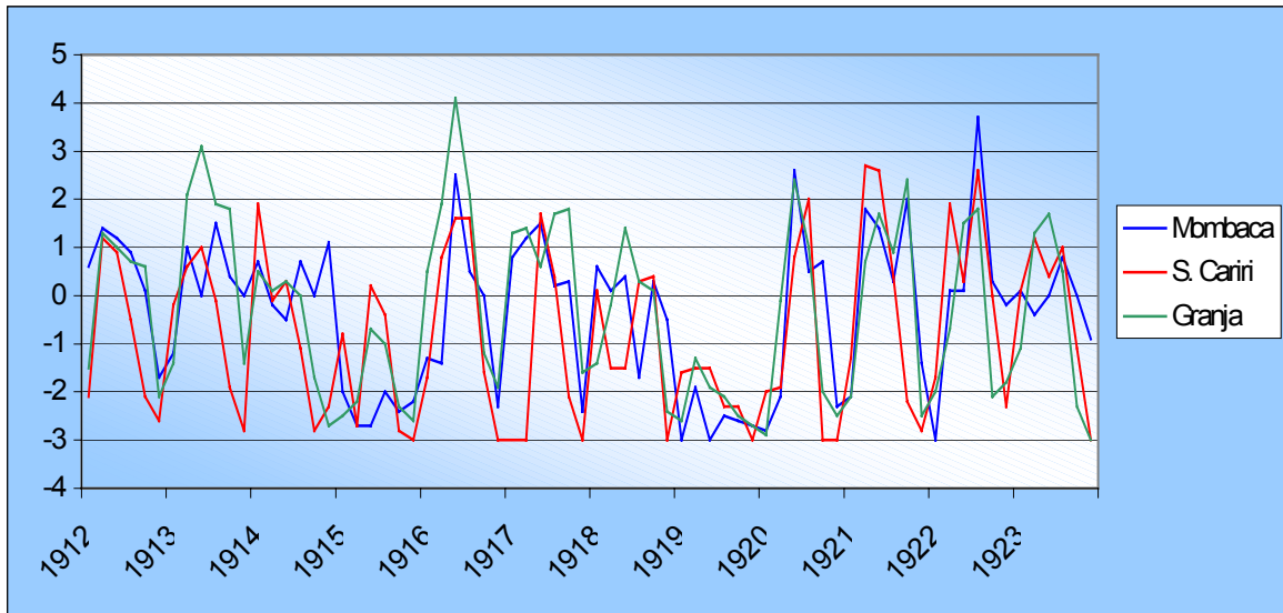
Figura 2: Rainfall Anomaly Index (RAI) para três postos pluviométricos do Estado do Ceará.
